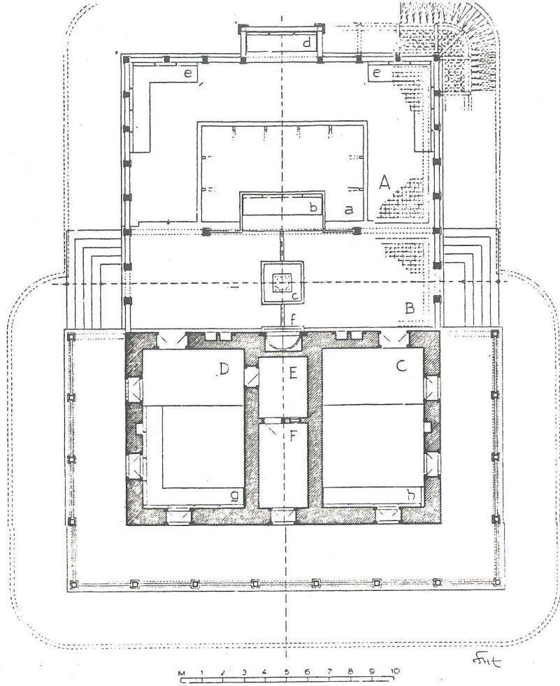
Şekil 8. Fener köşkü restitüsyon planı.
