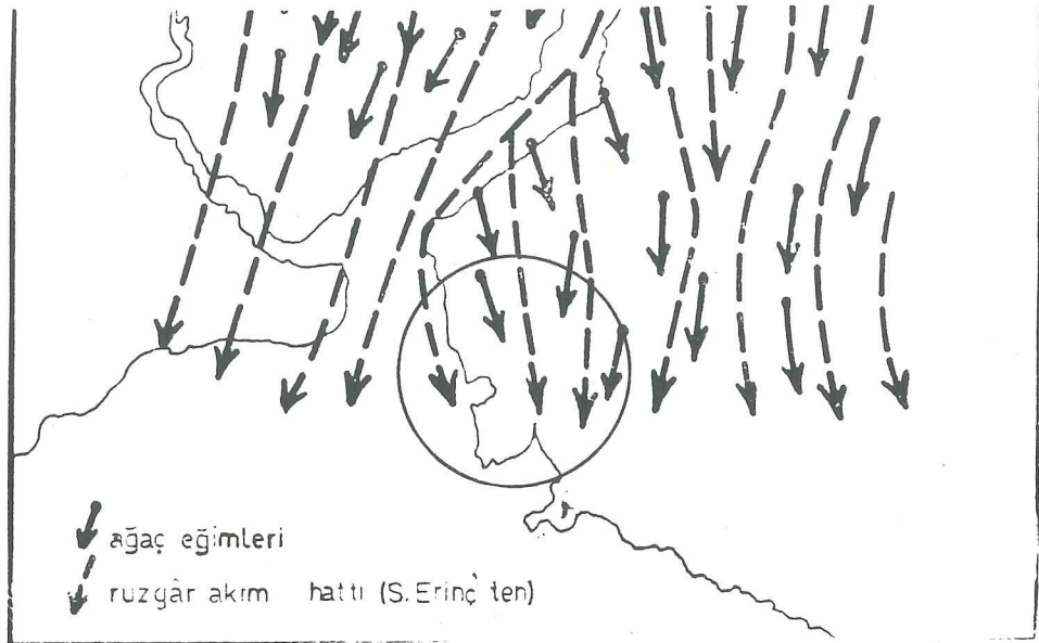
Şekil 2. Rüzgâr Akım Hattı
