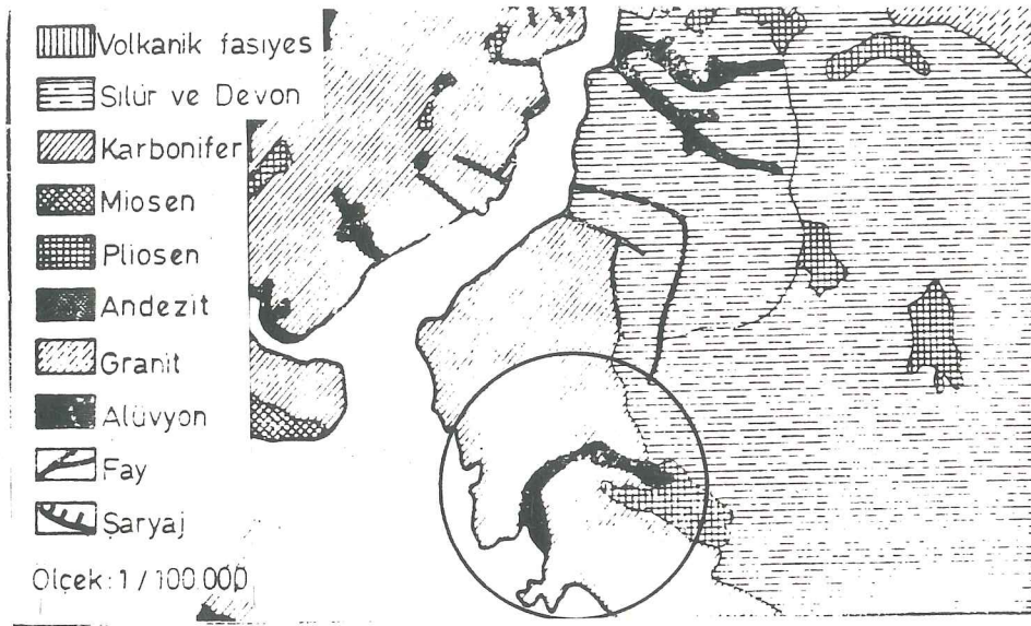
Şekil 1: Kurbagalidere Jeolojik Yapısı
