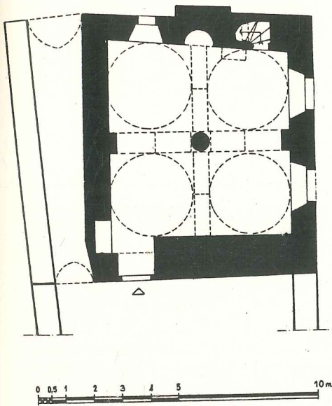
P.4- Taş Cami
