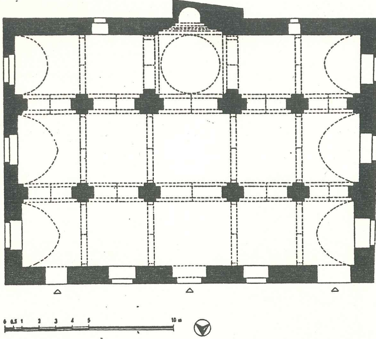
P.1- Bitlis Ulu Camii Plânı
