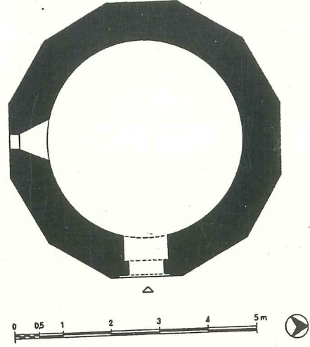
P.8- Şeyh Tahiri Gürği Türbesi Plânı
