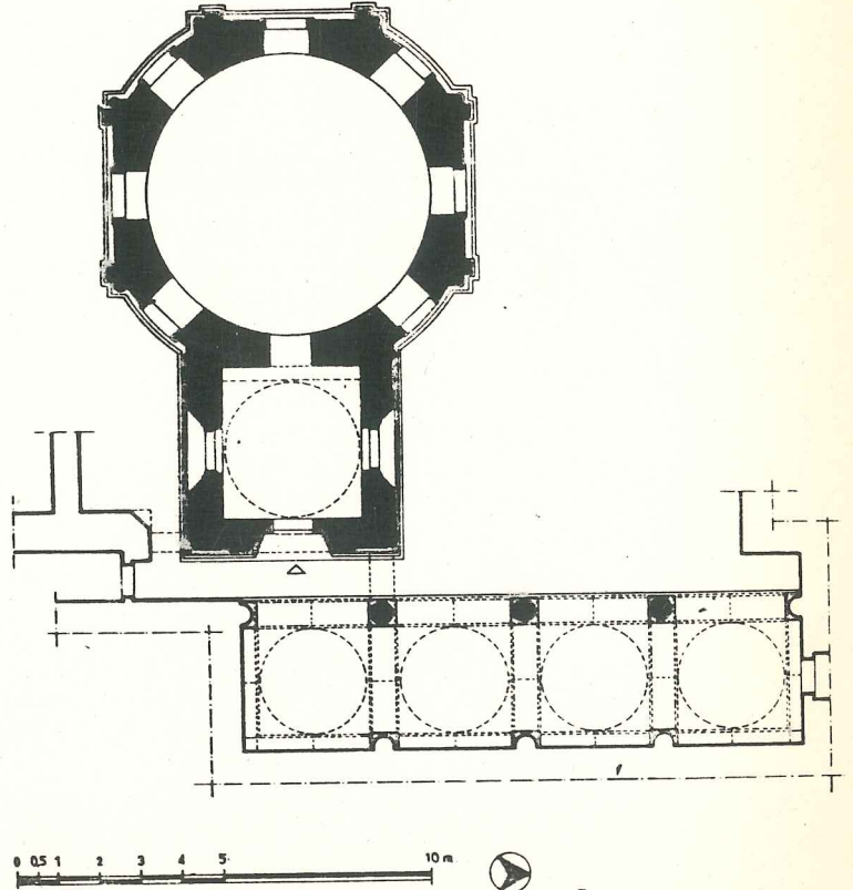
P.10- Küfrevi Türbe ve Dergâhı Plânı
