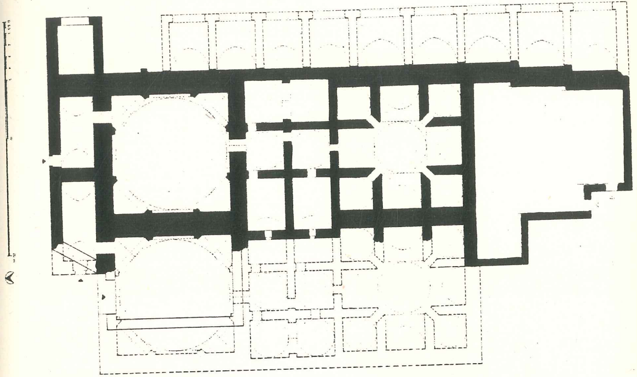
P.15- Hüsrev Paşa Hamamı Planı
