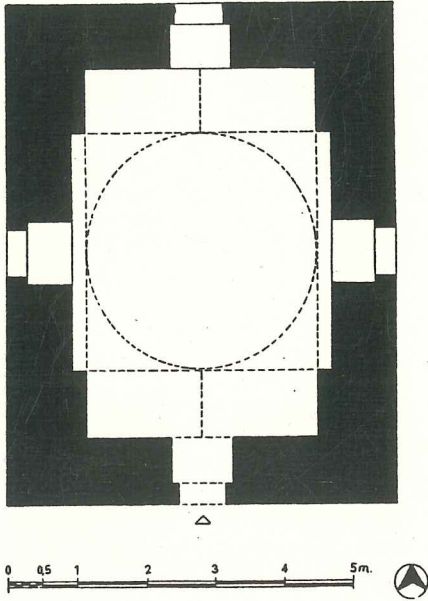
P.9- Nuhiye Türbesi Plânı
