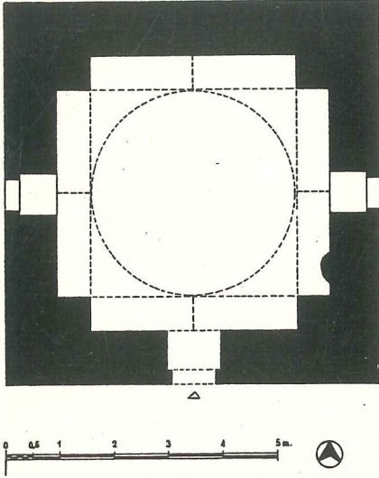
P.7- Şeyh Hacı İbrahim Türbesi Plânı
