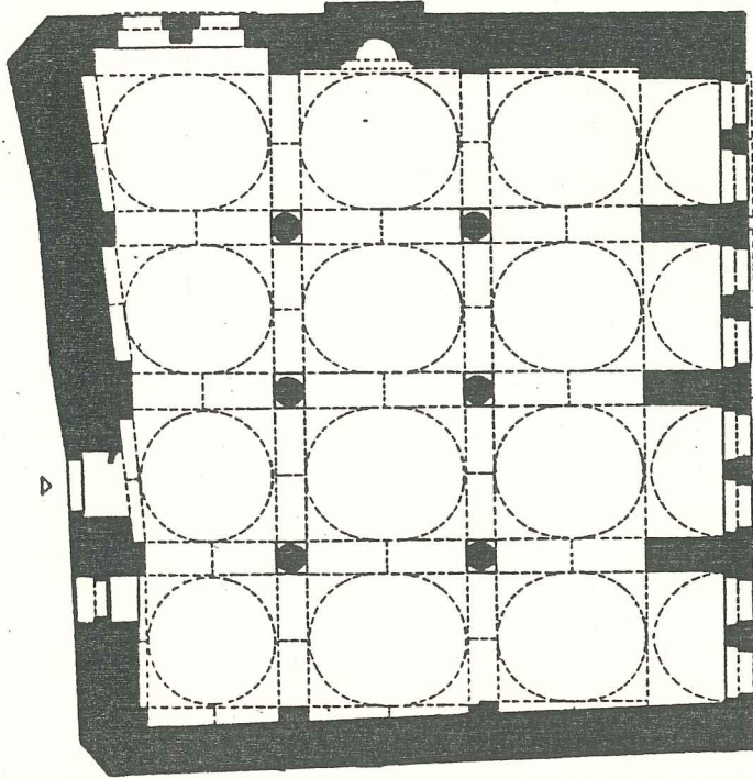
P.2- Kızıl Mescit Plânı
