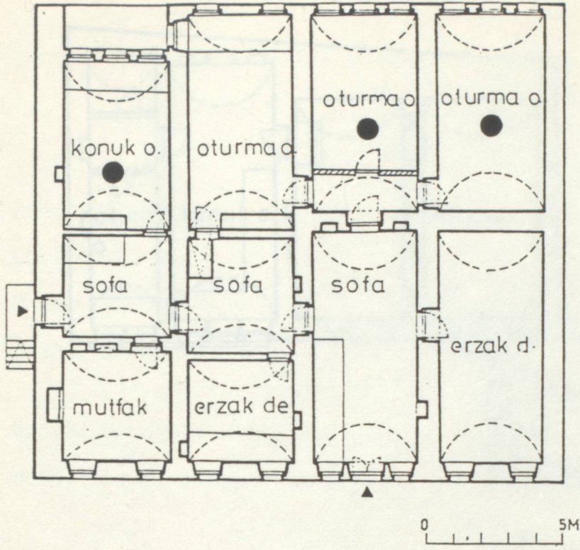
GİRİŞ KATI PLANI
