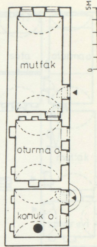
GİRİŞ KATI PLANI
