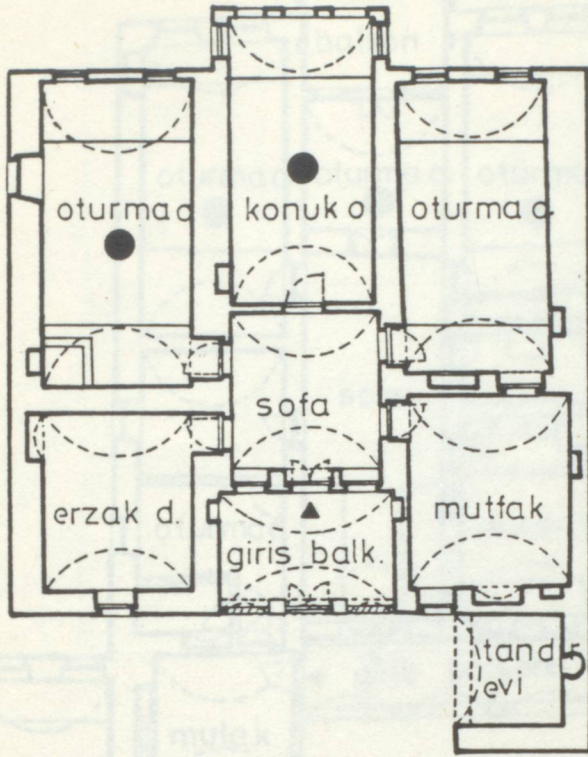
GİRİŞ KATI PLANI
