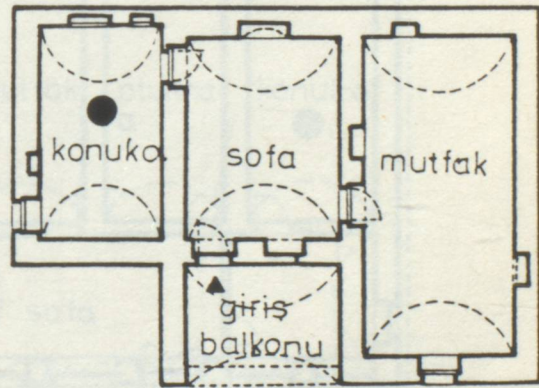
GİRİŞ KATI PLANI
