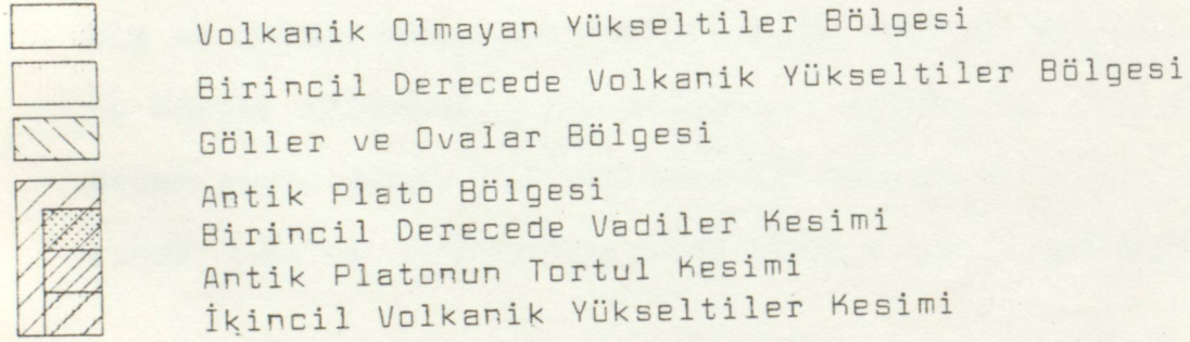
Çizim No.3: Kapadokya'nın Jeolojik Bölgeleri
