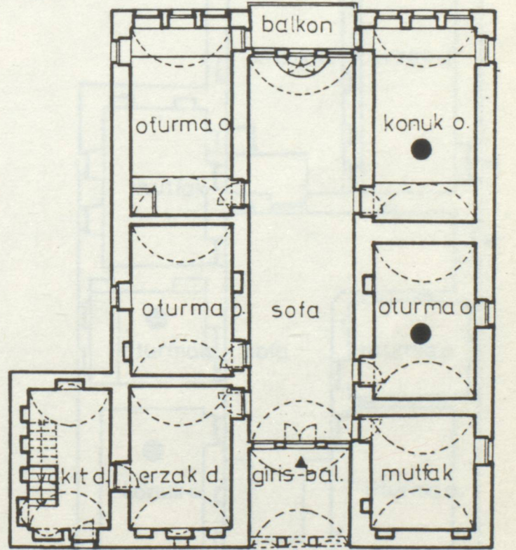
GİRİŞ KATI PLANI
