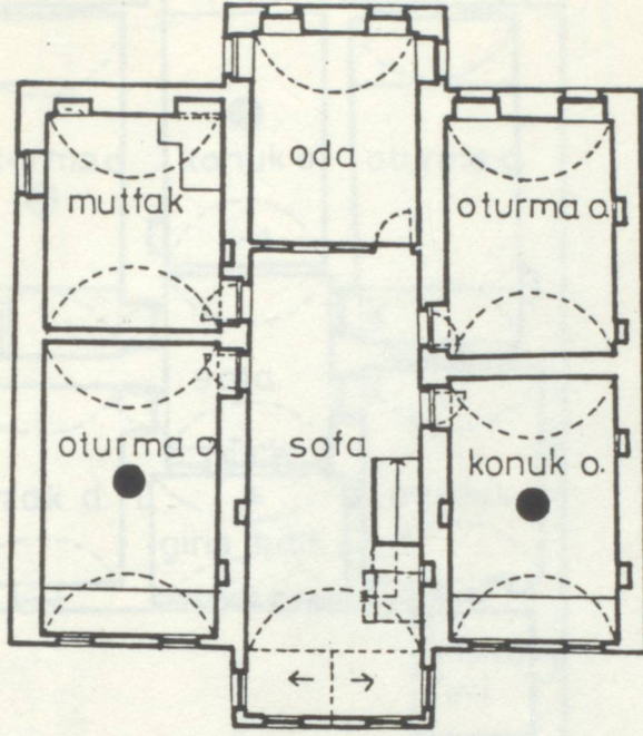
ÜST KAT PLANI
