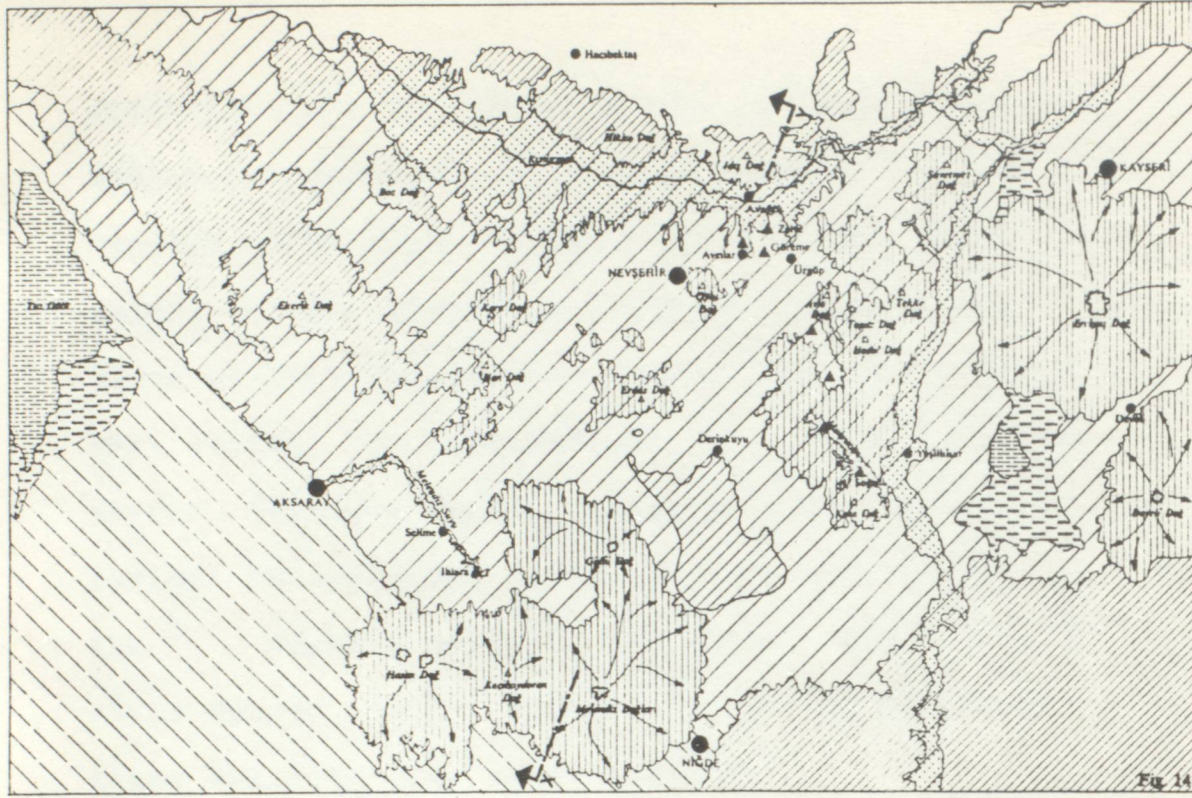
Çizim No.3: Kapadokya'nın Jeolojik Bölgeleri
