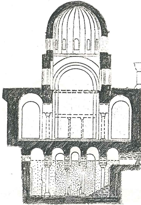
Kilisenin orjinal durumunu gösteren enine kesit (Hallensleben'den)
