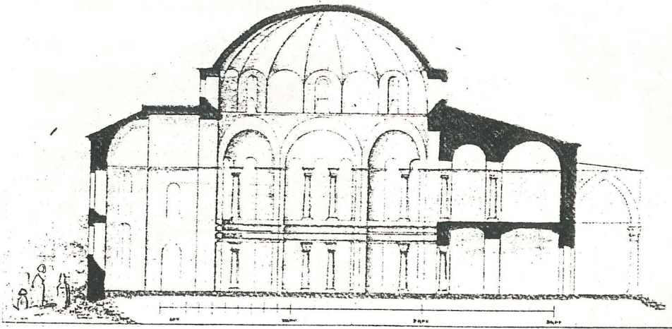
- 1878'de D.PULGHER tarafından çizilen kesidi.
