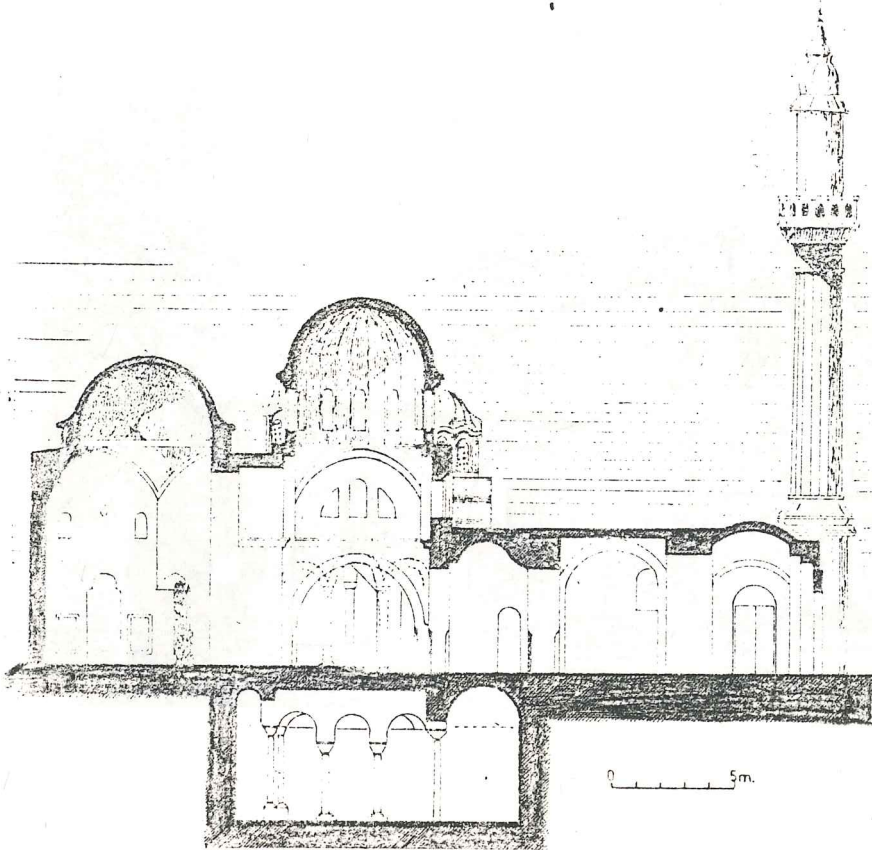
Yapının Fetihden sonraki konumu durumunu gösteren kesiti
