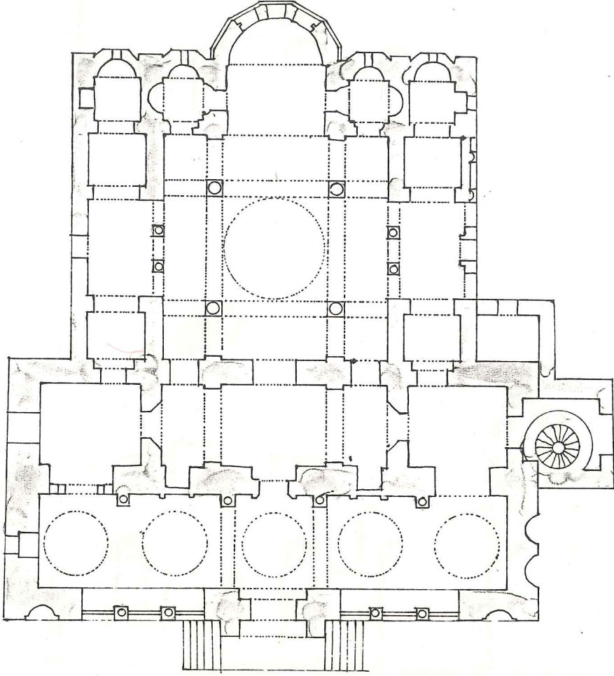
Kilise Camiinin 1840'larda Texier tarafından çizilen planı
