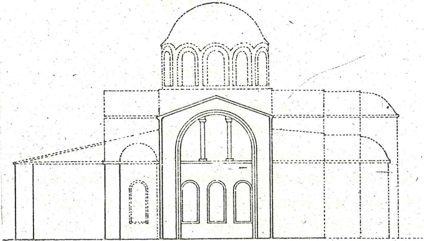
Enine kesit.
