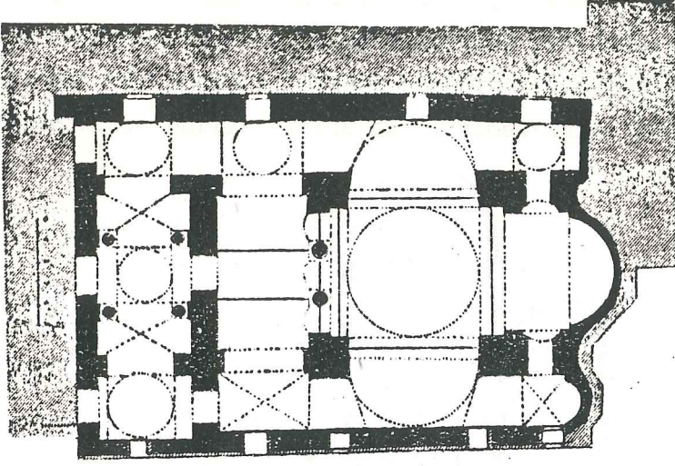
Koca Mustafa Paşa Camiinin planı
