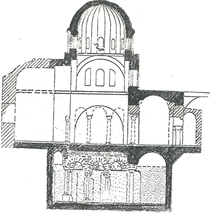
Fethiye Camii esas kilisesinin orjinal mimarisi ile boyuna kesit (Hallensleben'den)
