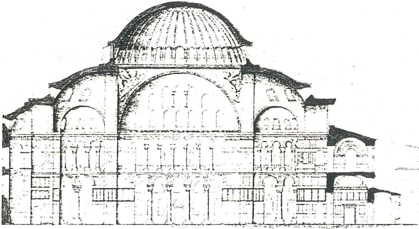
- 1878'de D.PULGHER tarafından çizilen kesidi.
