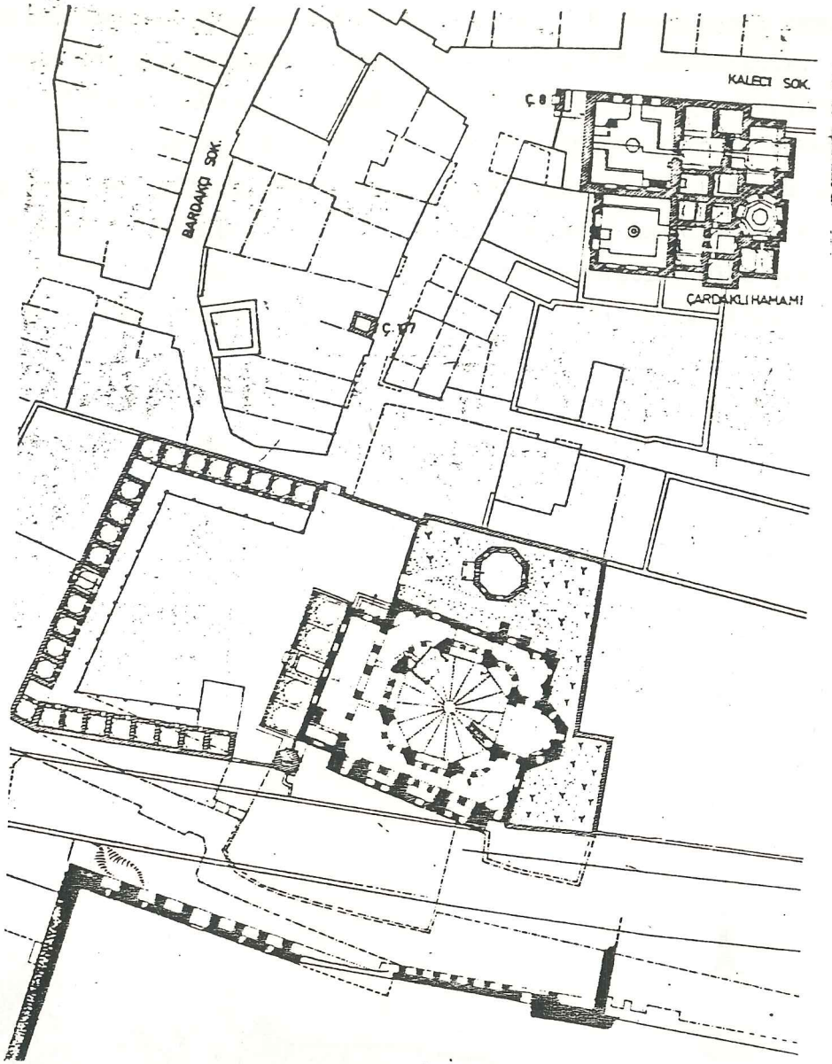
Konum planı
