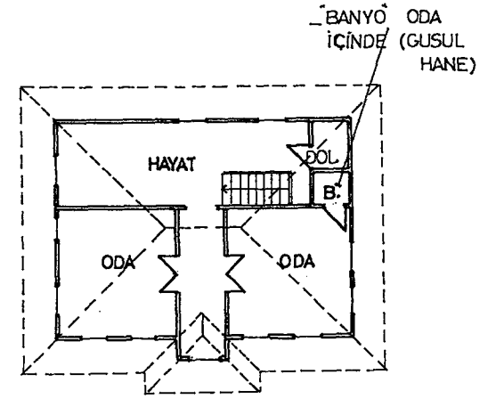
ÜST KAT
