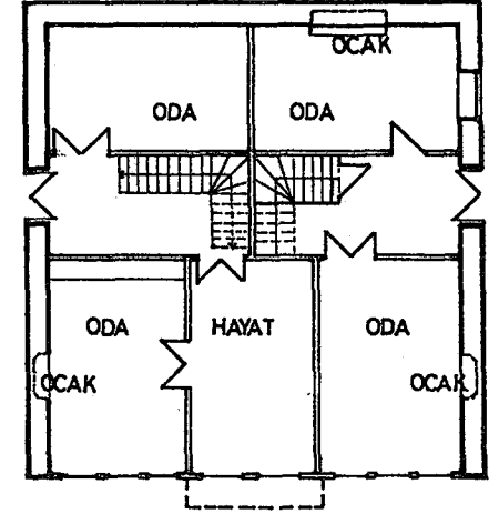
BİRİNCİ KAT
