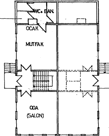
GİRİŞ KATI
