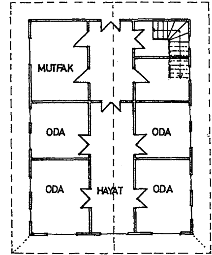
YAŞAMA KATI — ÇATI KATINA GİRİLEMEMİŞTİR.
