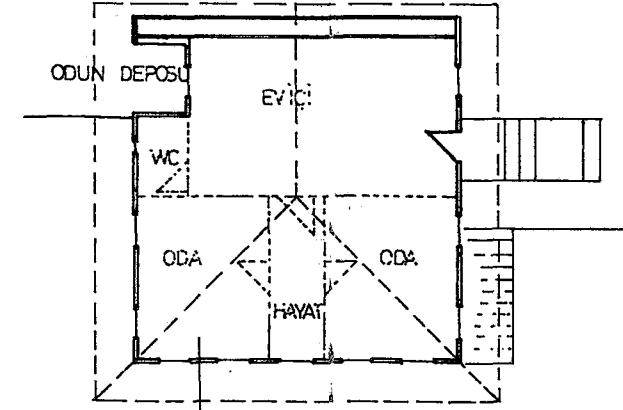
—İÇİNE GİRİLEMEDİ PLAN CEPHEDEN YARARLANILARAK TAHMİNİ OLARAK ÇİZİLDİ.
