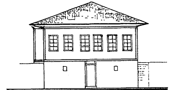
ÖN CEPHE
