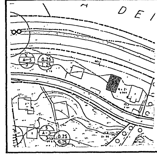
VAZİYET PLANI
