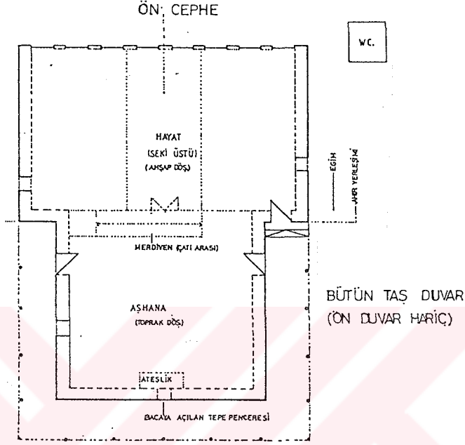
SÜRMENE-ORTA MAHALLEDE KONUT ÖRNEĞİ (P.1)
