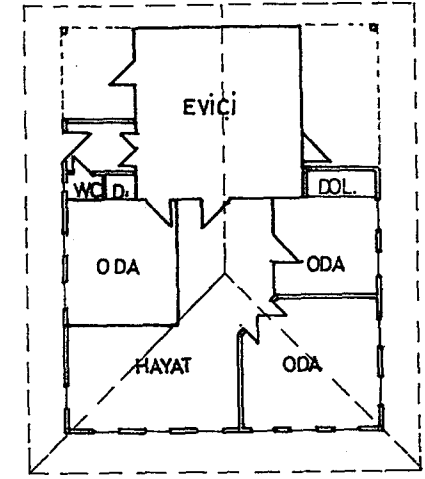
YAŞAMA KATI
