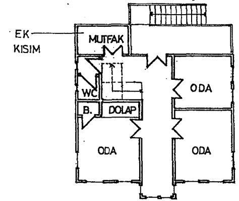
YAŞAMA KATI
