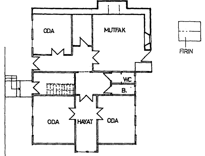
İKİNCİ KAT
