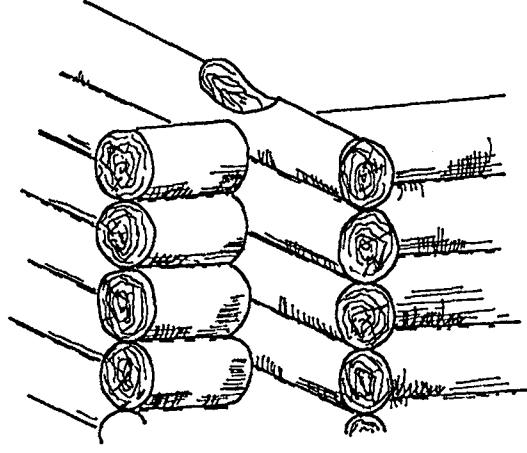
YUVARLAK AĞAÇ (TOMRUK) İLE YAPIM (ÖNEL, S. 29)
