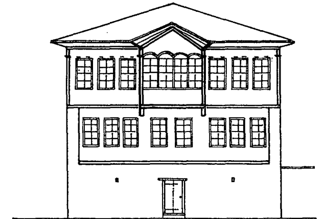
ÖN GÖRÜNÜŞ
