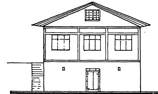
ÖN CEPHE
