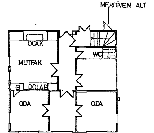
BİRİNCİ KAT
