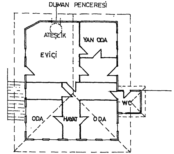
YAŞAMA KATI
