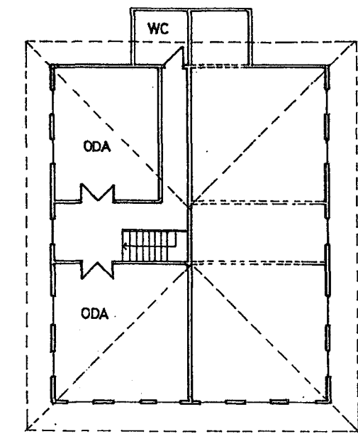
ÜST KAT
