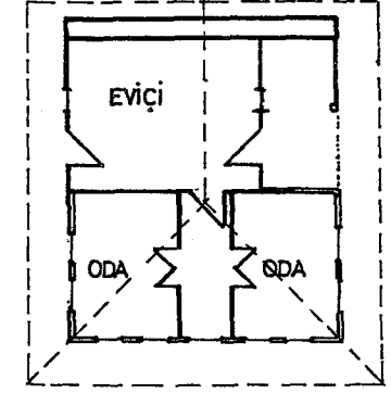
YAŞAMA KATI
