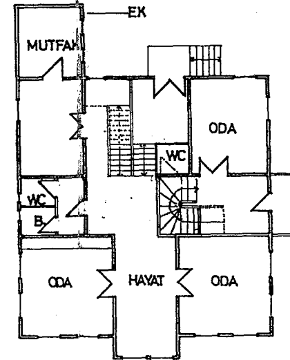
İKİNCİ KAT
