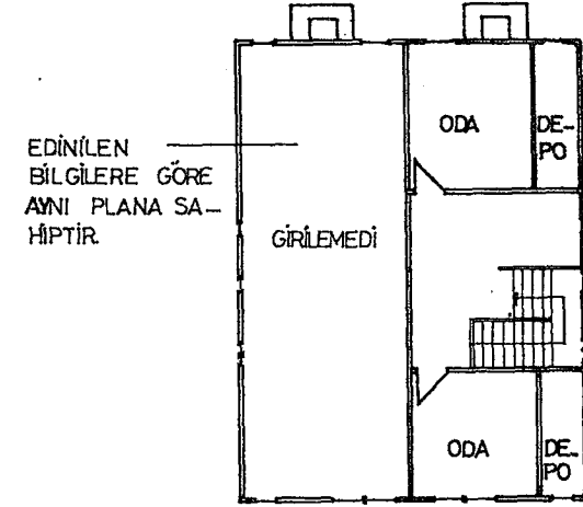
ÇATI KATI
