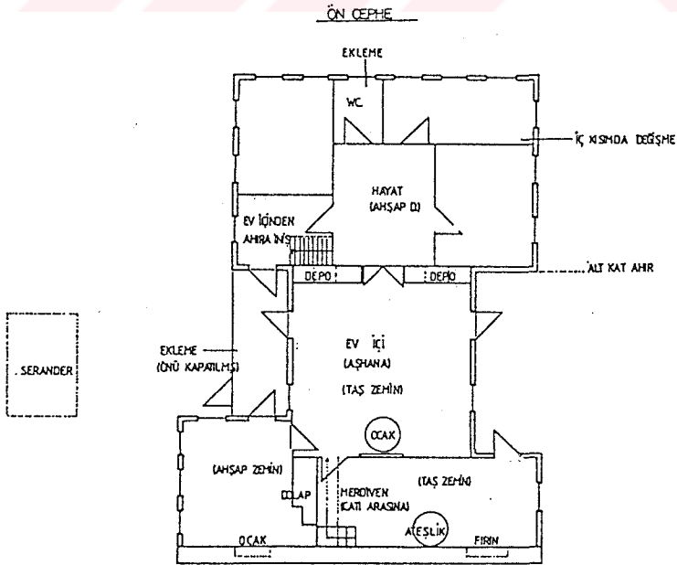
SÜRMENE ÜSTÜNDAL (KARAKANZI) KÖYÜNDE KONUT ÖRNEĞİ (P.5)
