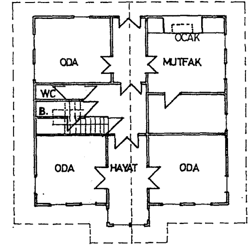
YAŞAMA KATI
