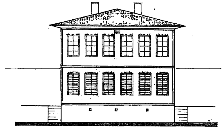
ÖN CEPHE
