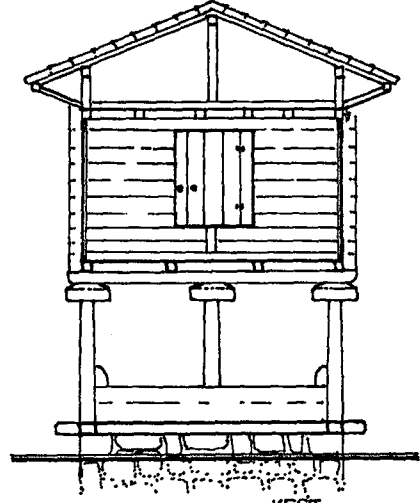
KESİT
