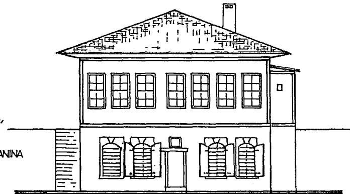
ÖN CEPHE
