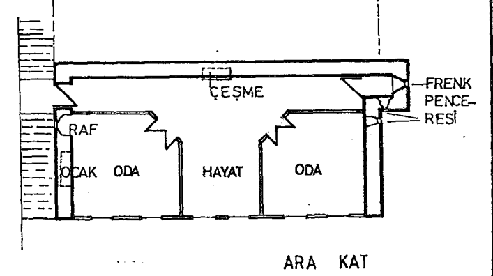
YAŞAMA KATI EDİNİLEN BİLGİLERE GÖRE ÇİZİLMİŞTİR
