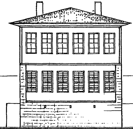
ÖN CEPHE
