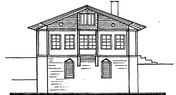
ÖN CEPHE
