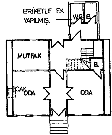
YAŞAMA KATI
