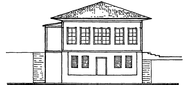
ÖN CEPHE
