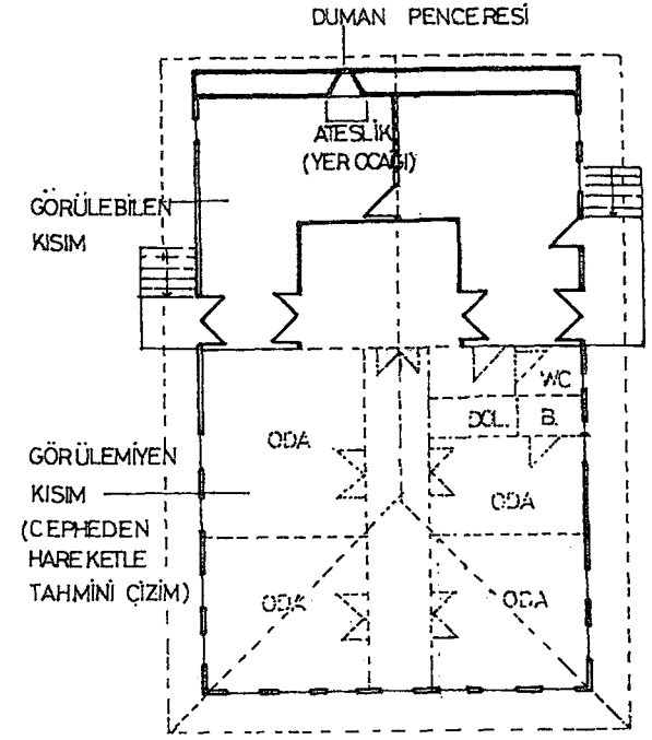
YAŞAMA KATI
