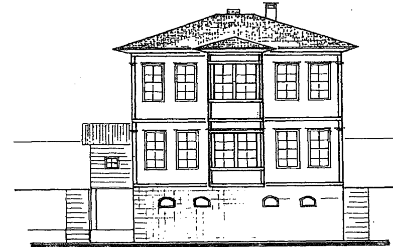
ÖN CEPHE
