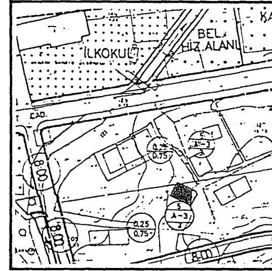
VAZİYET PLANI
