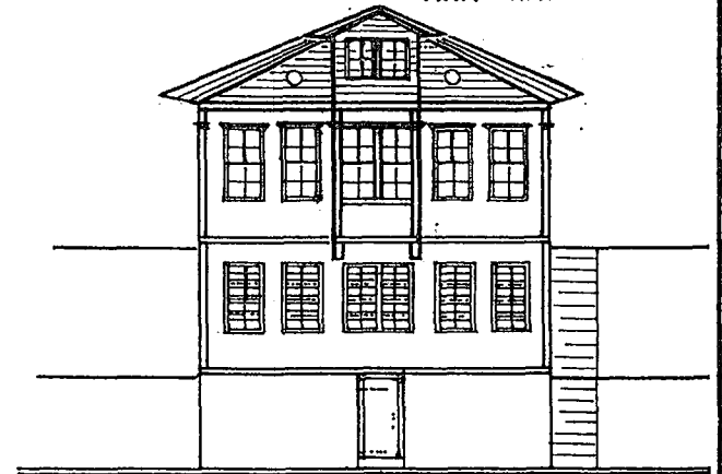
ÖN CEPHE
