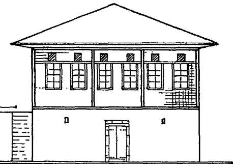
ÖN CEPHE RESTİTÜSYONU
