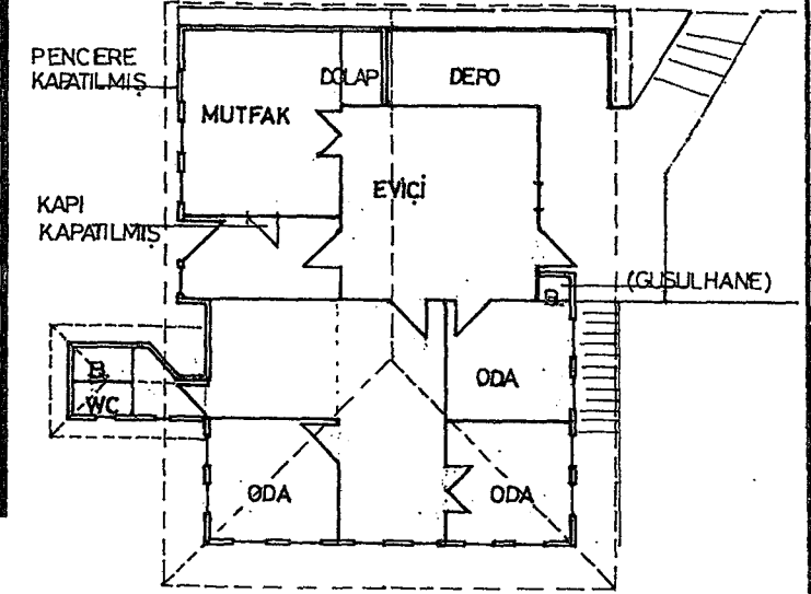
YAŞAMA KATI
