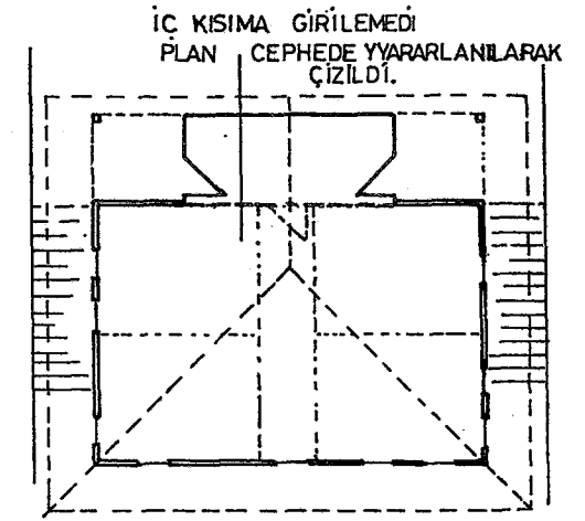
YAŞAMA KATI
