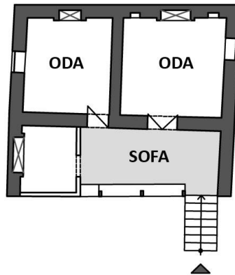
Şekil 4. 4 Sofanın kesintiye uğradığı plan tipi (Envanter no: 256)
