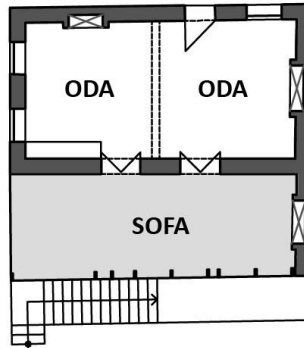
Şekil 4. 3 Sofanın cephe boyunca yer aldığı plan tipi (Envanter no: 258)
