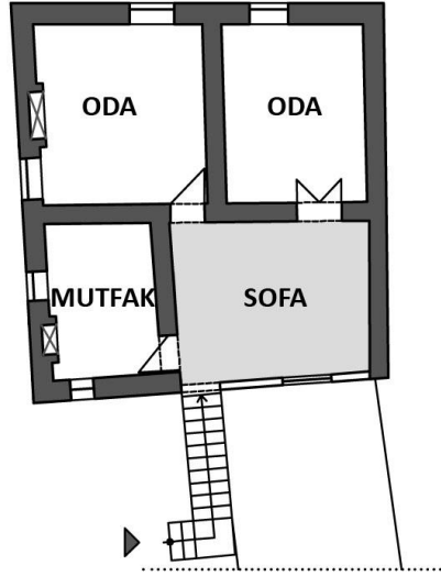
Şekil 4. 5 Üç odalı plan tipi (Envanter no: 33)
