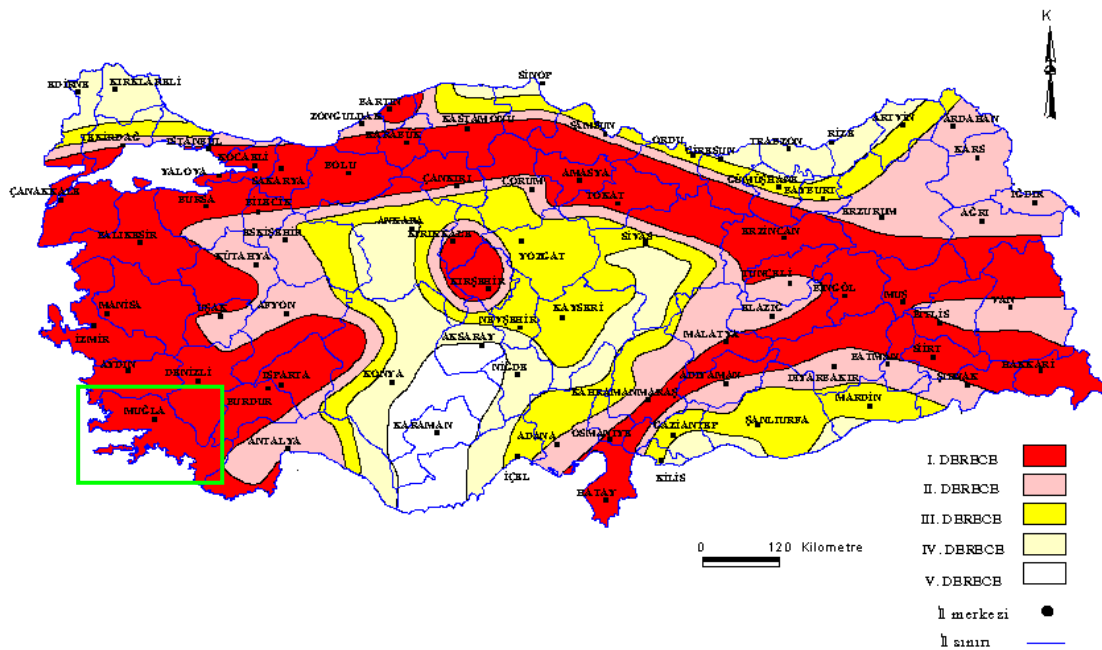
Şekil 2. 6 Türkiye deprem bölgeleri haritasında Muğla ili [9]
