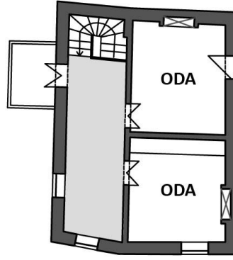
Şekil 4. 10 Merdivenin sofanın bir ucunda yer aldığı plan tipi (Envanter no: 50)
