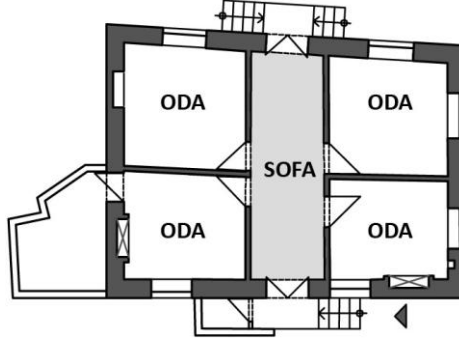
Şekil 4. 7 İç sofalı simetrik plan tipi (Envanter no: 170)
