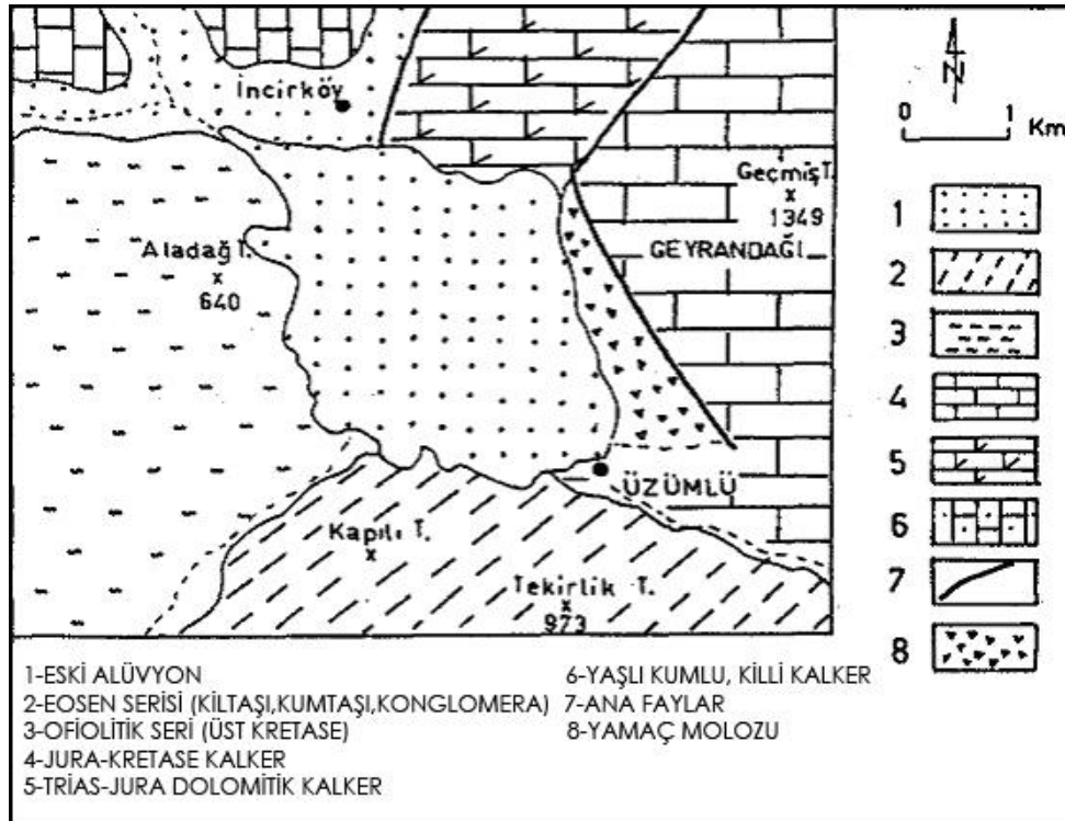
Şekil 2. 5 Üzümlü Ovası ve çevresinin jeoloji haritası [6]
