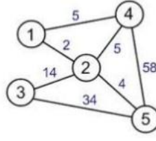
Şekil 2.3: Ağırlıklı Çizge
