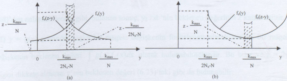
Şekil 6-11 Olasılık dağılım fonksiyonunun, konvolüsyon yöntemiyle bulunması
