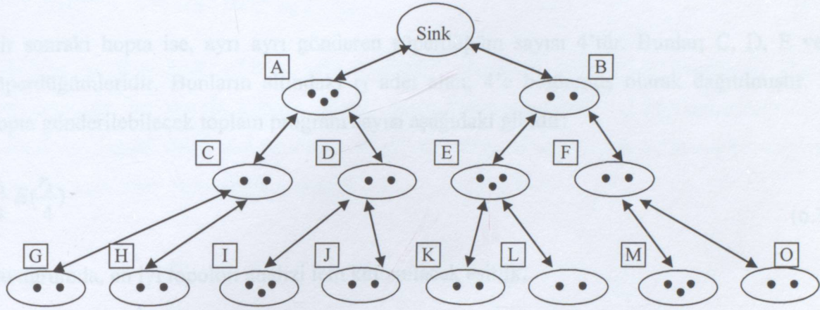
Şekil 6-19 Yeni ağ topolojisi
