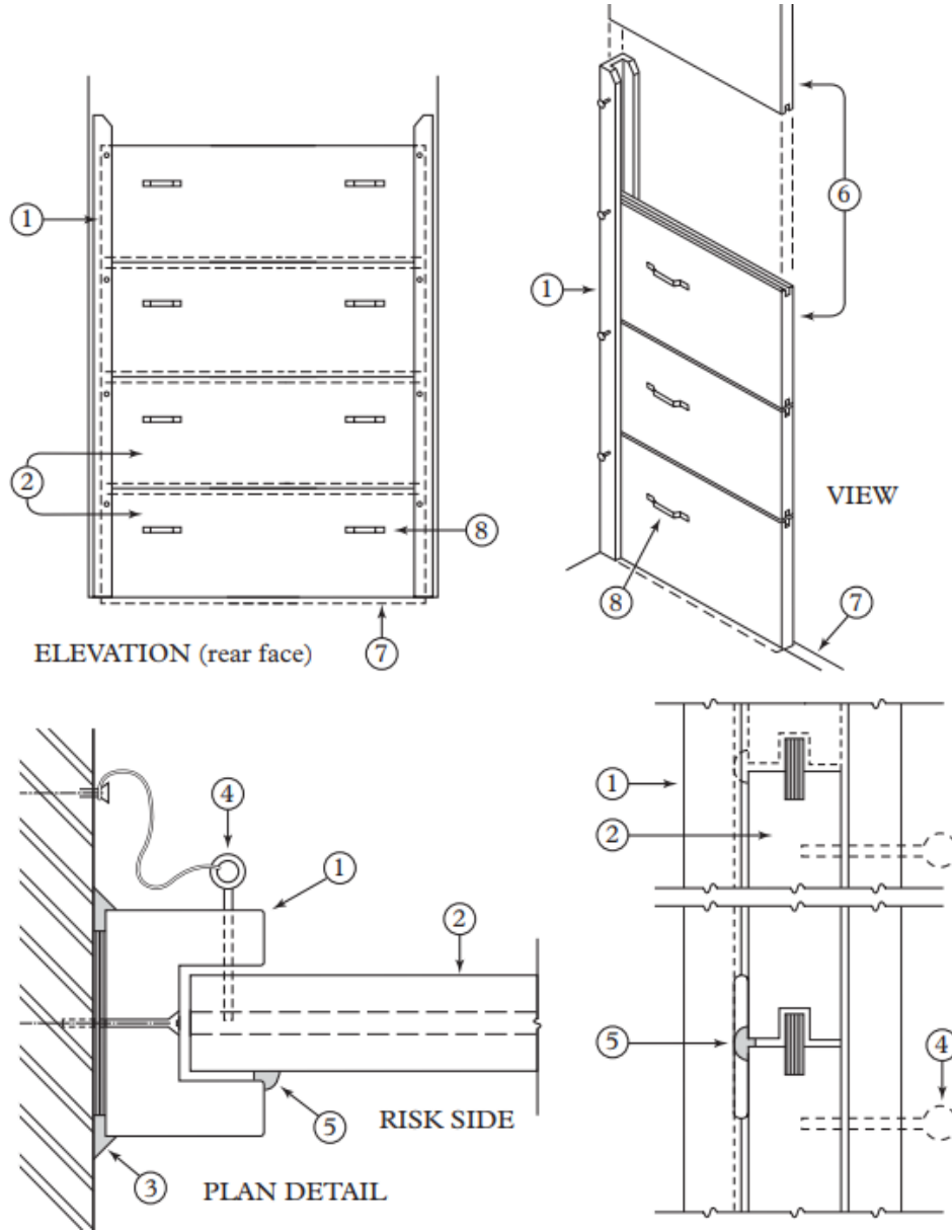
Şekil 3.46 Yükseltilebilir geçici sel bariyeri detayı (1- Kanal, 2- Bariyer, 3- Sızdırma önleyici, 4 Pim (Levhanın kalkmasını önlemek için), 5-Sızdırma önleyici, 6- Ek levha, 7- Kanal, 8- Kaldırma kol )(English Heritage, 2015)
