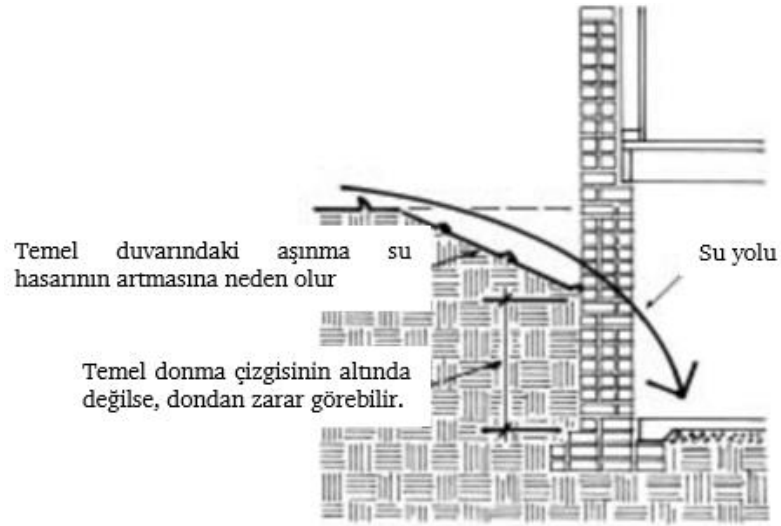
Şekil 3.29 Selin temel duvarı etrafındaki toprağı aşındırması (National Trust, 2005)
