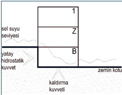
Şekil 4.13 G4.2’ye ait şema ve sele bağlı ortaya çıkan etkiler (Gökmen Erdoğan, 2021)
