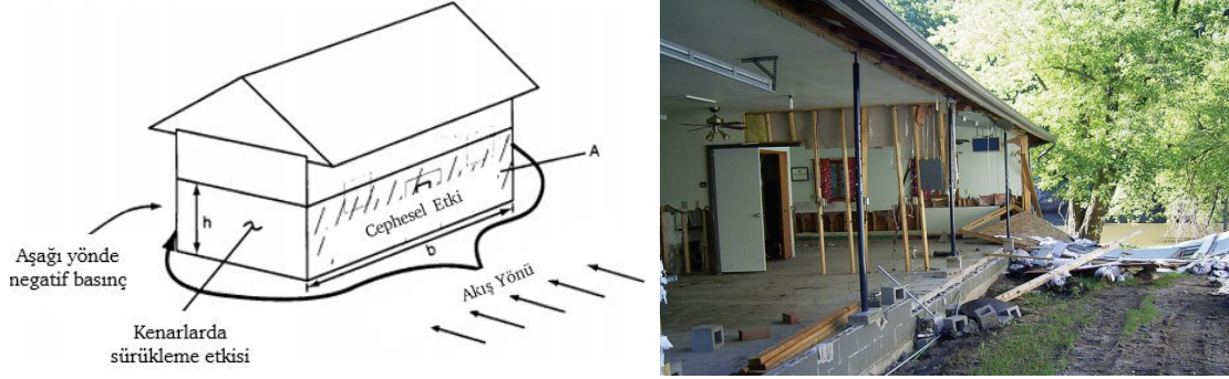
Şekil 3.20 Yapı üzerinde sel kaynaklı yatay hidrodinamik kuvvetler (FEMA, 1998)
