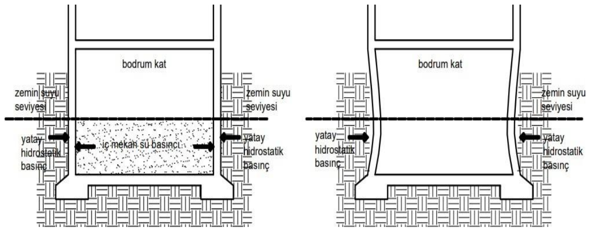
Şekil 3.36 Bodrum kattaki sel suları tahliye edilmeden önce (sol) ve edildikten sonraki (sağ) kuvvetler (National Trust, 2005).
