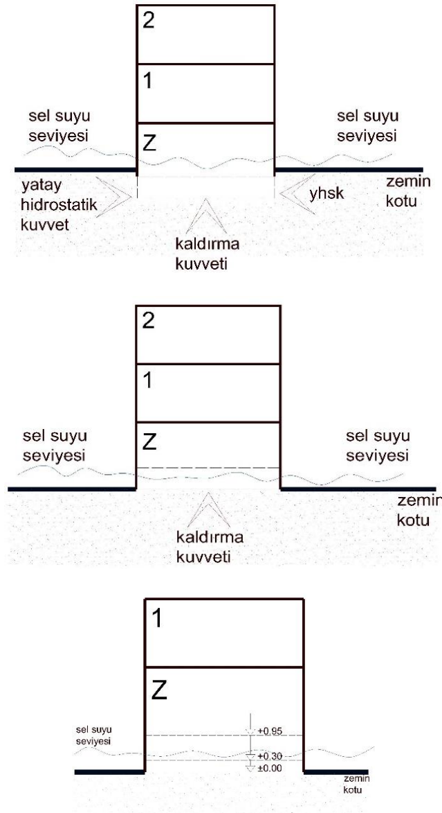
Şekil 4.14 G4.3, G4.4 ve G4.5 şematik gösterim (Yukarıdan aşağıda)
