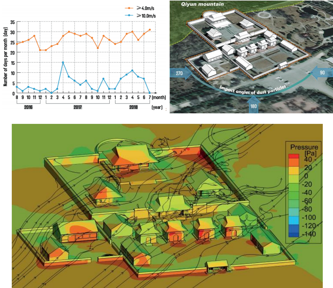
Şekil 2.29 Yongling Mozolesi'nde rüzgar erozyonu çalışması (Wang vd., 2019)
