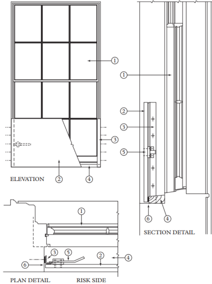
Şekil 3.48 Pencere için geçici bariyer detayı (1- Pencere kanadı, 2- Bariyer (Su geçirmez malzemeden levha şeklinde), 3- Metal köşe tutucu: Su geçirmez mastiksel sabitlenmiş), 4- Ahşap destek, 5- Kilit, 6- Köpük yalıtım) (English Heritage, 2015)
