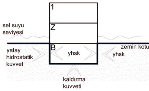
Şekil 4.12 G4.1’e ait şema ve sele bağlı oluşan etki ve kuvvetler (Gökmen Erdoğan, 2021)
