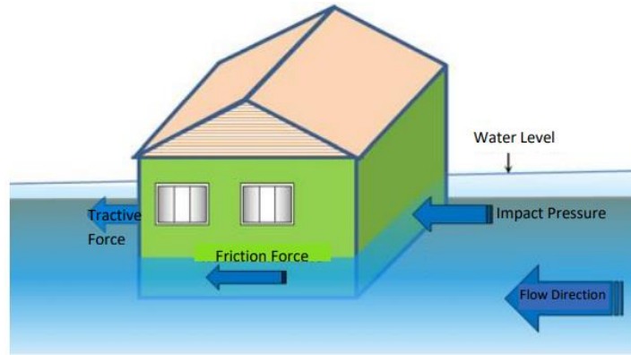
Şekil 2.24 Sel sularının oluşturduğu etki ve kuvvetler (Bikçe vd., 2018)
