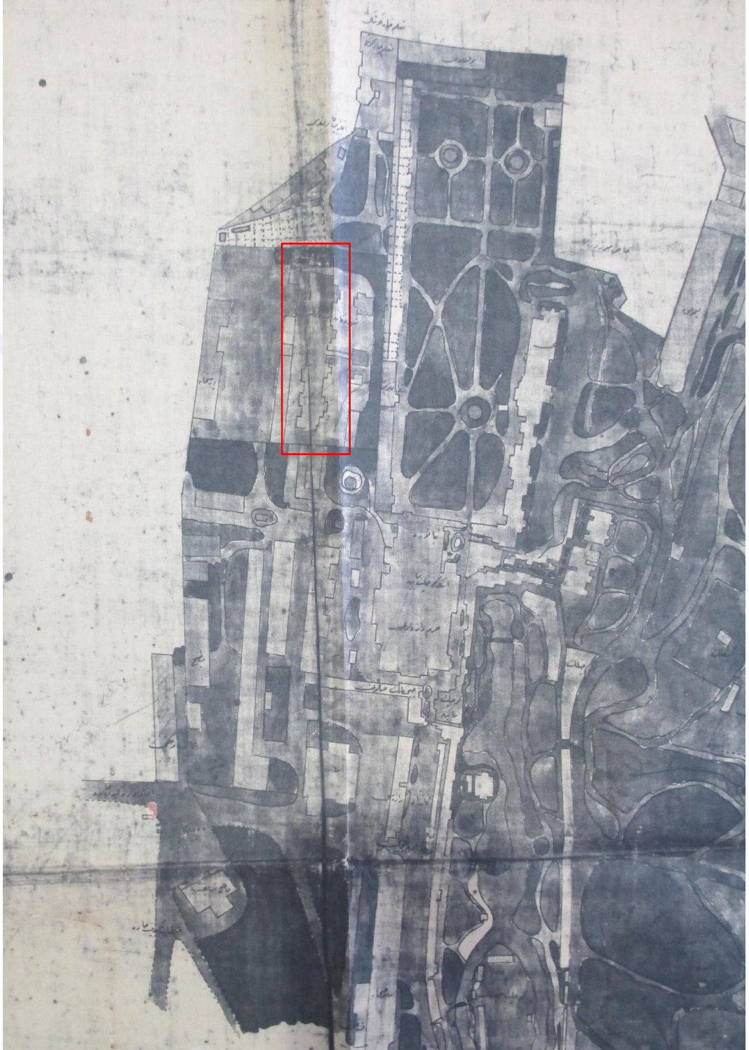
Şekil 4.115 Osmanlıca hazırlanmış vaziyet planı, 1928 öncesi (İstanbul III Numaralı KVKBKM Arşivi, Yıldız Sarayı Dosyası)
