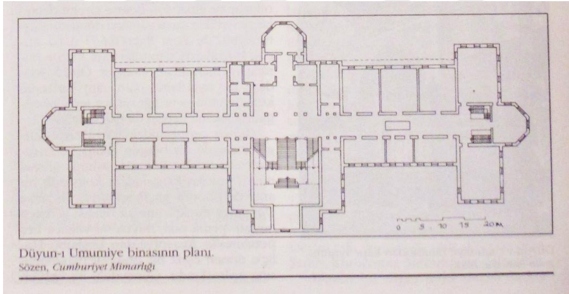
Şekil 4.74 Özgün plan (Dünden Bugüne İstanbul Ansiklopedisi, cilt 3, 1994, s. 111)
