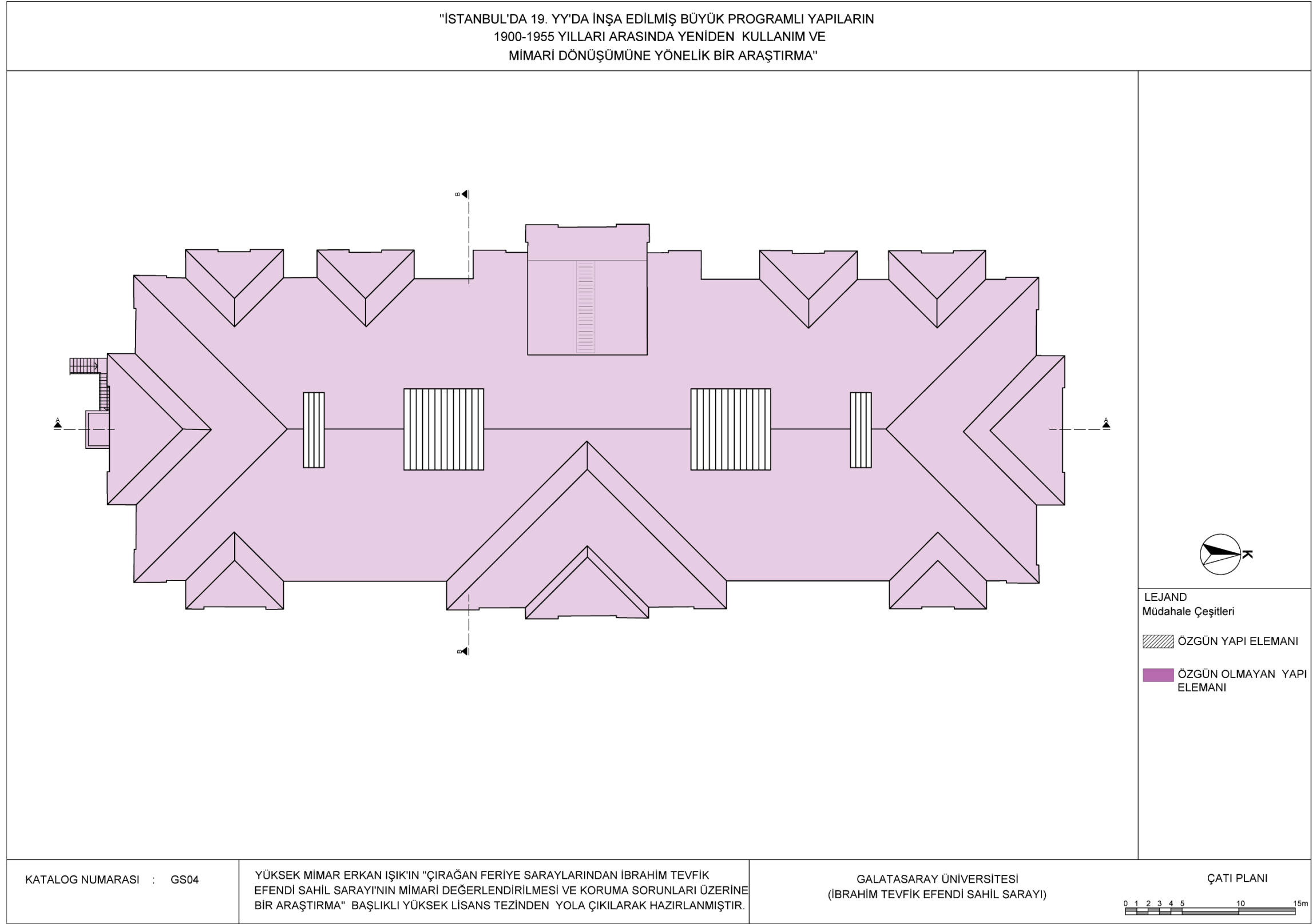
Şekil 4.271 GSÜ çatı planı (Kaytan, 2022)
