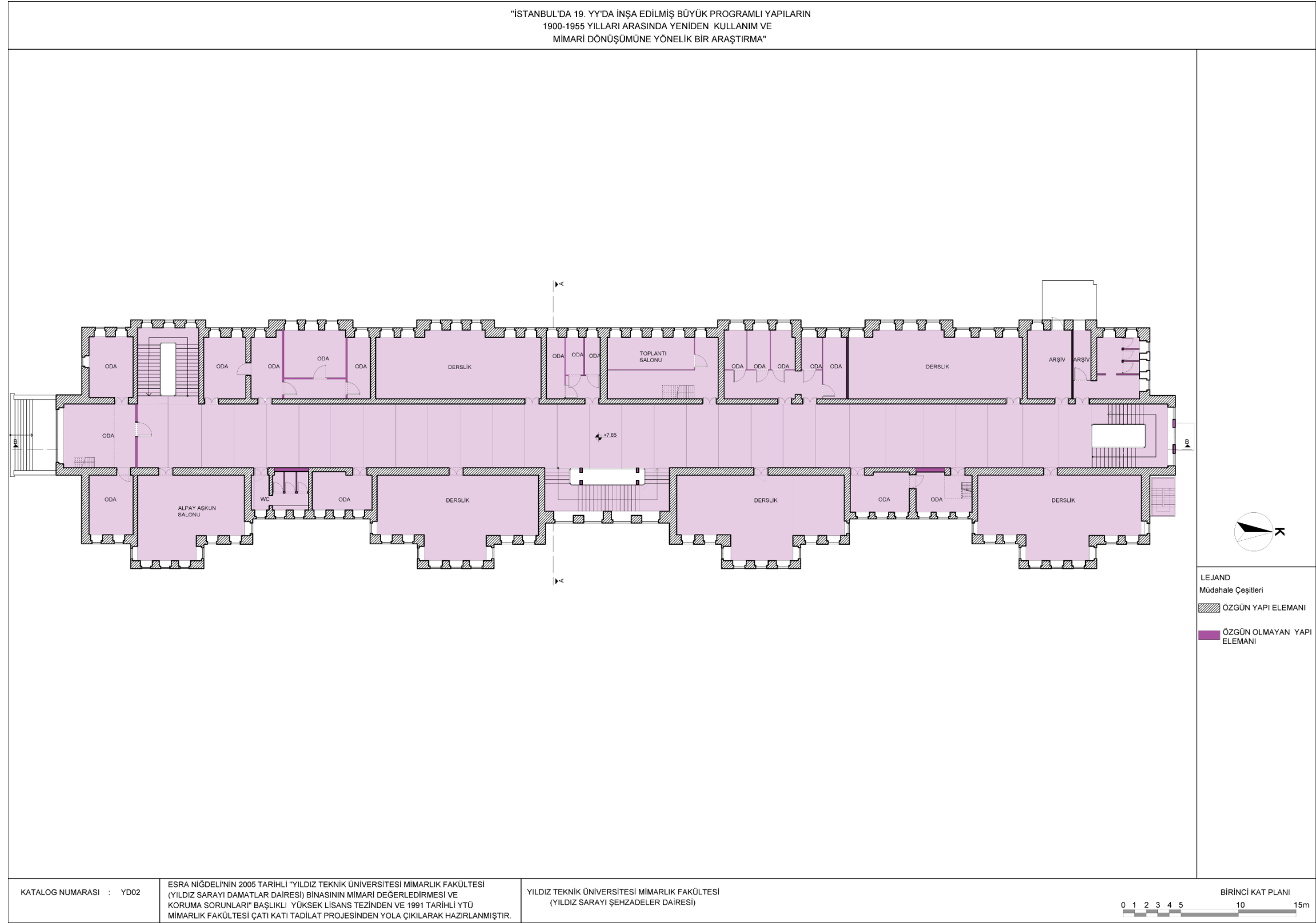
Şekil 4.134 YTÜ Mimarlık Fakültesi birinci kat planı (Kaytan, 2022)
