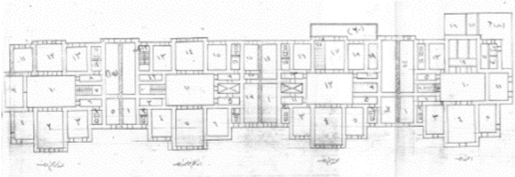
Şekil 4.119 1937 uygulaması öncesi özgün bodrum kat planı (Niğdeli, s. 70)
