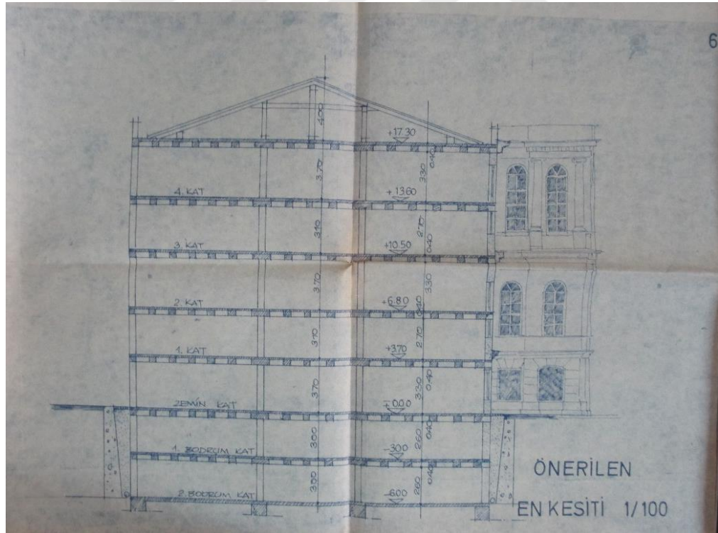
Şekil 4.20 Restorasyon projesi, enine kesit (13125, 1981)
