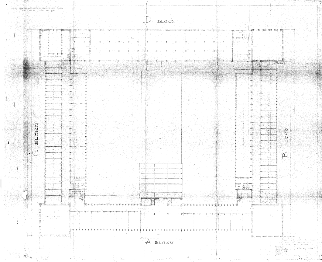
Şekil 4.33 İTÜ Makina ve Elektrik Fakülteleri Binası İlave Çatı Katı Planı (İstanbul II Numaralı KTVKBKM)
