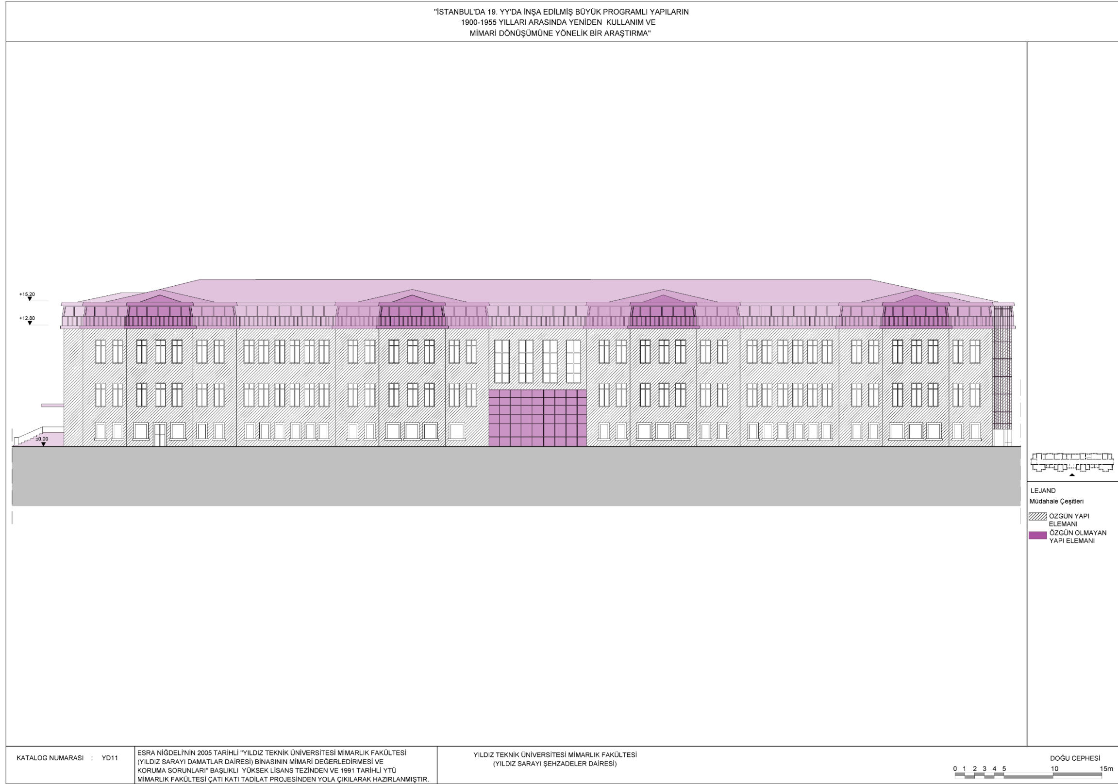
Şekil 4.143 YTÜ Mimarlık Fakültesi doğu cephesi (Kaytan, 2022)
