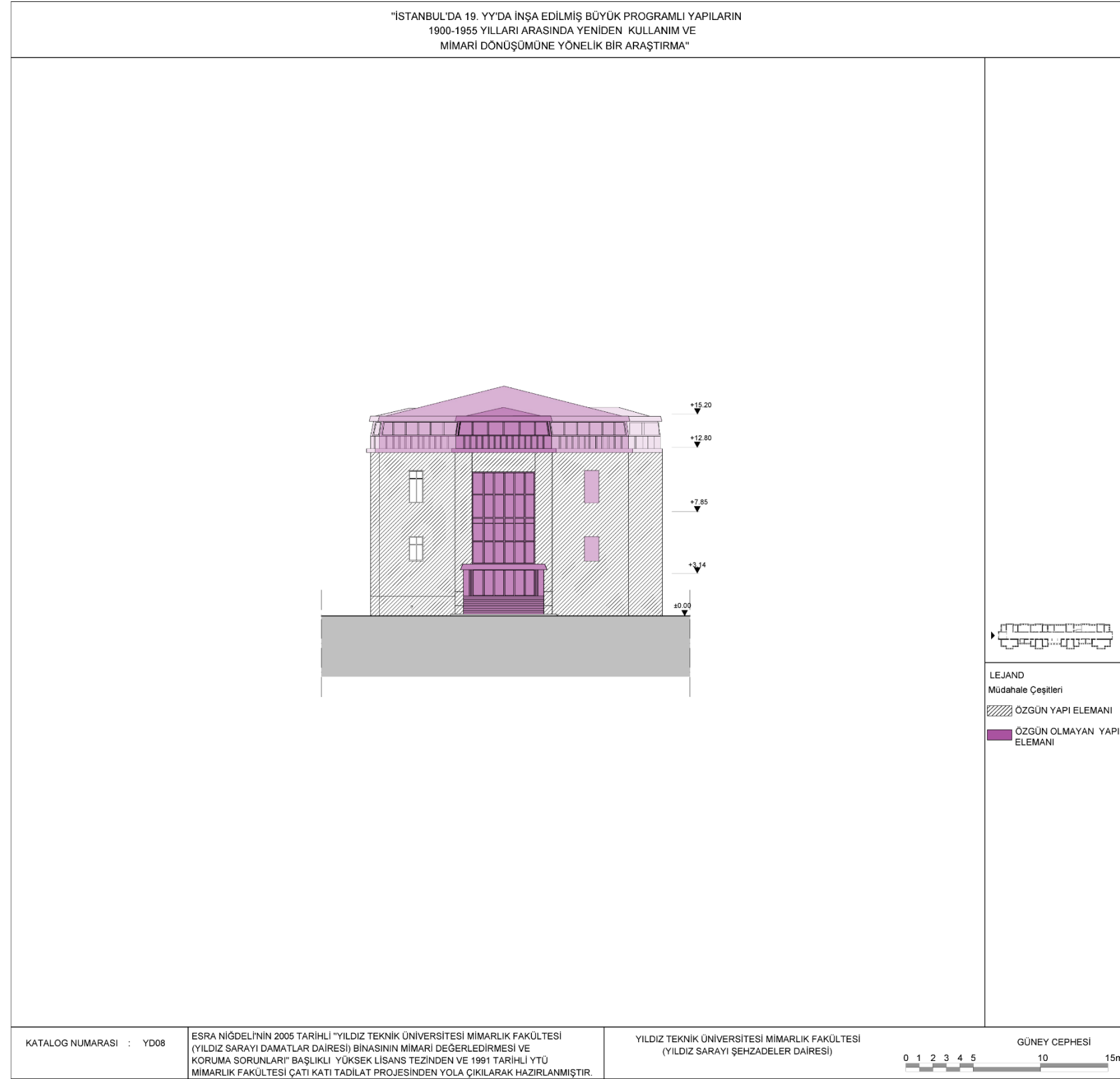
Şekil 4.140 YTÜ Mimarlık Fakültesi güney cephesi (Kaytan, 2022)
