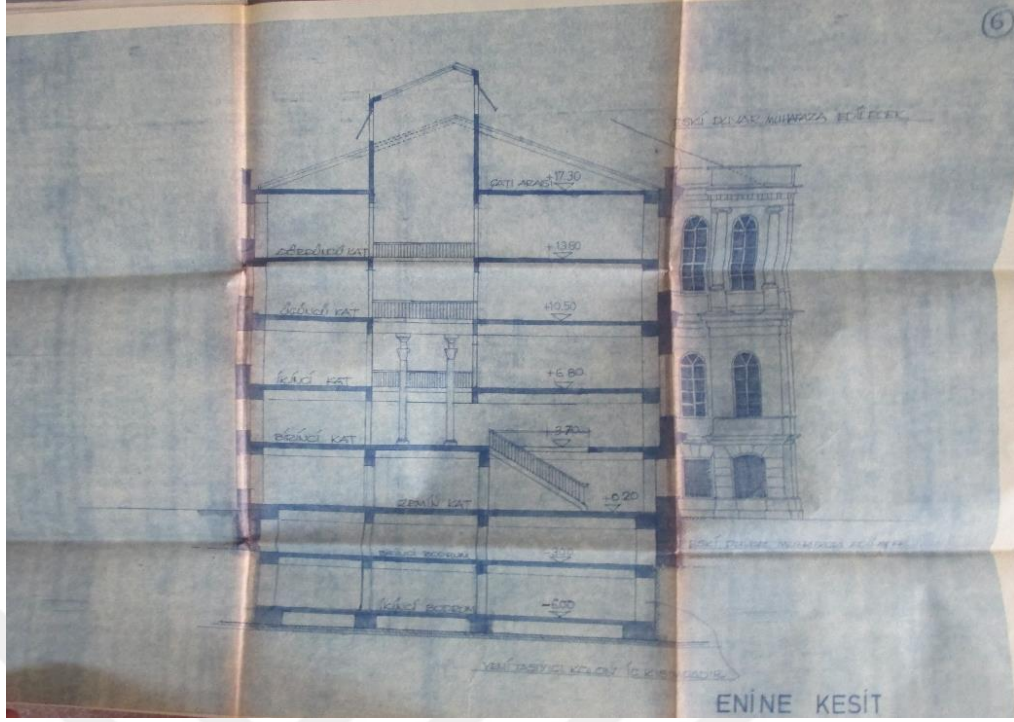
Şekil 4.19 Rölöve, enine kesit (13125, 1981)
