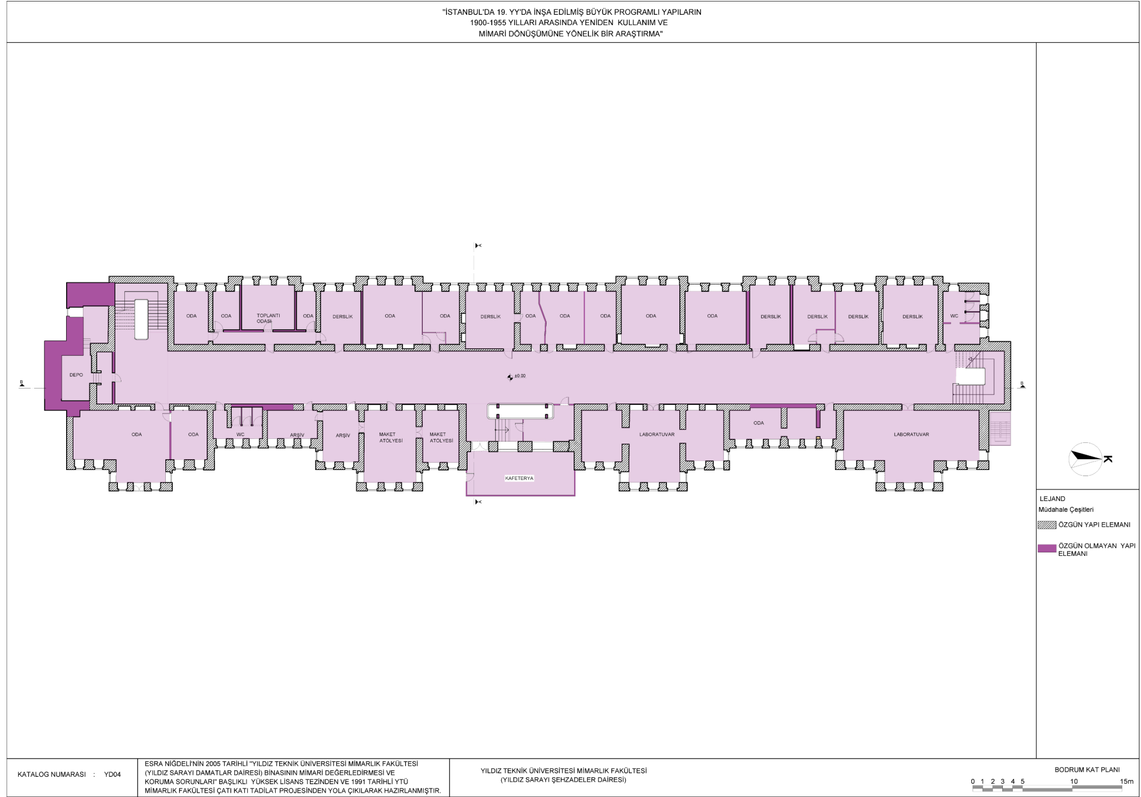
Şekil 4.136 YTÜ Mimarlık Fakültesi bodrum katı planı (Kaytan, 2022)
