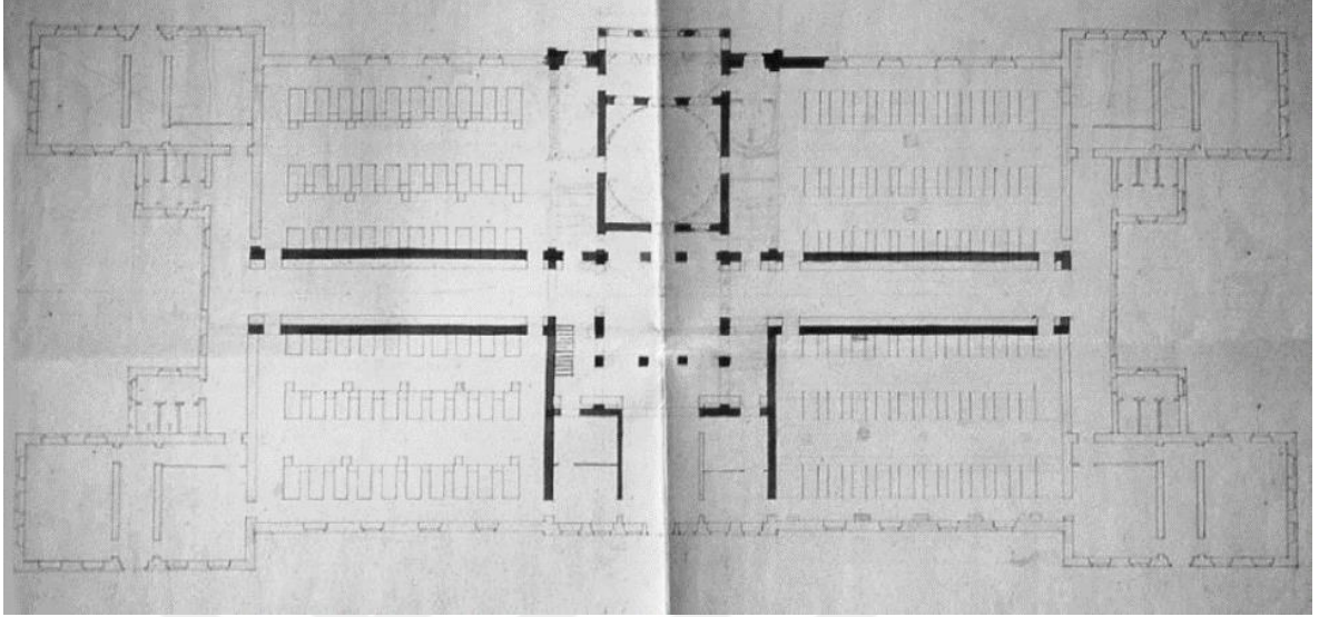
Şekil 4.68 İsviçre Bellnizona Cantonale arşivi Fossati özgün projesi – plan (Cengiz Can arşivi)
