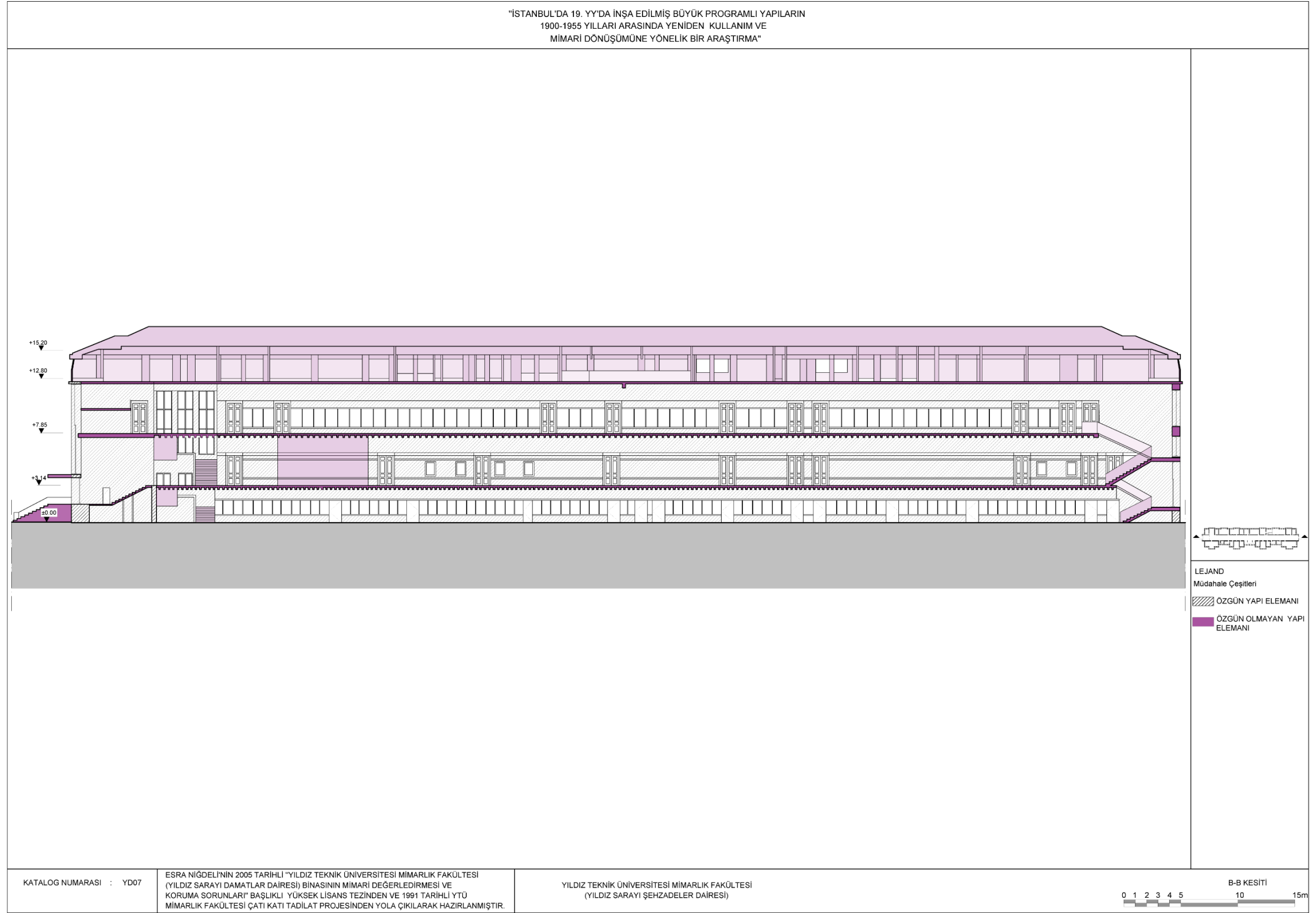
Şekil 4.139 YTÜ Mimarlık Fakültesi B-B kesiti (Kaytan, 2022)
