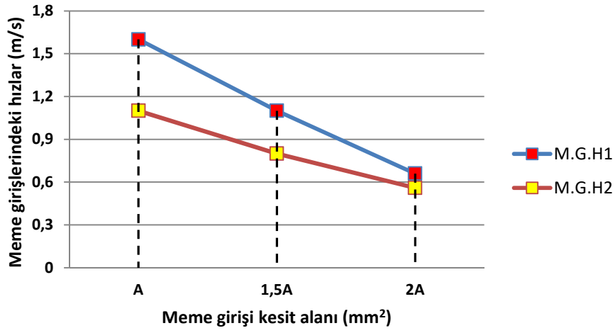
Şekil 5.22 Meme girişi kesit alanının hıza etkisi
