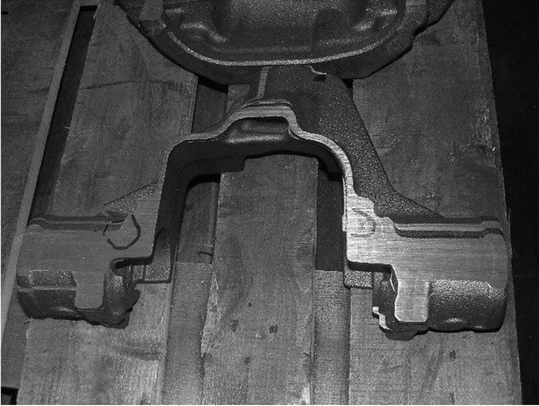
Şekil 6.48 Parçanın kesit görüntüsü ve çekinti
