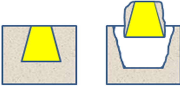
Şekil 2.2 Ters açıda kalan yüzeylerin olduğu model ile kalıplama
