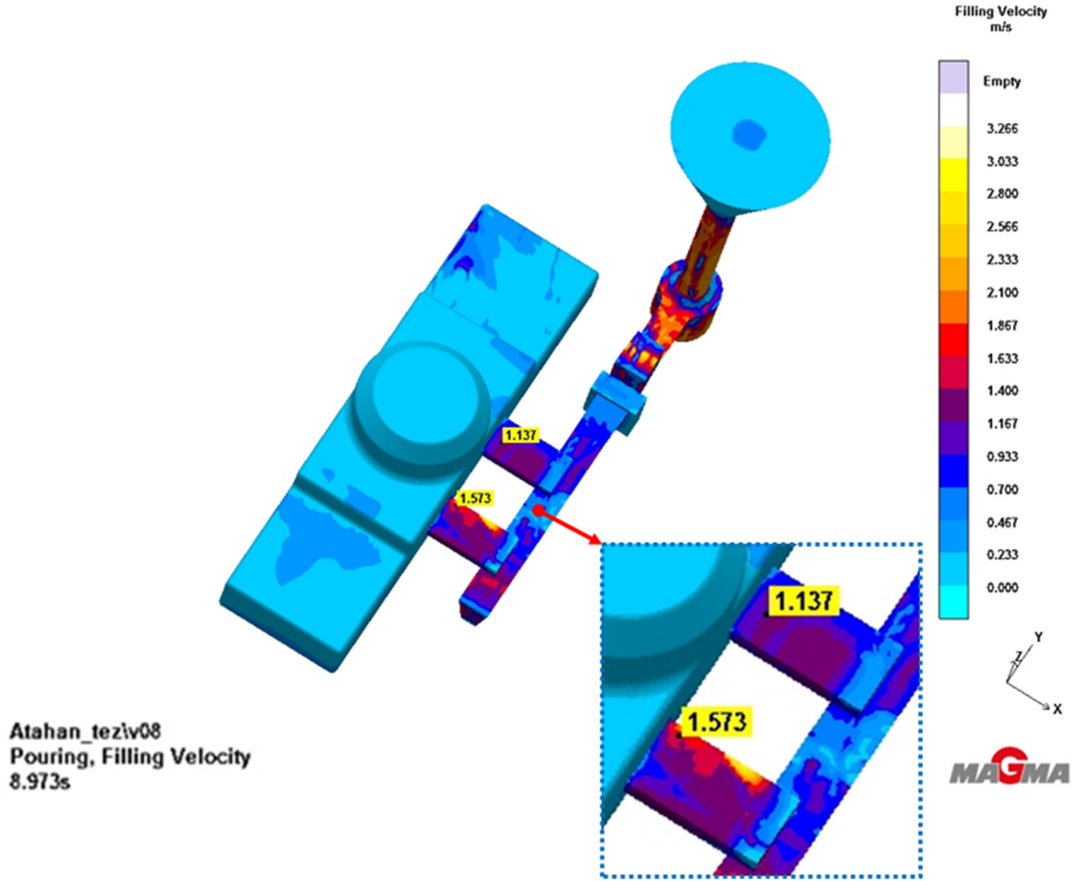
Şekil 5.12 Hesaplanan kesit alanları ile yapılan dizaynda okunan meme girişi hızları
