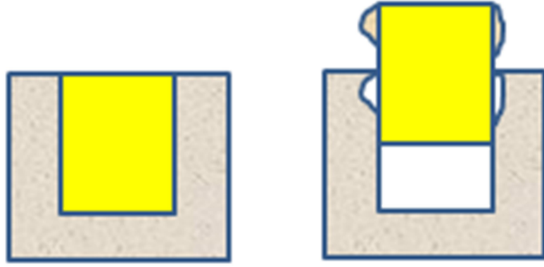
Şekil 2.1 Koniklik verilmemiş model ile kalıplama
