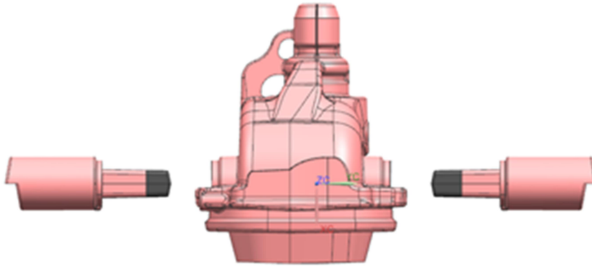
Şekil 6.22 Maçaların beraber görünümü
