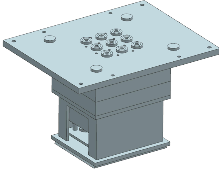
Şekil 2.9 Maça sandığı dış görünüm
