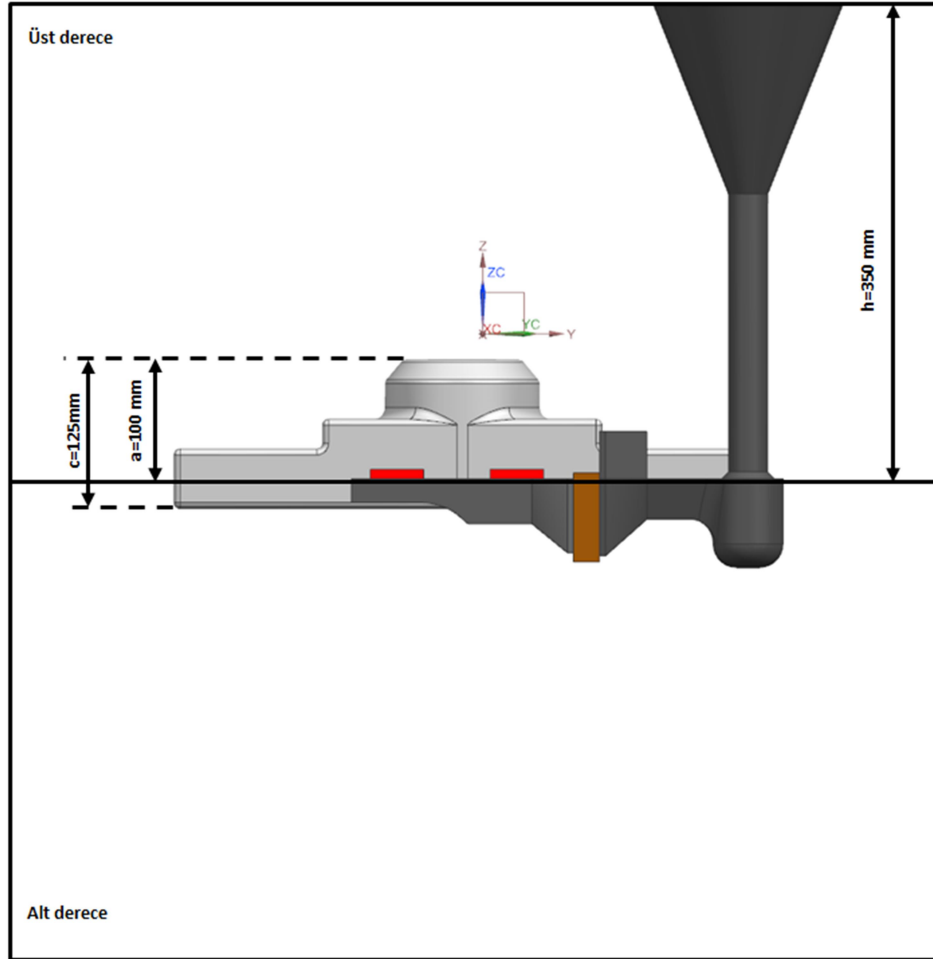
Şekil 5.11 Örnek parçanın derece içerisindeki konumu ölçüleri
