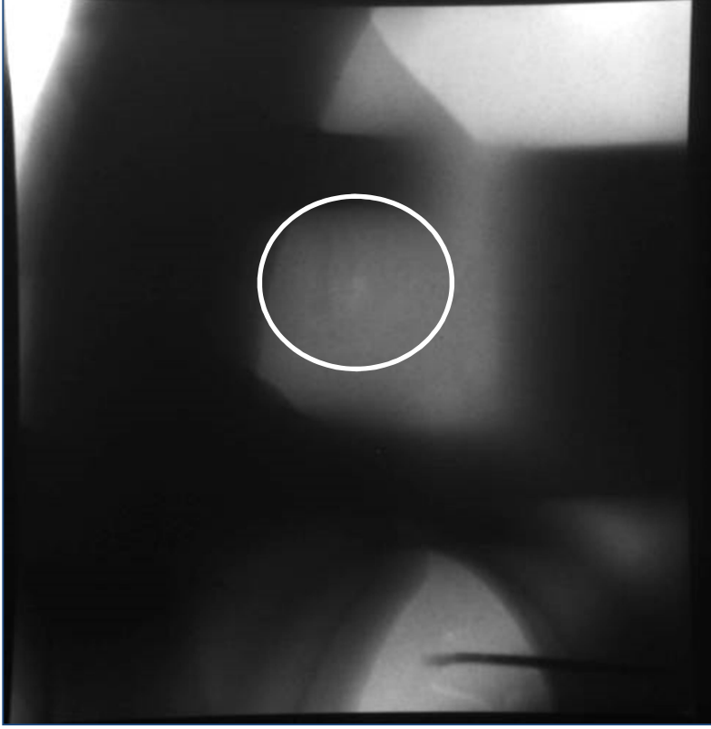
Şekil 6.63 Yeni yolluk ile dökülen parçanın x-ray kontrolleri
