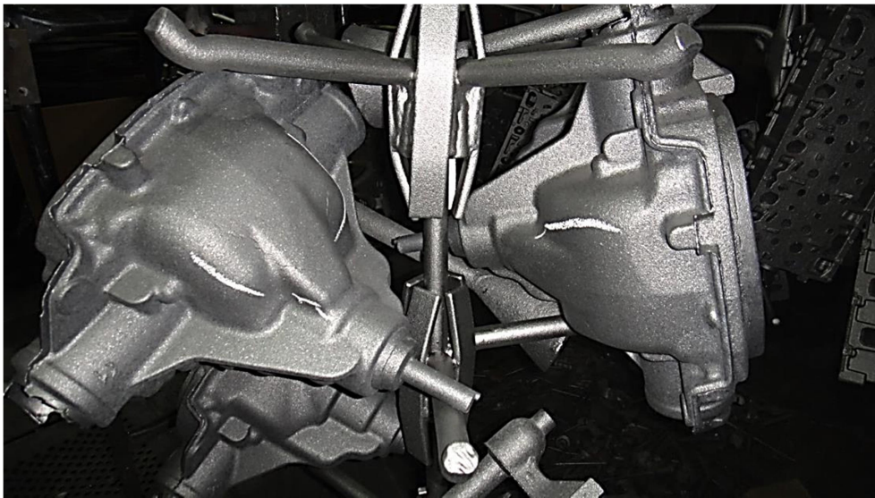
Şekil 6.32 Askılı temizlemeden çıkan parçalar
