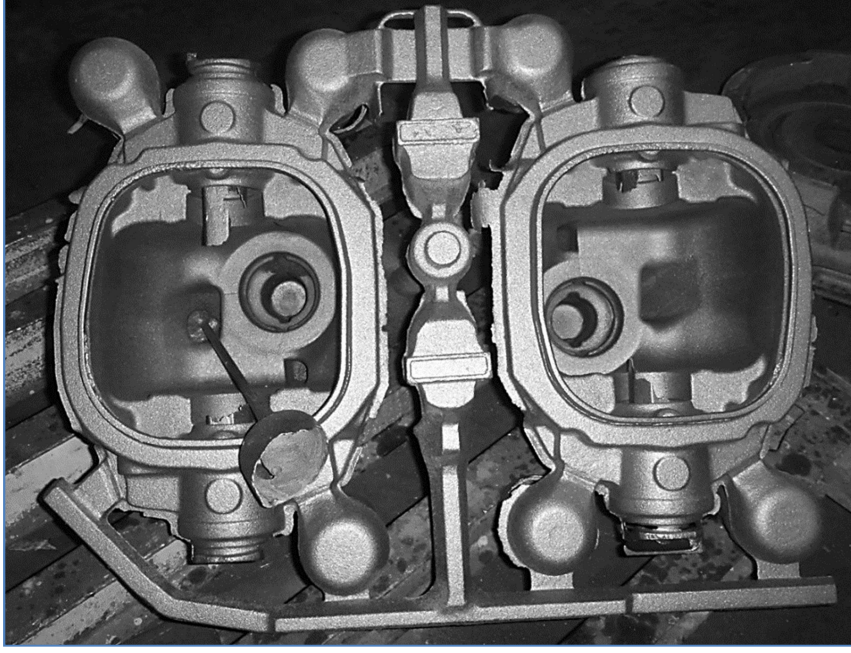
Şekil 6.57 Yeni yolluk dizaynı ile yolluklu proje parçası
