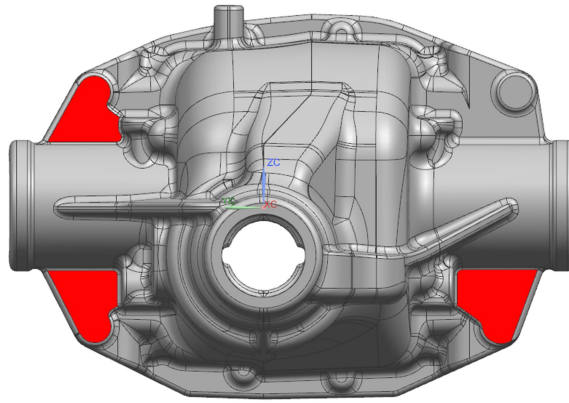
Şekil 6.51 Modifikasyon çalışması
