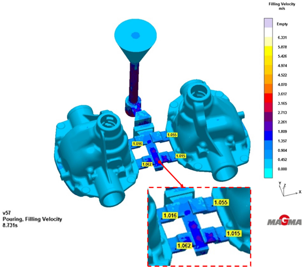
Şekil 6.24 Proje parçası dolum simülasyonu
