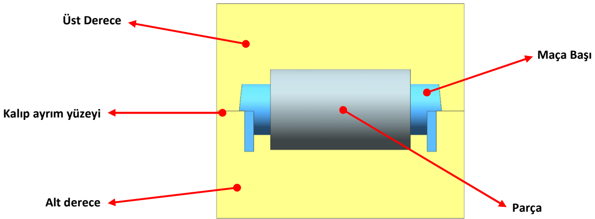
Şekil 2.5 Parçanın maça başı ile derece içerisindeki görünümü
