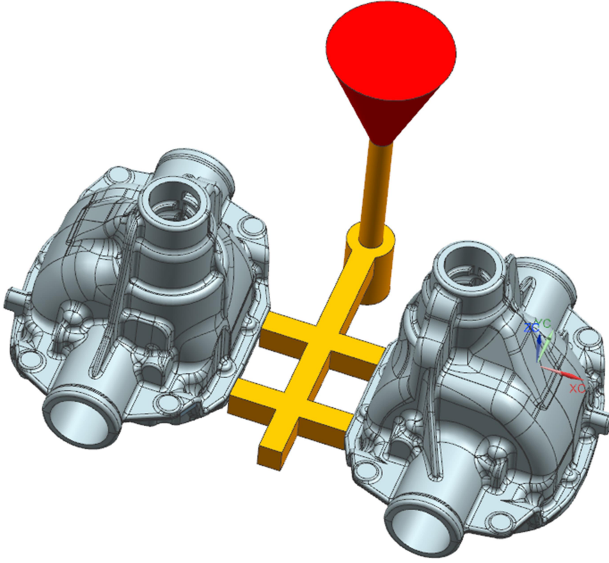
Şekil 6.5 Yolluk taslağı
