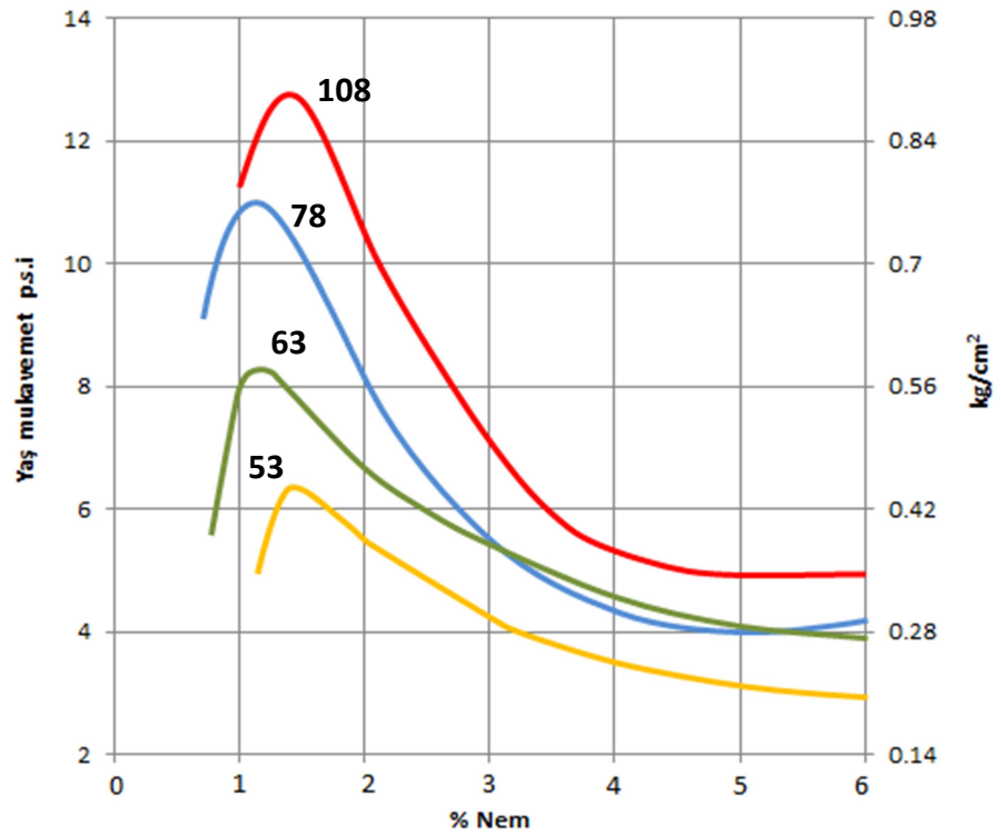
Şekil 2.30 Farklı tane inceliklerine göre yaş mukavemet değişimi [6]
