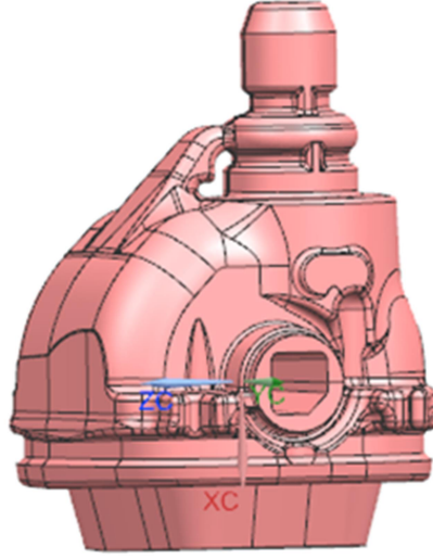
Şekil 6.20 Gövde maça
