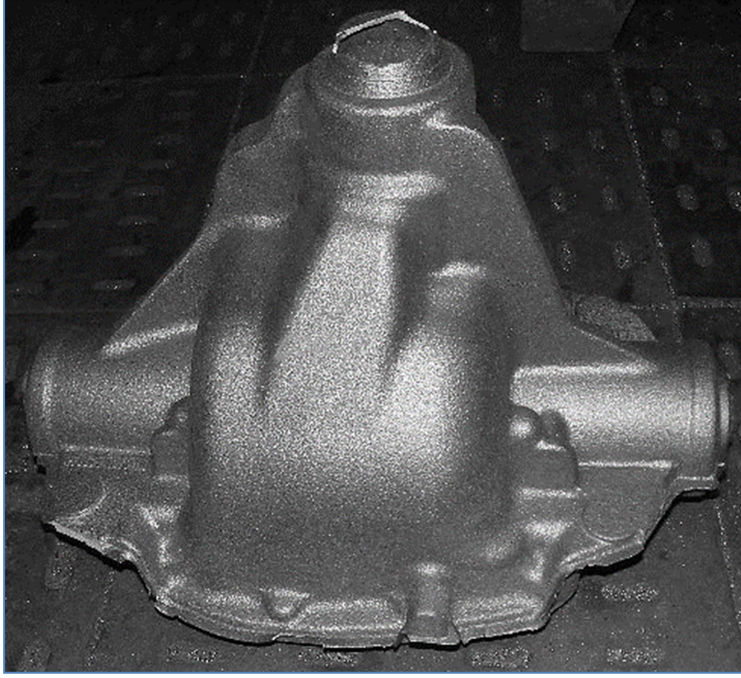
Şekil 6.58 Yeni yolluk ile dökülen parçalarda katmer sakatı gözlemi
