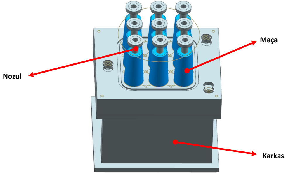
Şekil 2.10 Maça ve nozullar ile gösterilen ayrıntılı maça sandığı görünümü
