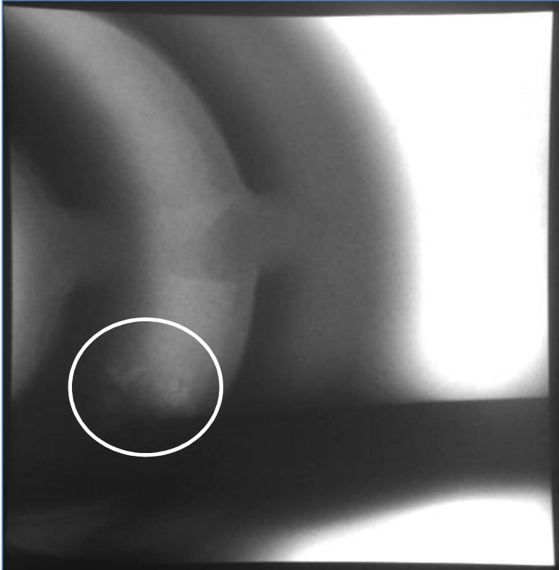
Şekil 6.60 Yeni yolluk ile dökülen parçanın x-ray kontrolleri
