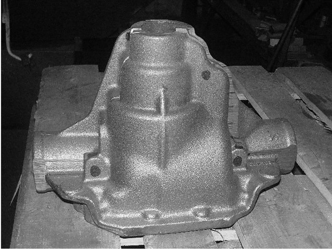
Şekil 6.41 X-ray sonucunda tespit edilen çekinti bölgeleri
