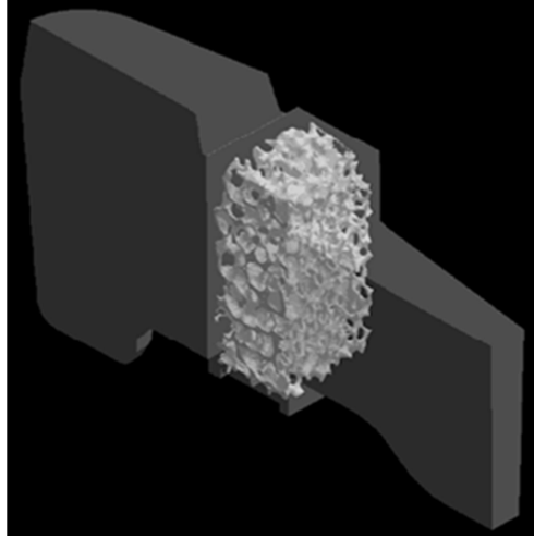
Şekil 2.48 Köpük filtrenin yolluk sistemi içerisindeki görünümü[10]
