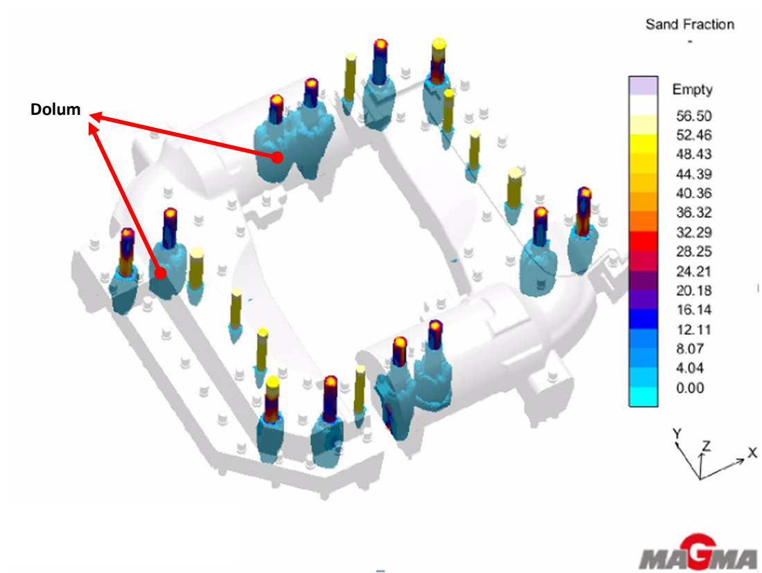
Şekil 2.13 Maça dolum simülasyonu 2
