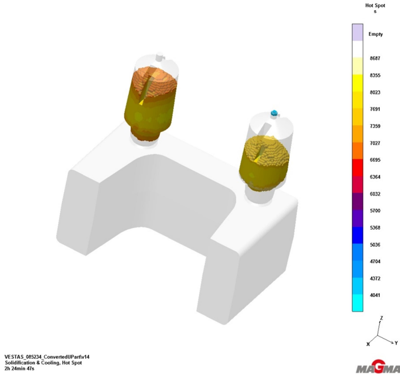
Şekil 2.58 Besleyiciler ile sıcak bölgelerin belirlenmesi
