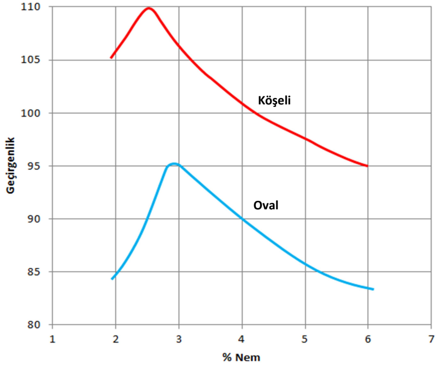
Şekil 2.34 Kum şekli ve geçirgenlik arasındaki ilişkinin gösterildiği grafik [6]
