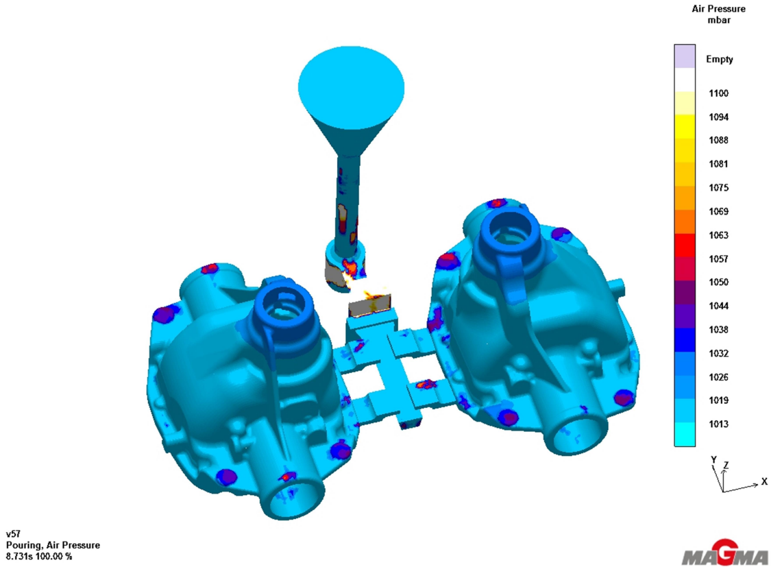
Şekil 6.26 Proje parçası hava basıncı
