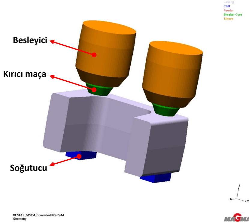
Şekil 2.57 Belirlenen modüllere göre besleyici seçimi
