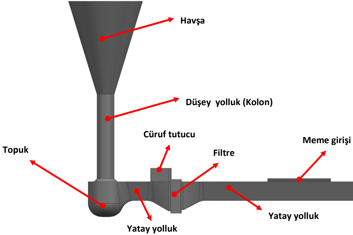
Şekil 2.44 Yolluk sisteminin unsurları
