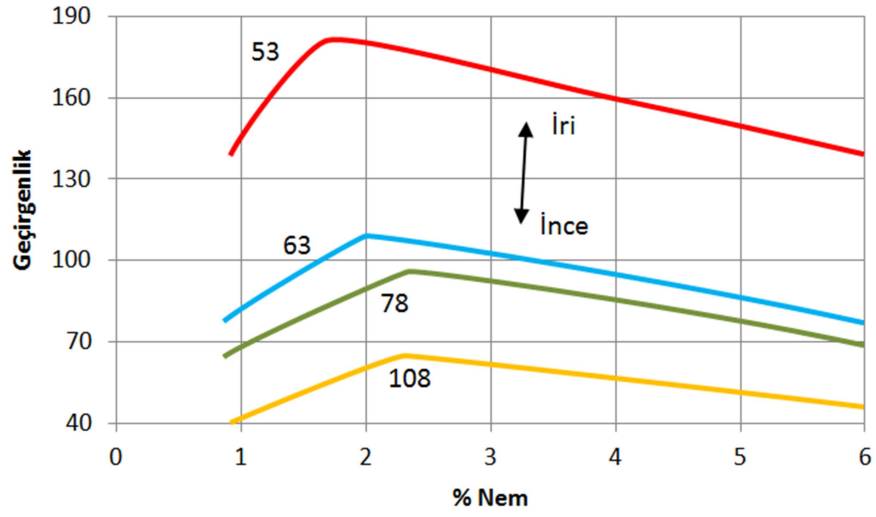
Şekil 2.33 Kum tane inceliği, nem oranı ve gaz geçirgenliği arasındaki ilişkinin grafik üzerinde gösterimi [6]
