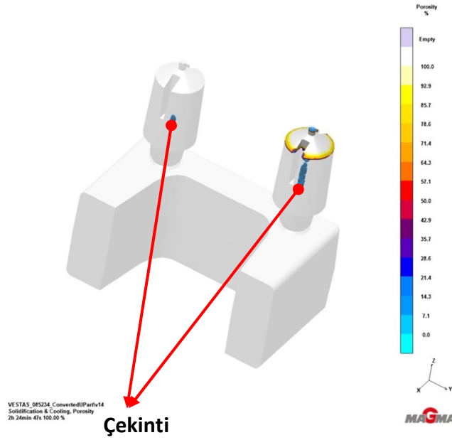
Şekil 2.59 Çekinti (shrinkage porosity) riskinin olduğu bölgelerin belirlenmesi
