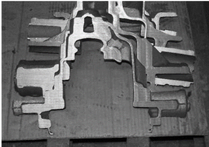
Şekil 6.69 Yeni yolluk ile dökülen parçanın kesit görüntüsü
