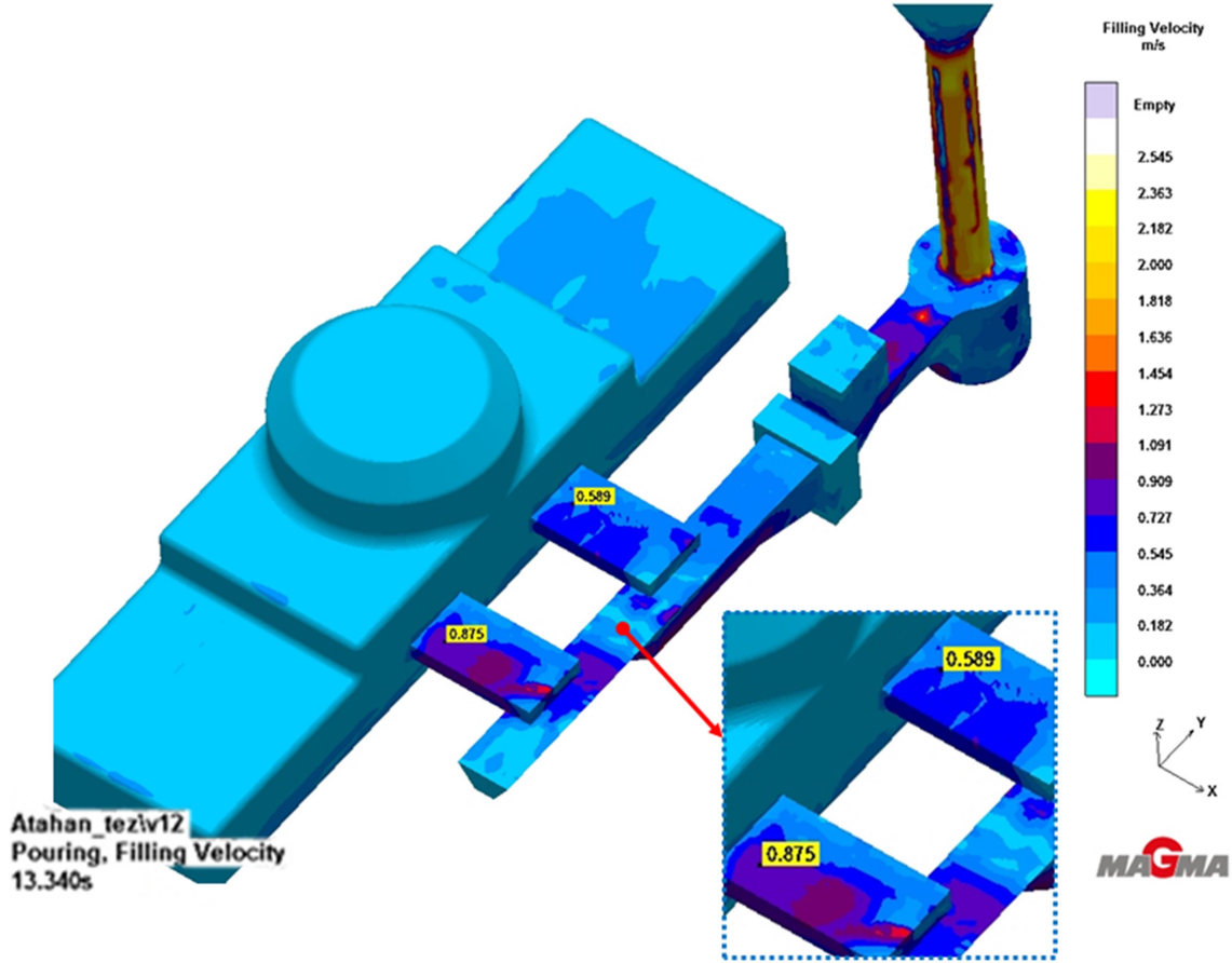
Şekil 5.16 Yolluk kesit alanı daraltılmış olan dizayn ( \varnothing 25 )
