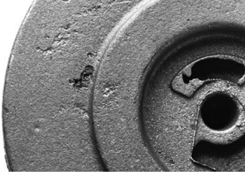
Şekil 4.2 Cüruf sakatı [23]
