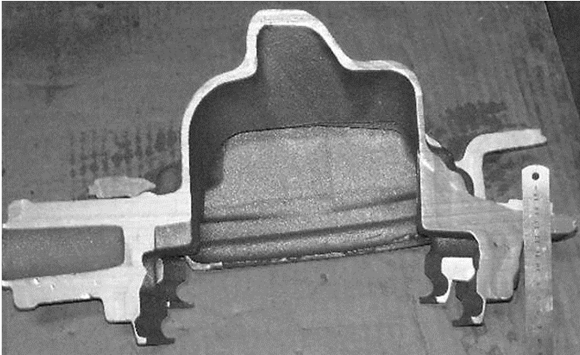
Şekil 6.66 Yeni yolluk ile dökülen parçanın kesit görüntüsü
