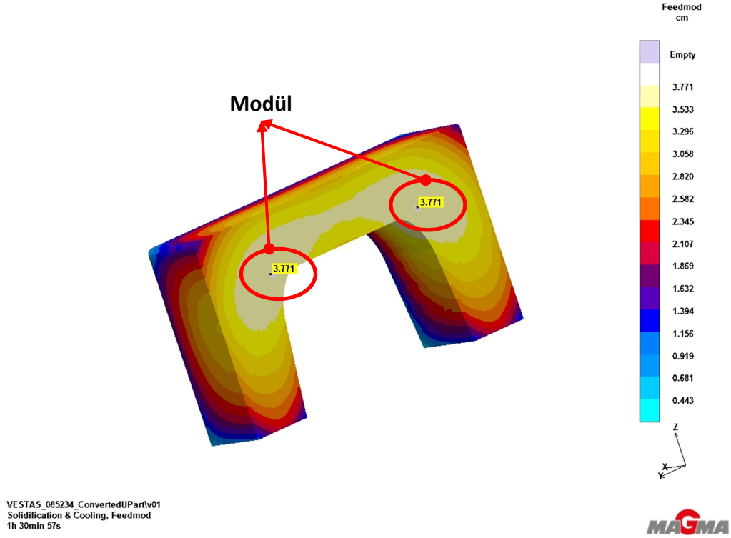
Şekil 2.56 sıcak bölgelerin modülünün belirlenmesi
