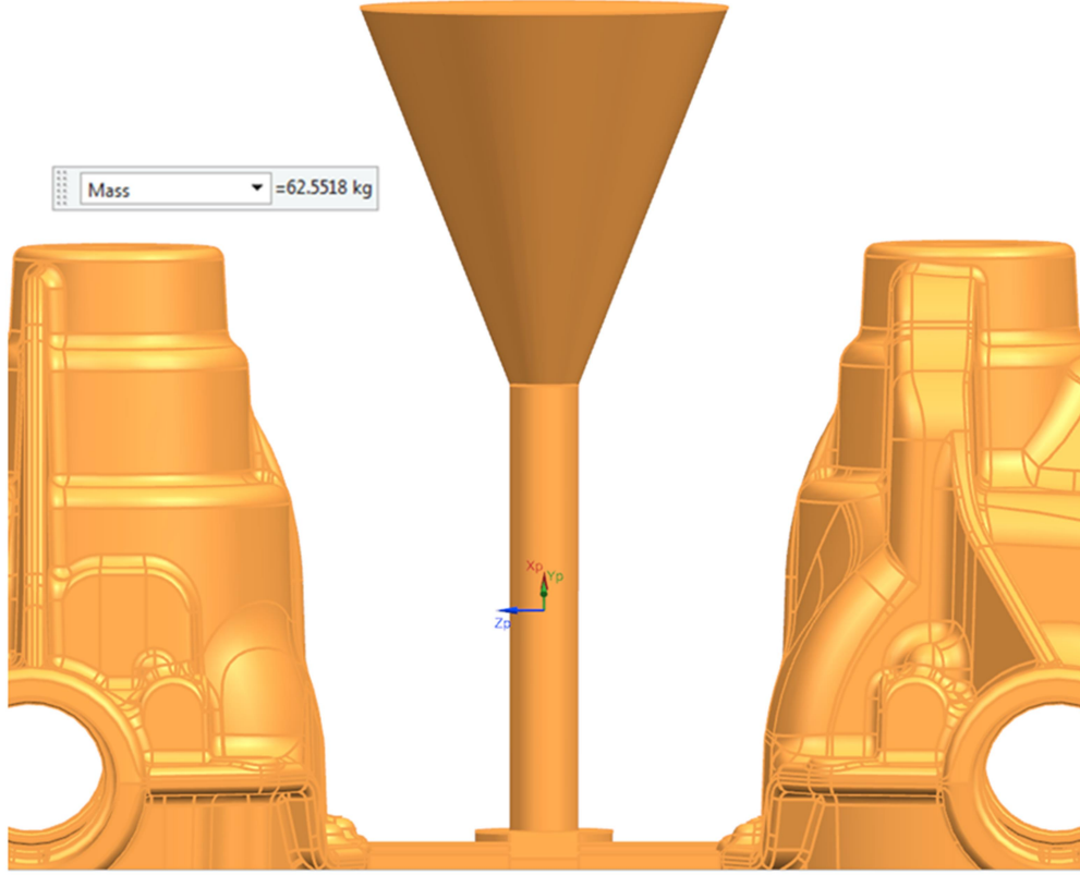
Şekil 6.7 Yaklaşık brüt ağırlığın data üzerinden hesabı
