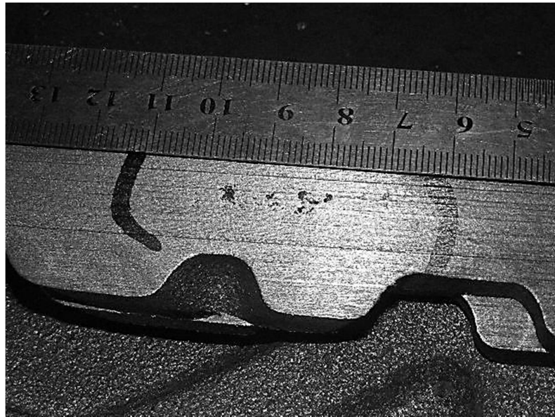
Şekil 2.50 Parça kesitinde gözlemlenen çekinti örneği
