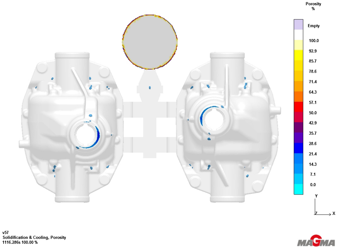
Şekil 6.28 Proje parçasının iç boşluk riski
