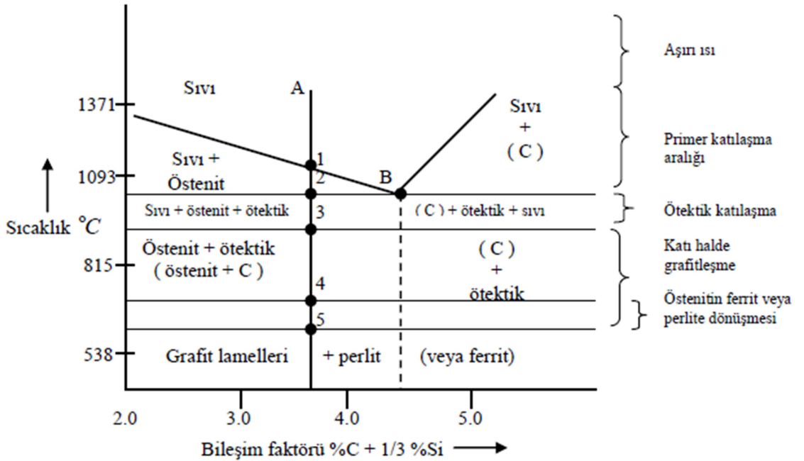
Şekil 3.6 Dökme demirlerde katılaşmanın ve grafit oluşumunun sıcaklık aralığının yaklaşık olarak gösterimi [6]
