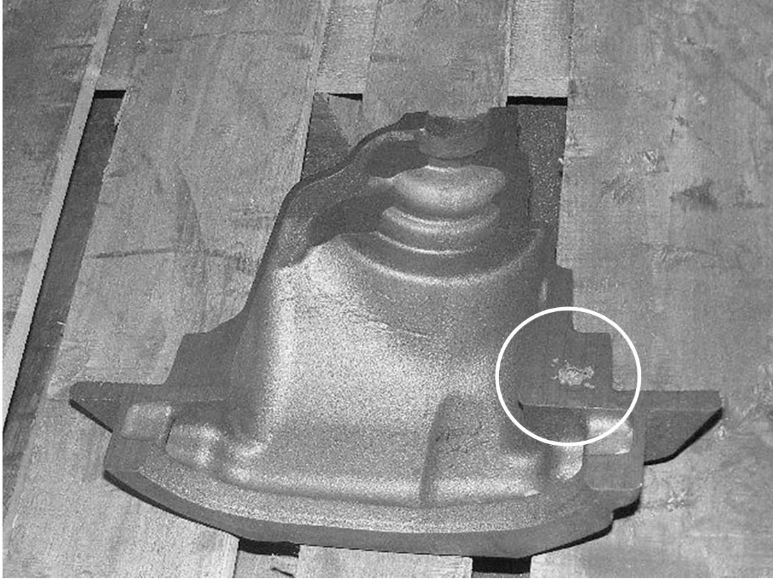
Şekil 6.43 Parçanın kesit görüntüsü ve çekinti
