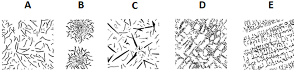
Şekil 3.1 Gri dökme demirlerin grafit türleri [27]
