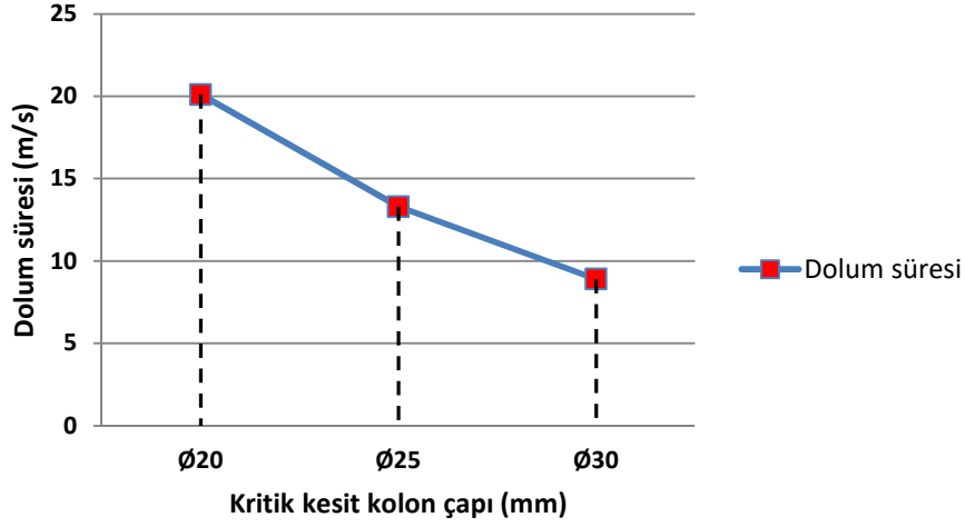
Şekil 5.21 Kritik kesit kolon çapının dolum süresi üzerine etkisi
