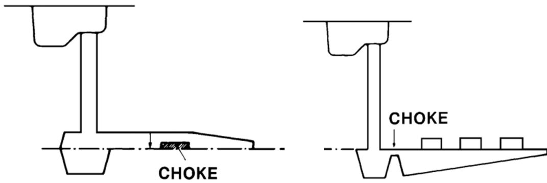
Şekil 5.1 Basıncılı ve basıncısız yolluk örneği [24]
