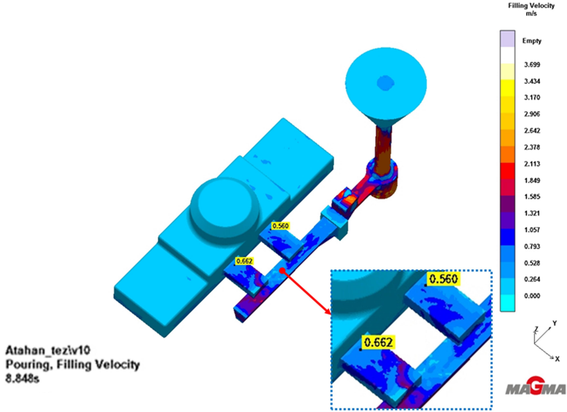
Şekil 5.14 Toplam meme giriş kesit alanının 2 kat arttırılması sonucu okunan hız değerleri
