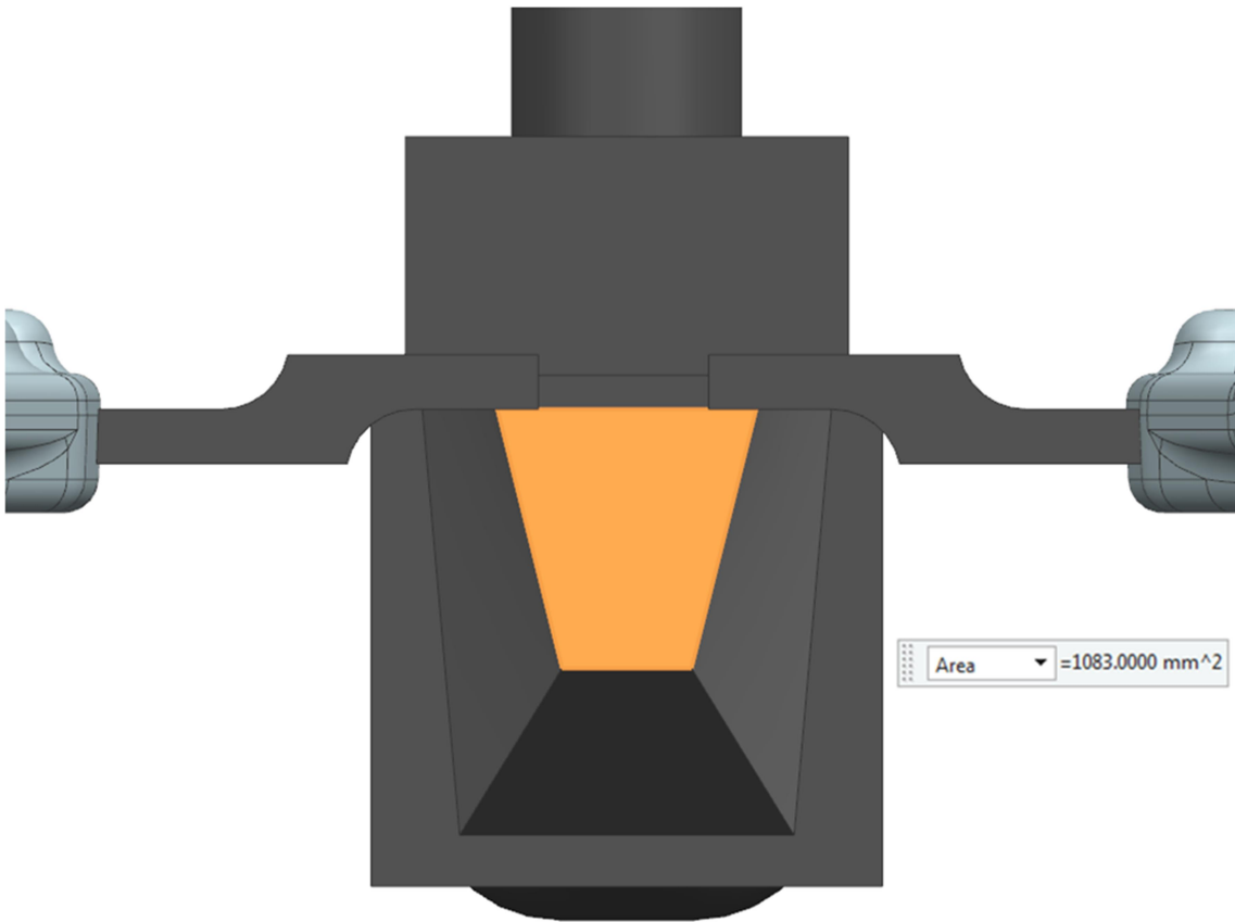
Şekil 6.11 Yatay yolluk kesit alanı
