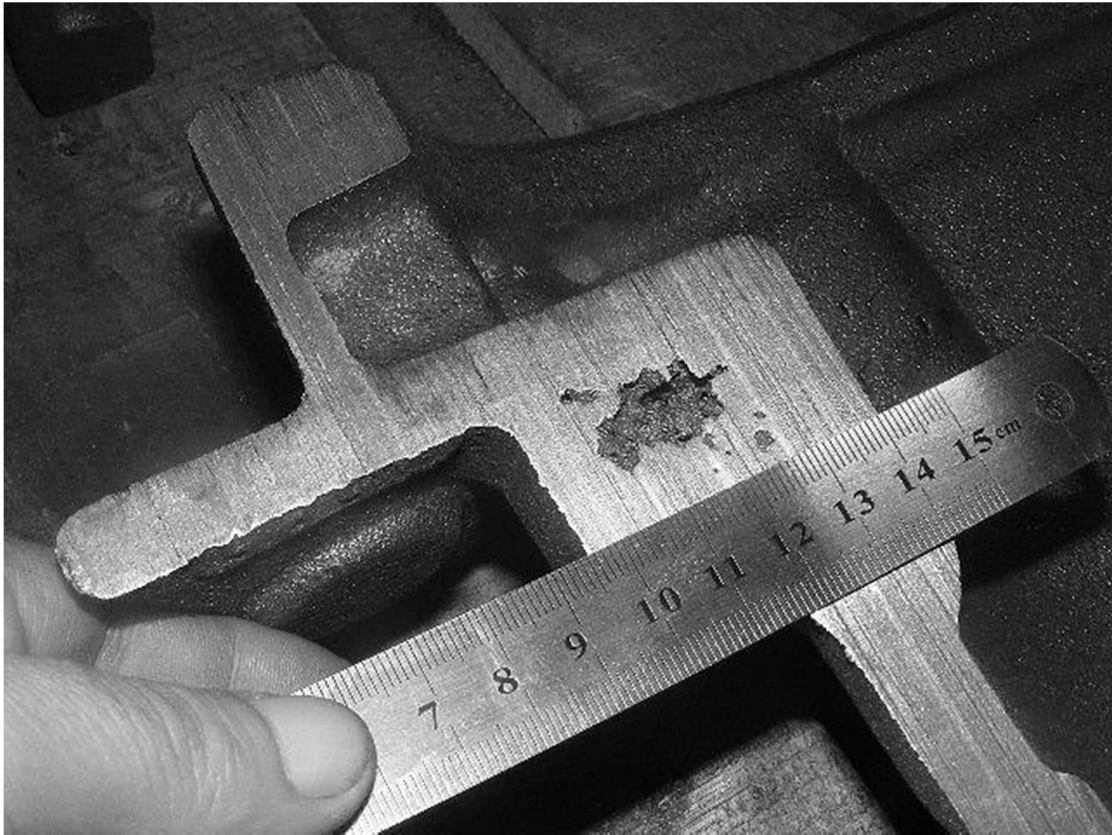
Şekil 6.44 Parçanın kesit görüntüsü ve çekinti
