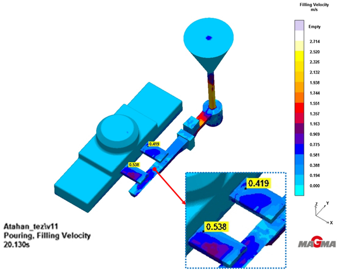
Şekil 5.17 Yolluk kesit alanı daraltılmış olan dizayn ( \varnothing 20 )
