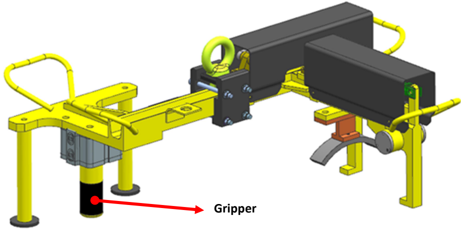
Şekil 2.26 Gripper maça aparatı
