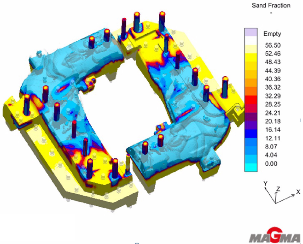
Şekil 2.16 Maça dolum simülasyonu 5
