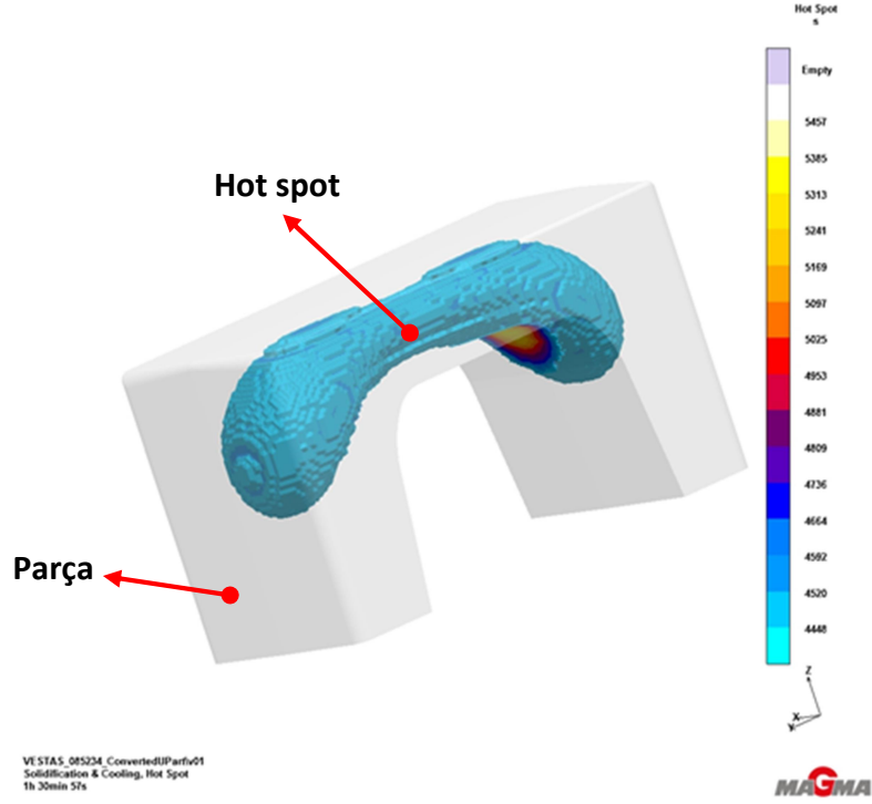
Şekil 2.55 Parçanın sıcak bölgelerinin belirlenmesi
