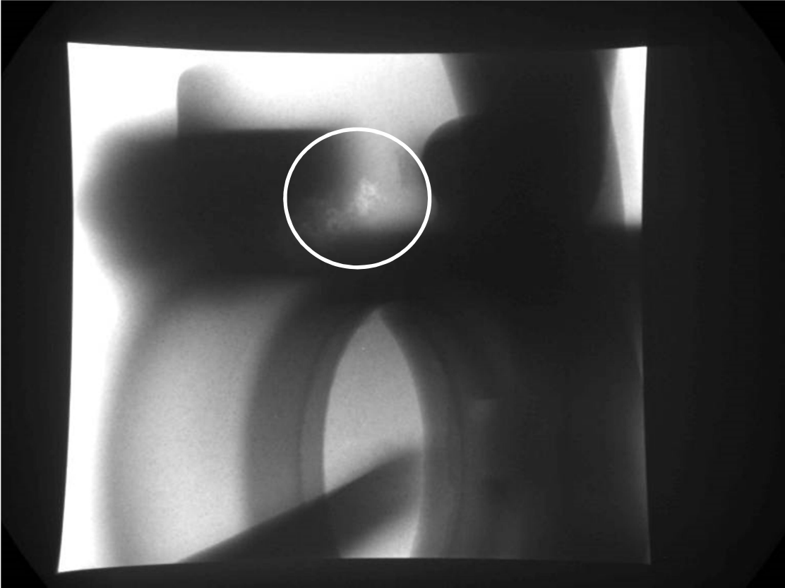
Şekil 6.38 X-ray görüntüsü ve çekinti
