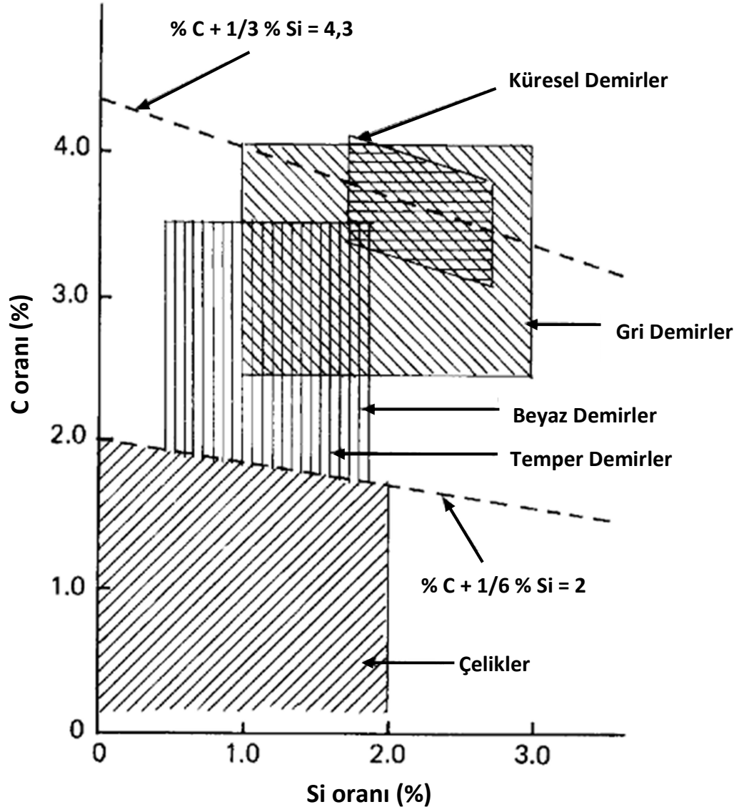
Şekil 3.5 Farklı dökme demirlerin ve çeliklerin C ve Si oranları [20]
