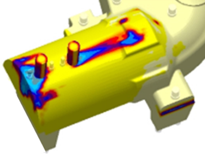
Şekil 2.17 Maça dolum simülasyonu 6
