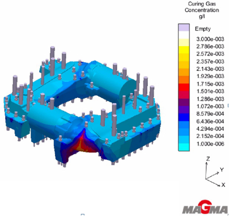
Şekil 2.20 Maça kürleme simülasyonu 2
