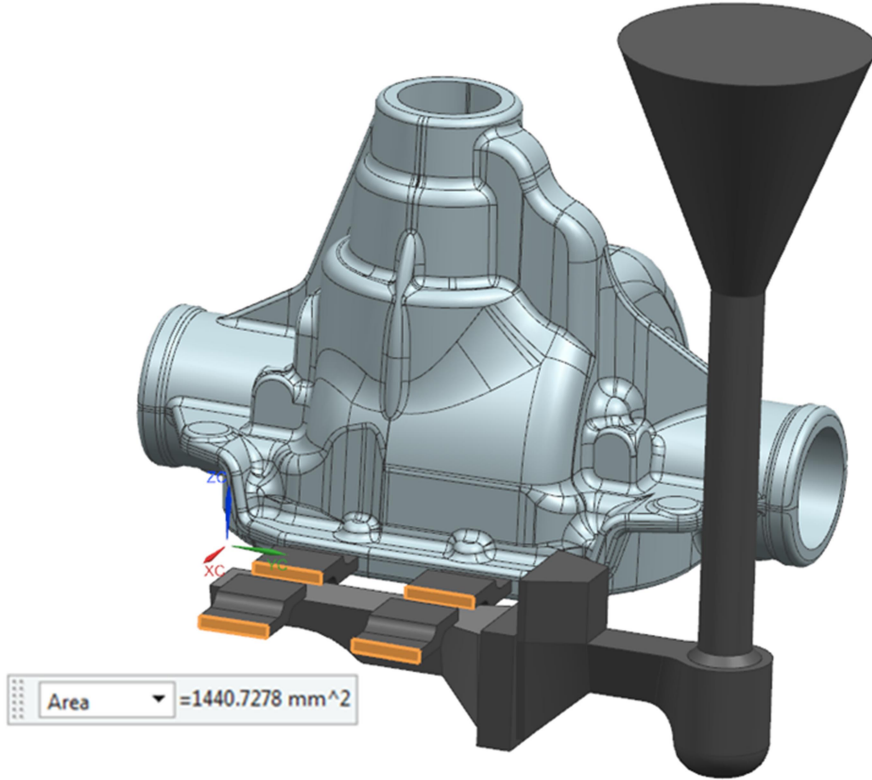
Şekil 6.15 Meme girişleri kesit alanları toplamı
