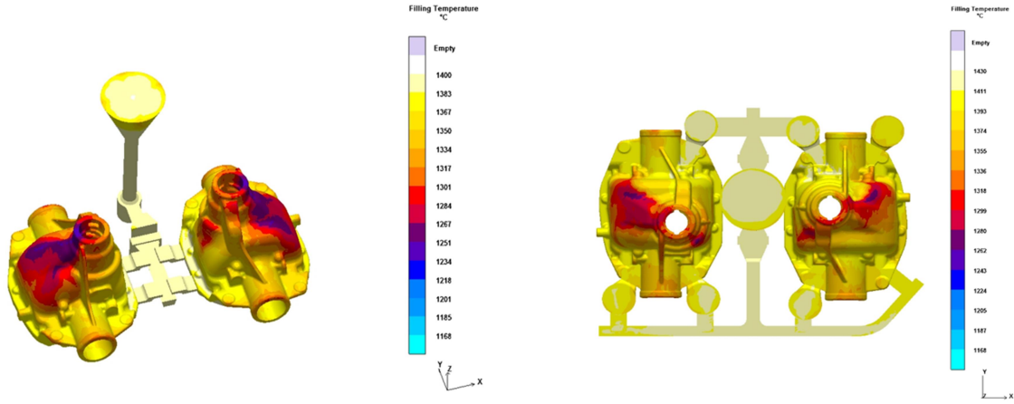
Şekil 6.55 Eski ve yeni sıcaklık dağılımı simülasyon sonuçlarının karşılaştırması
