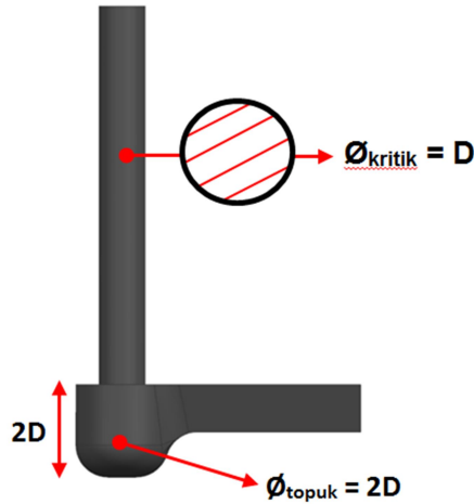
Şekil 5.8 Topuk ölçüsü değerleri
