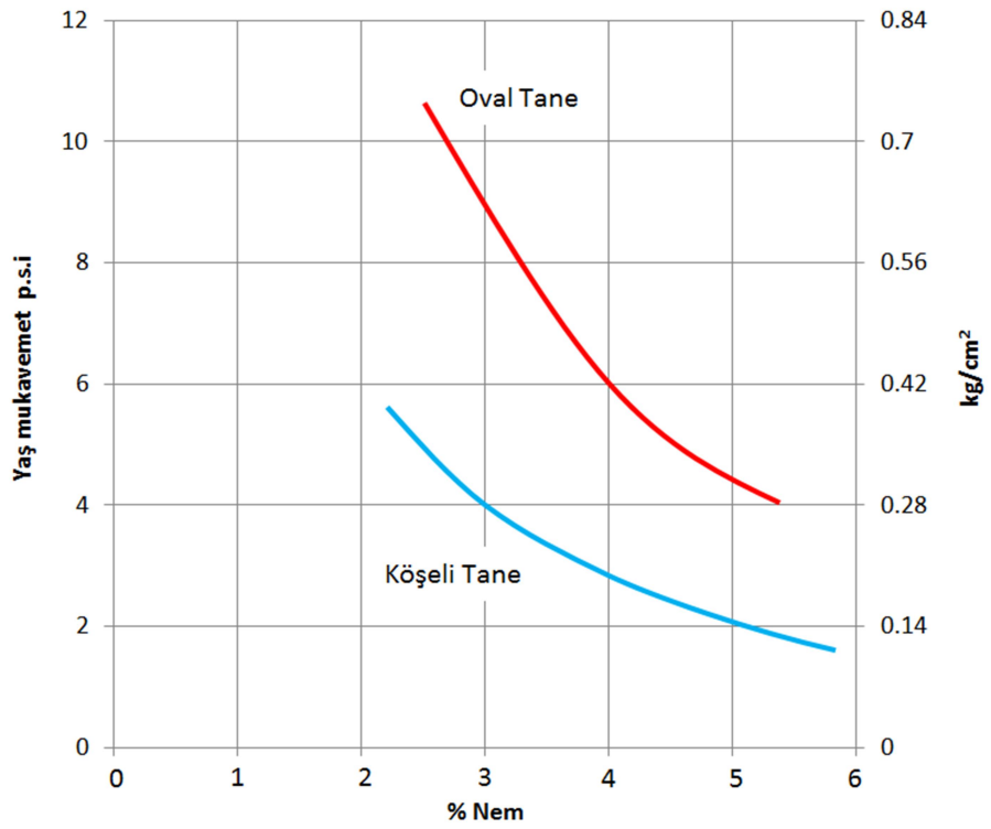
Şekil 2.32 Kum Şekli – Yaş Mukavemet grafiği [6]
