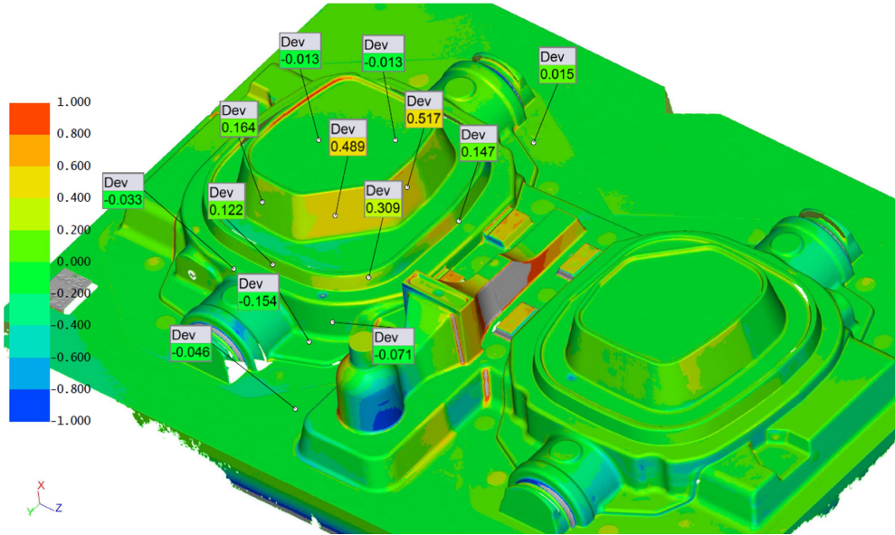
Şekil 6.30 Alt model ölçüsel tasarım raporu
