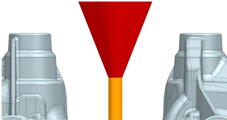
Şekil 6.6 Hat-3 havşası ile tahmini kolonun kesişimi
