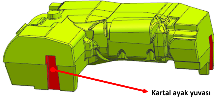
Şekil 2.25 Kartal ayak bölgelerinin gösterildiği maça dizaynı
