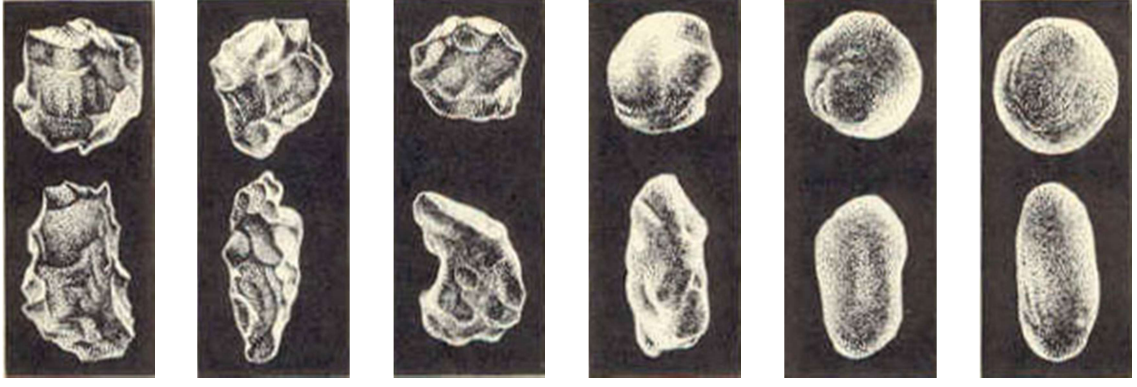
Şekil 2.40 Kum tanelerinin ayrıntılı sınıflandırılmış şekli [8]
