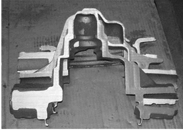
Şekil 6.68 Yeni yolluk ile dökülen parçanın kesit görüntüsü
