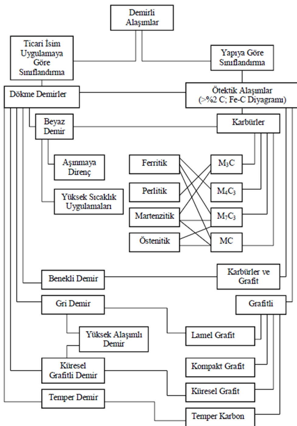
Şekil 3.4 Dökme demirler [17,18]
