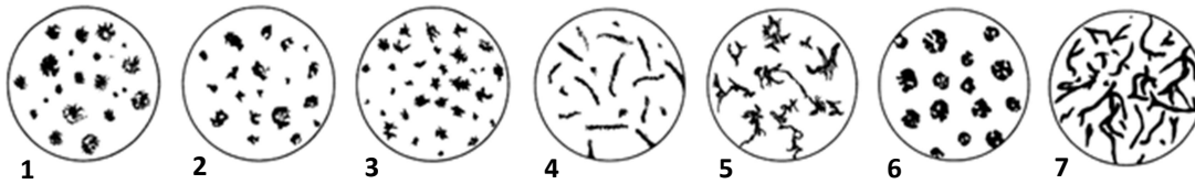
Şekil 3.2 Grafit şekilleri [27]
