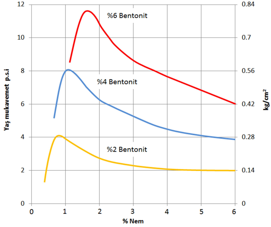
Şekil 2.31 Değişen bentonit miktarlarının nem oranına göre yaş mukavemet üzerindeki etkisi [6]
