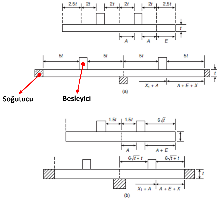
Şekil 2.53 Besleyici etkin mesafesinin hesaplanması. (a) Levha, genişlik : kalınlık > 5 : 1 ; (b) Çubuk, genişlik : kalınlık < 5 : 1 [11]
