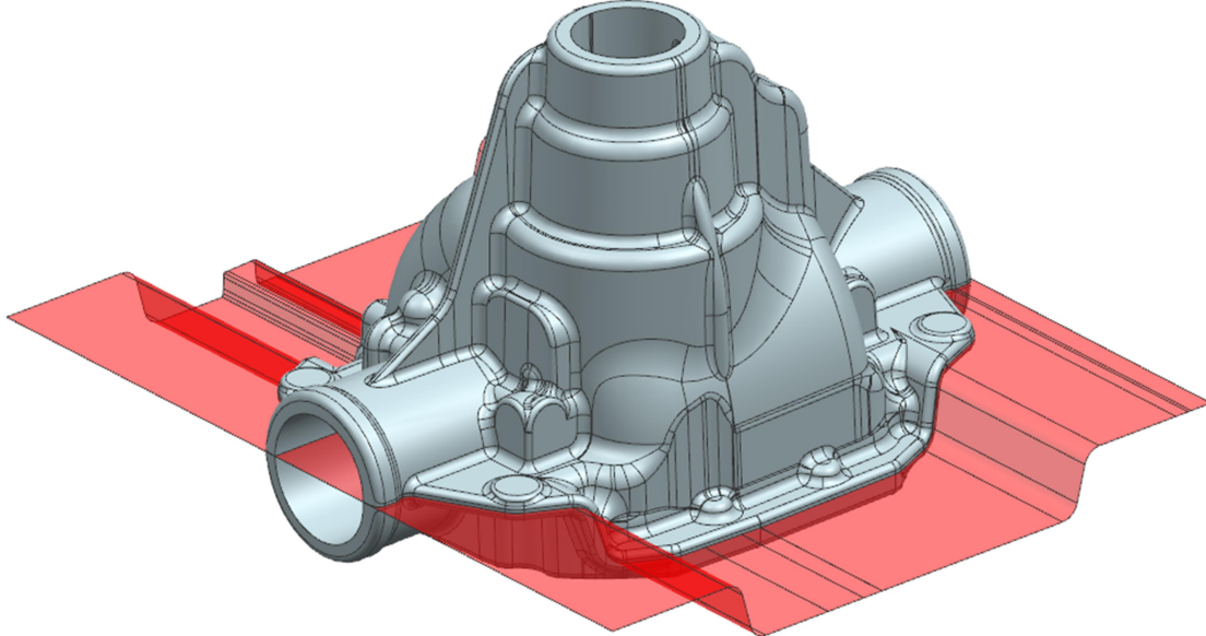
Şekil 6.8 Parçanın ayırım yüzeyi
