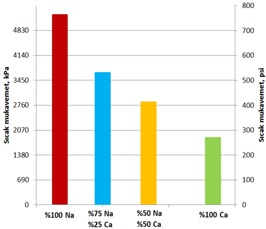
Şekil 2.43 Karıştırılmış Ca ve Na bentonitlerinin oranlarına göre sıcak mukavemet üzerindeki etkisi [2]
