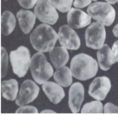
Şekil 2.36 İri taneli kum [7]
