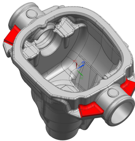
Şekil 6.52 Modifikasyon çalışması
