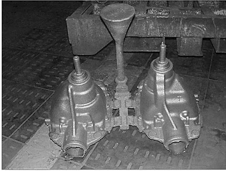
Şekil 6.31 Döküm sonrası yolluklu proje parçası
