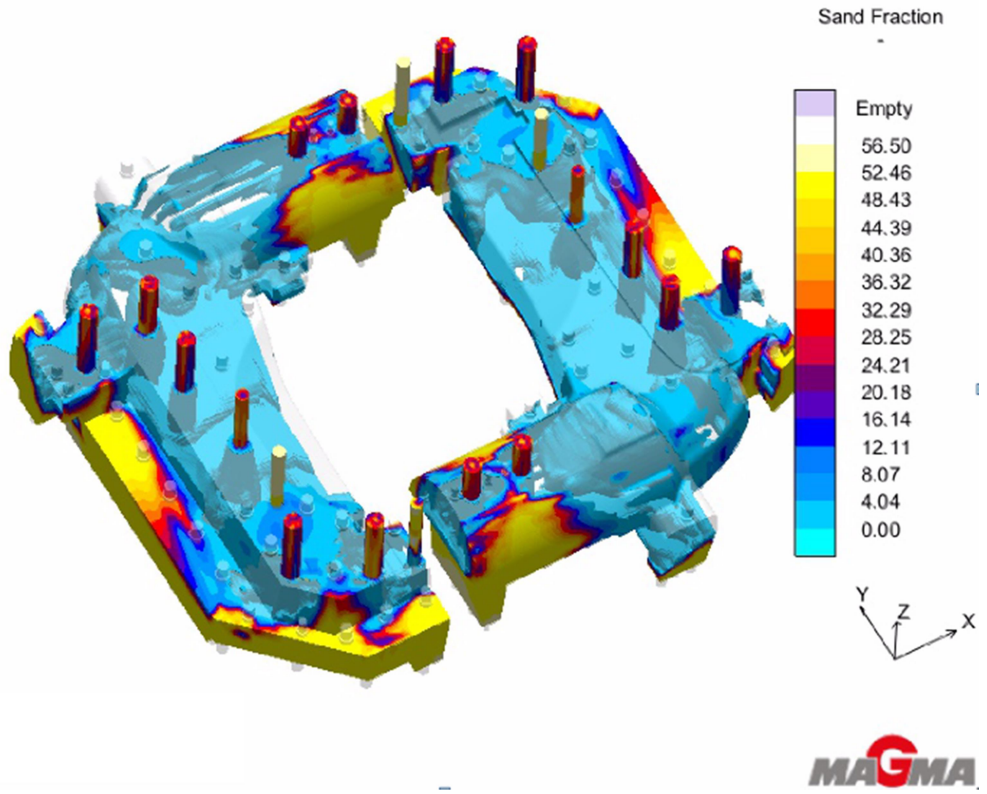
Şekil 2.15 Maça dolum simülasyonu 4
