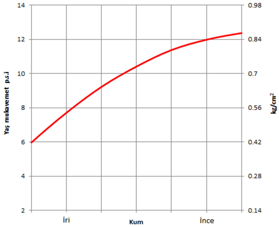
Şekil 2.29 Tane İnceliği – Yaş Mukavemet grafiği [6]
