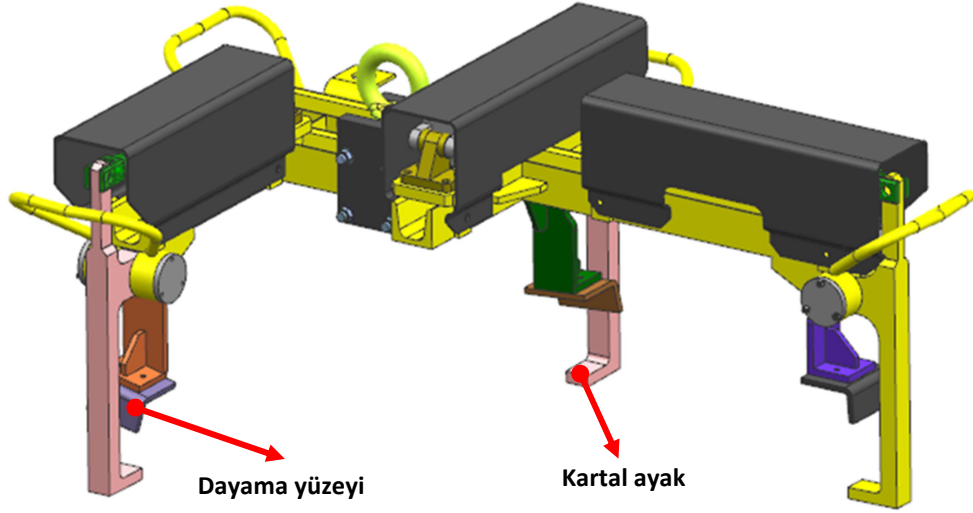
Şekil 2.24 Kartal ayak maça aparatı
