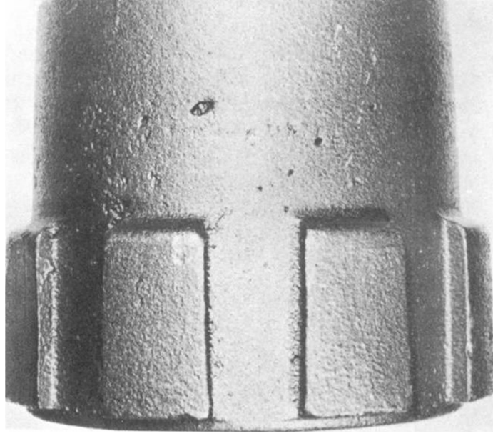
Şekil 4.1 Kum boşluğu [21,22]
