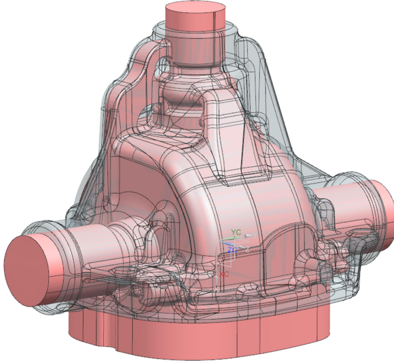
Şekil 6.23 Parça ve maçaların beraber görünümü
