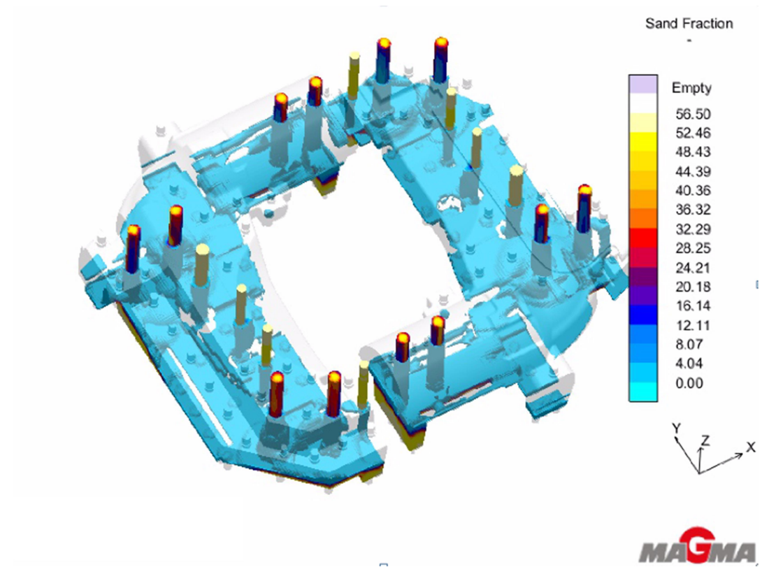
Şekil 2.14 Maça dolum simülasyonu 3
