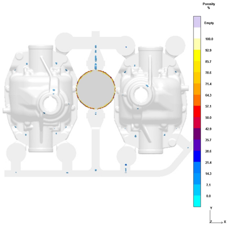
Şekil 6.54 Yeni dizayn ile iç boşluk riski
