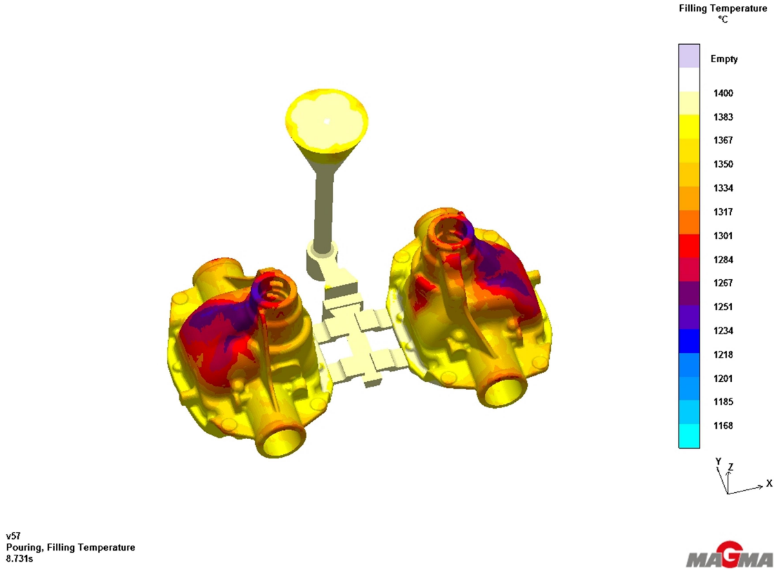
Şekil 6.25 Proje parçası sıcaklık dağılımı
