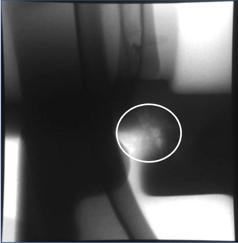
Şekil 6.62 Yeni yolluk ile dökülen parçanın x-ray kontrolleri
