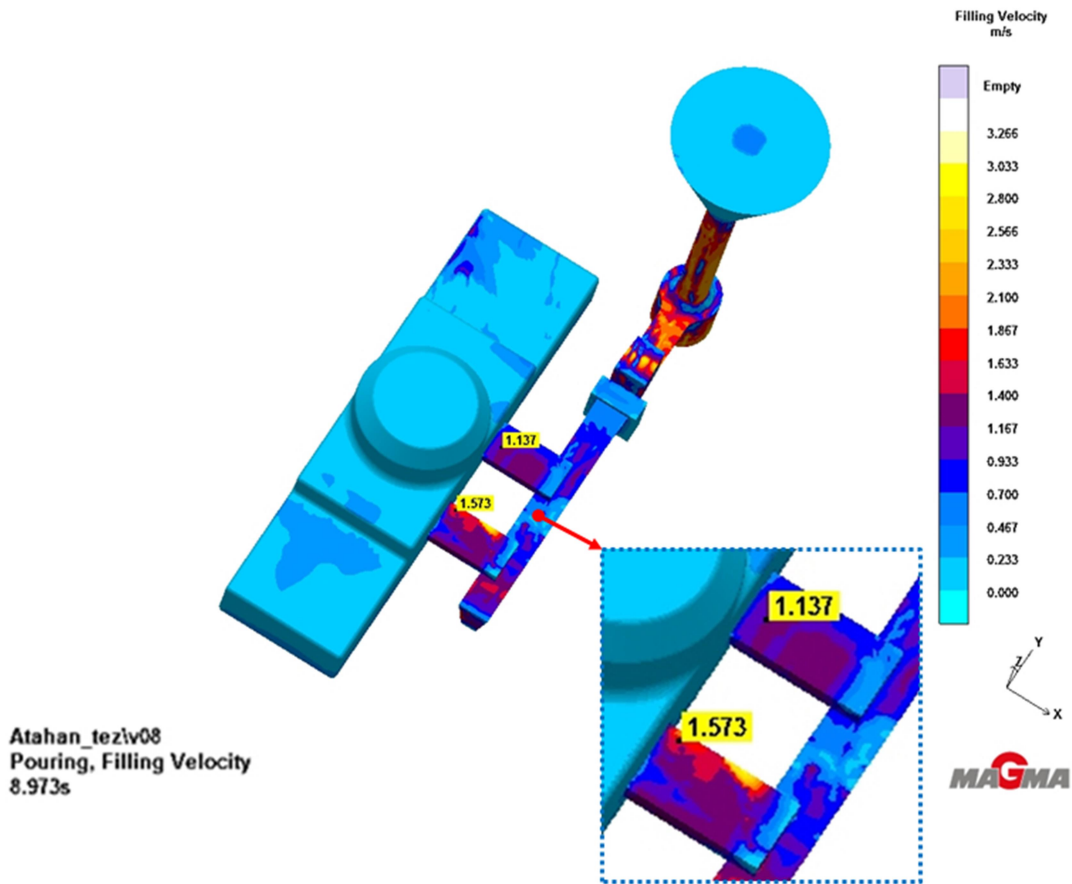
Şekil 5.15 Hesaplanan kesit alanları ile yapılan dizayn (Ø30)
