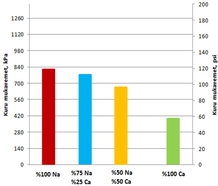
Şekil 2.42 Karıştırılmış Ca ve Na bentonitlerinin oranlarına göre kuru mukavemet üzerindeki etkisi [2]
