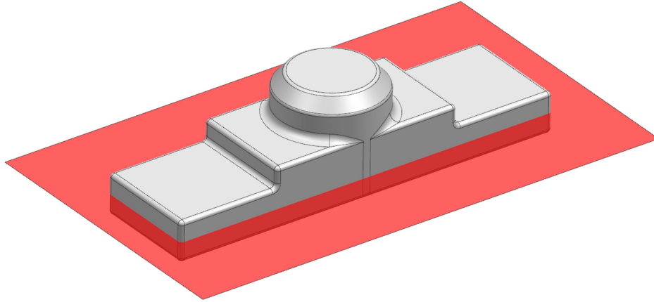
Şekil 5.10 Uygulama parçası ayırım yüzeyi
