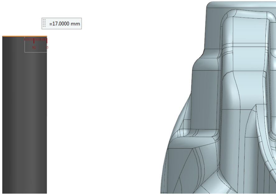
Şekil 6.10 Kolon kritik yarıçapı data ölçümü
