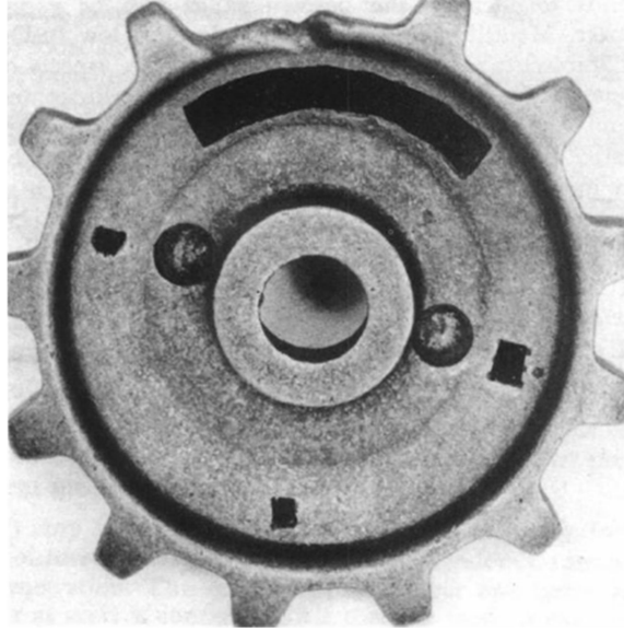
Şekil 4.5 Bir dişin olmadığı eksik döküm örneği [21,22]
