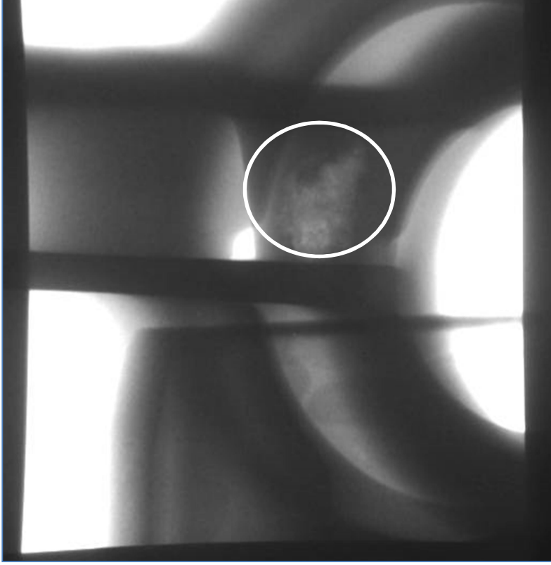
Şekil 6.61 Yeni yolluk ile dökülen parçanın x-ray kontrolleri
