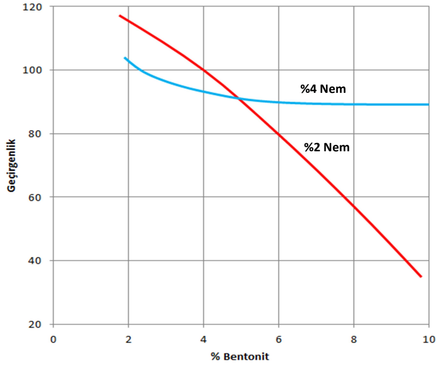
Şekil 2.35 Bentonit oranı, nem ve geçirgenlik arasındaki ilişkinin grafiği [6]
