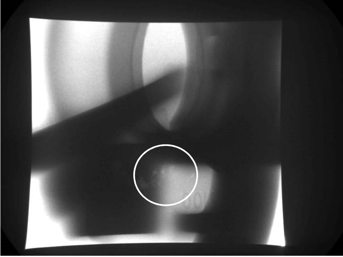
Şekil 6.37 X-ray görüntüsü ve çekinti
