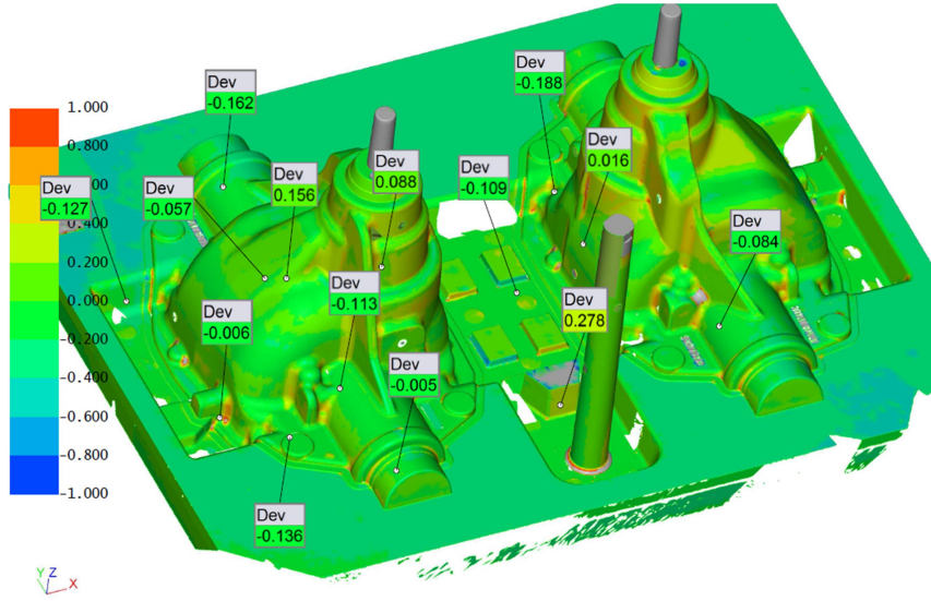
Şekil 6.29 Üst model ölçüsel tarama raporu
