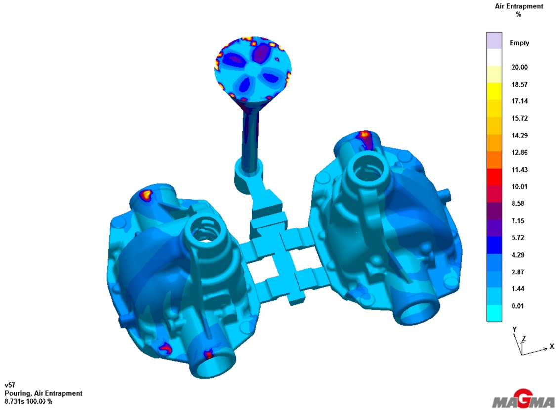
Şekil 6.27 Proje parçasının hava sıkışması
