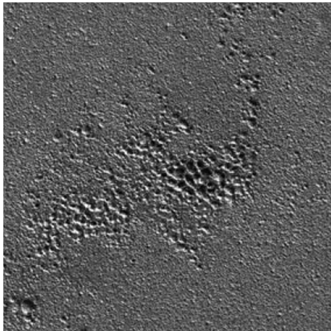
Şekil 4.4 Karınca (pinhole) sakatı [23]
