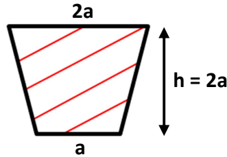
Şekil 5.6 Yatay yolluk kesidi örneği
