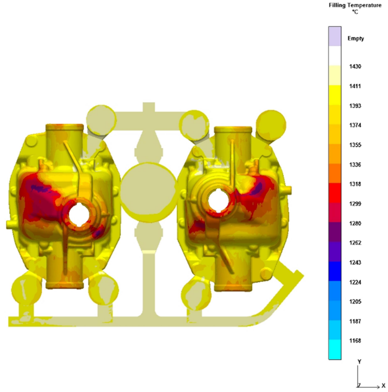
Şekil 6.53 Yeni dizayn ile sıcaklık dağılımı
