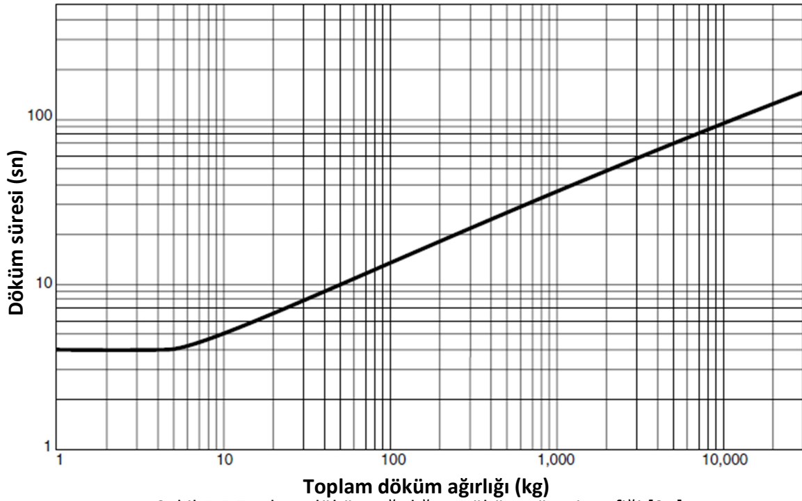
Şekil 5.5 Toplam döküm ağırlığı – Döküm süresi grafiği [24]
