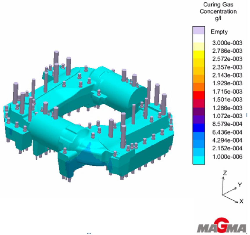
Şekil 2.22 Maça kürlleme simülasyonu 4
