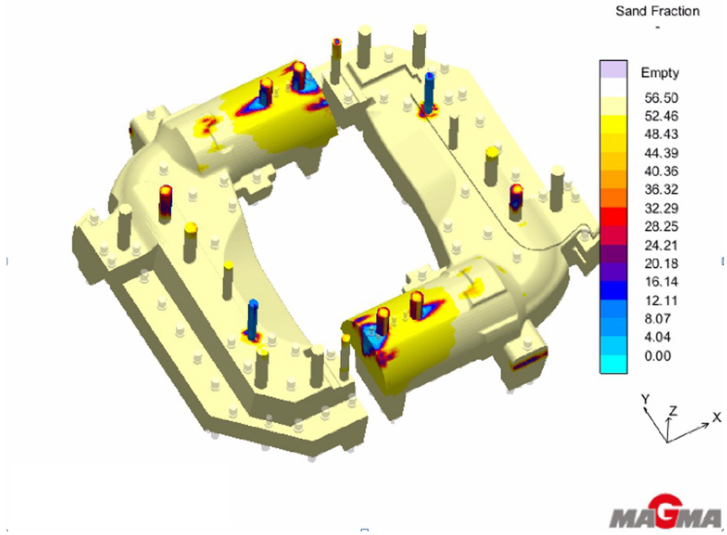
Şekil 2.17 Maça dolum simülasyonu 6
