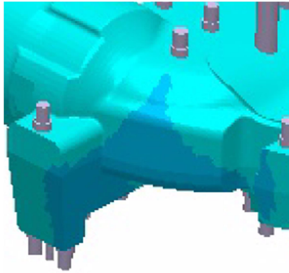
Şekil 2.23 Maça kürlleme simülasyonu sonucu risk teşkil eden bölge
