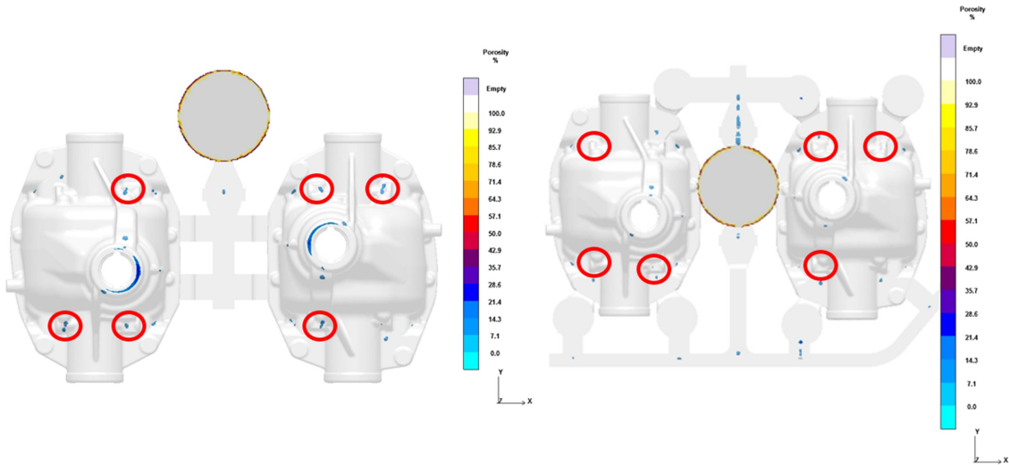
Şekil 6.56 Eski ve yeni çekinti riskinin gösterildiği simülasyon sonuçlarının karşılaştırması
