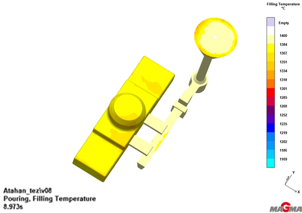
Şekil 5.18 \varnothing 30 mm – 8,9 sn dolum süresi sıcaklık dağılımı
