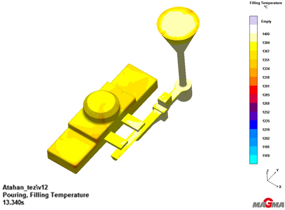
Şekil 5.19 Ø25 mm – 13,3 sn dolum süresi sıcaklık dağılımı
