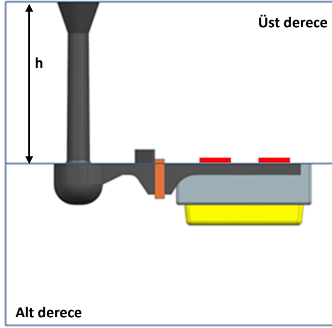
Şekil 5.3 Parçanın tümüyle alt derecede olduğu durum
