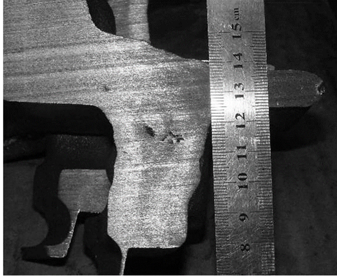
Şekil 6.67 Yeni yolluk ile dökülen parçanın kesit görüntüsü
