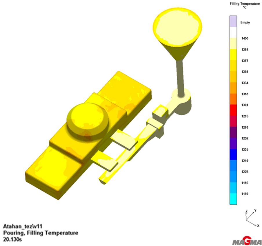
Şekil 5.20 Ø20 mm – 20,1 sn dolum süresi sıcaklık dağılımı
