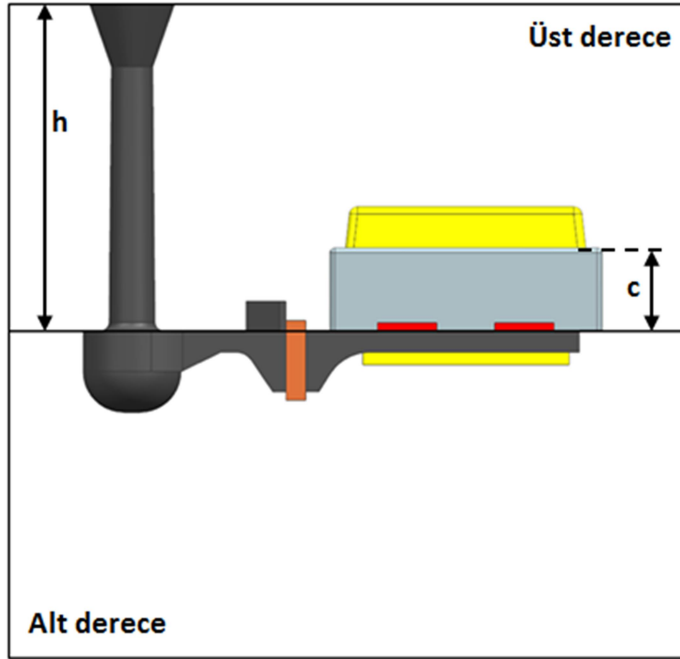
Şekil 5.4 Parçanın tümüyle üst derecede olduğu durum
