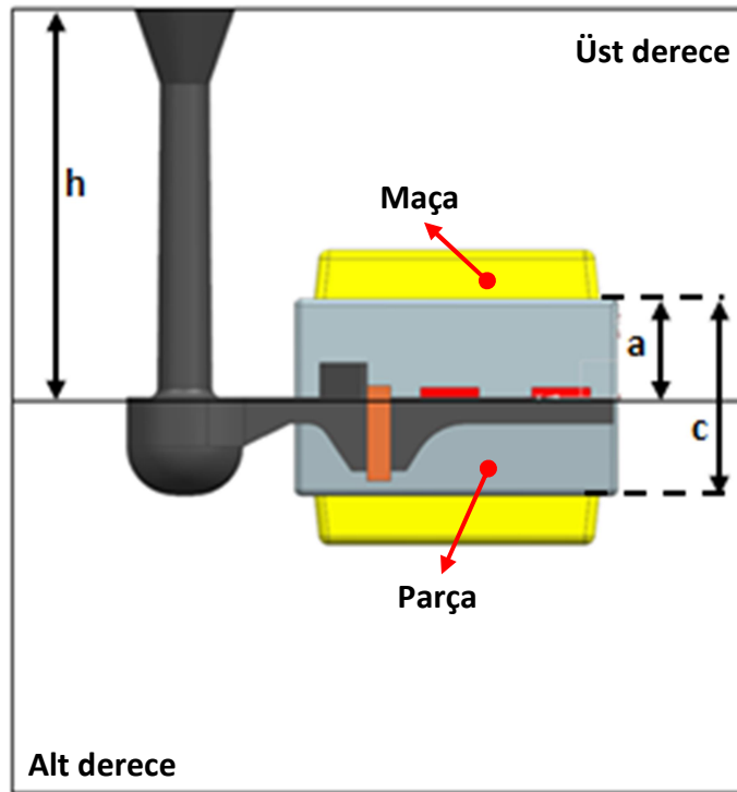
řekil 5.2 Parçanın hem alt hem de üst derecede olduęu durum
