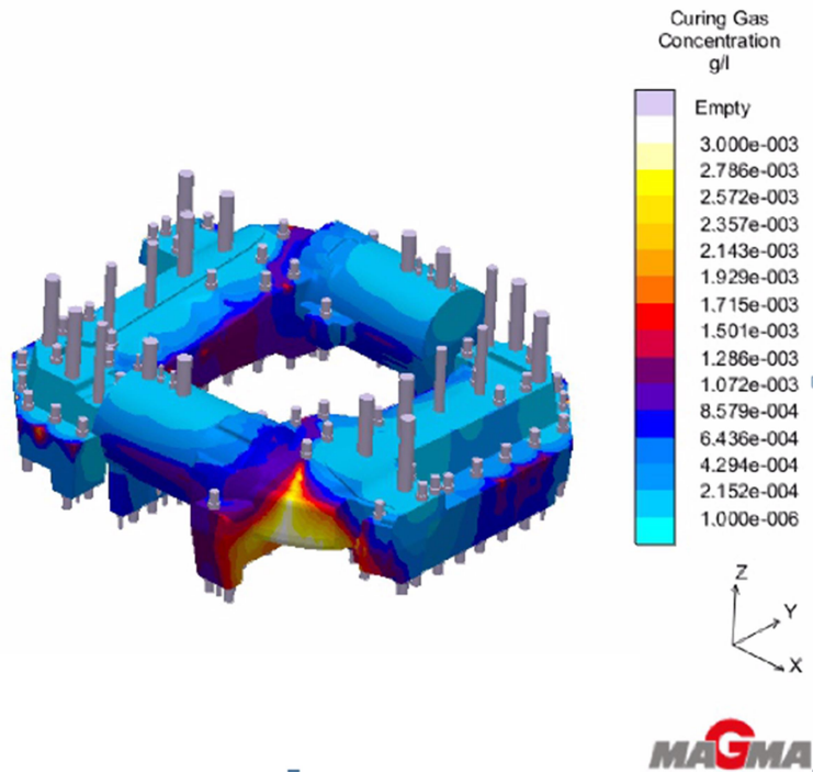
Şekil 2.19 Maça kürleme simülasyonu 1
