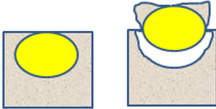
Şekil 2.3 Ters açıda kalan yüzeylerin olduğu model ile kalıplama
