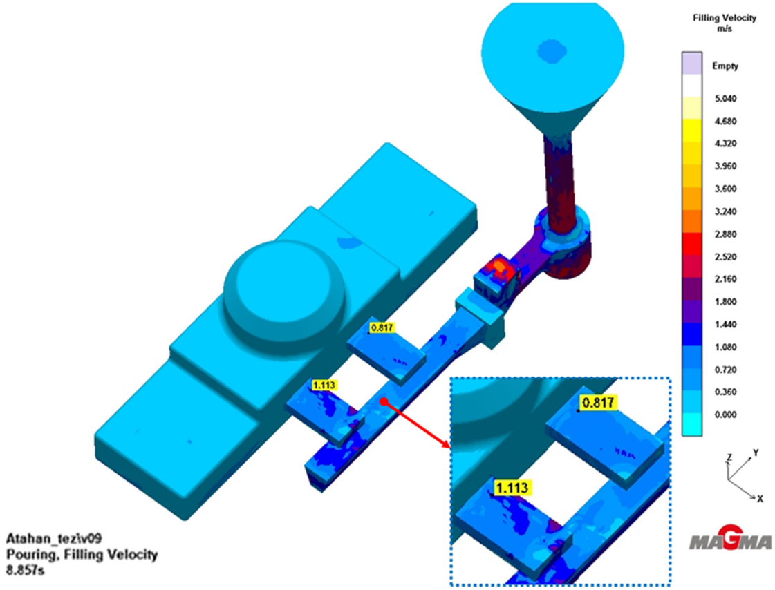
Şekil 5.13 Toplam meme giriş kesit alanının 1,5 kat arttırılması sonucu okunan hız değerleri
