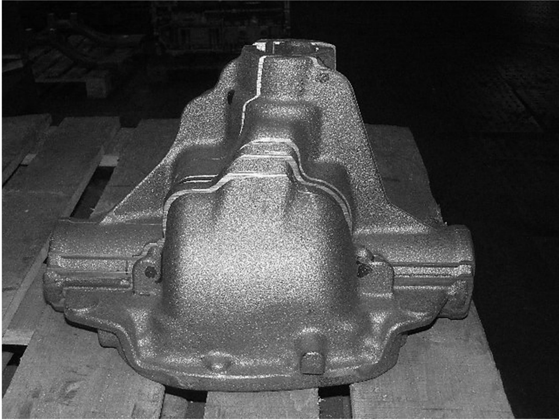
Şekil 6.42 X-ray sonucunda tespit edilen çekinti bölgeleri
