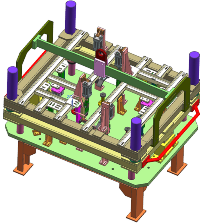
Şekil 2.28 Merkezlemeli aparat
