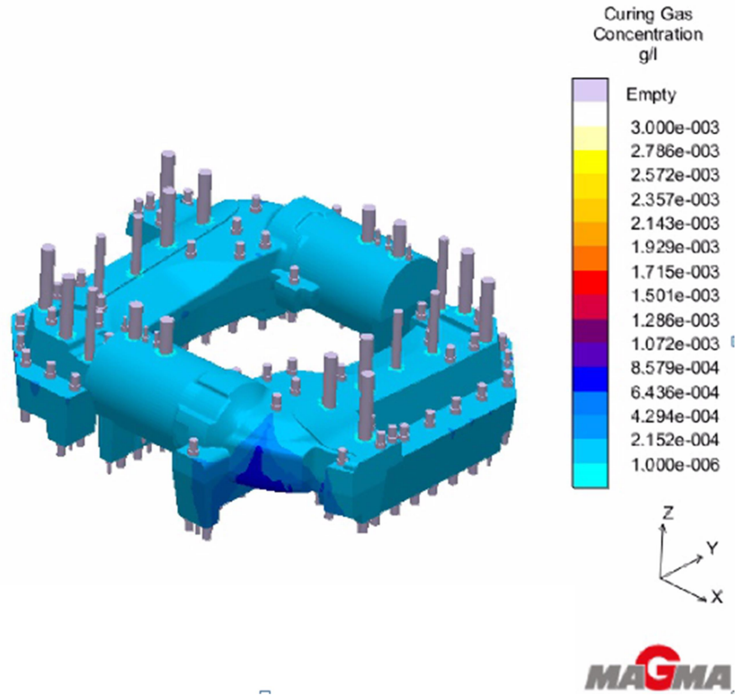
Şekil 2.21 Maça kürleme simülasyonu 3
