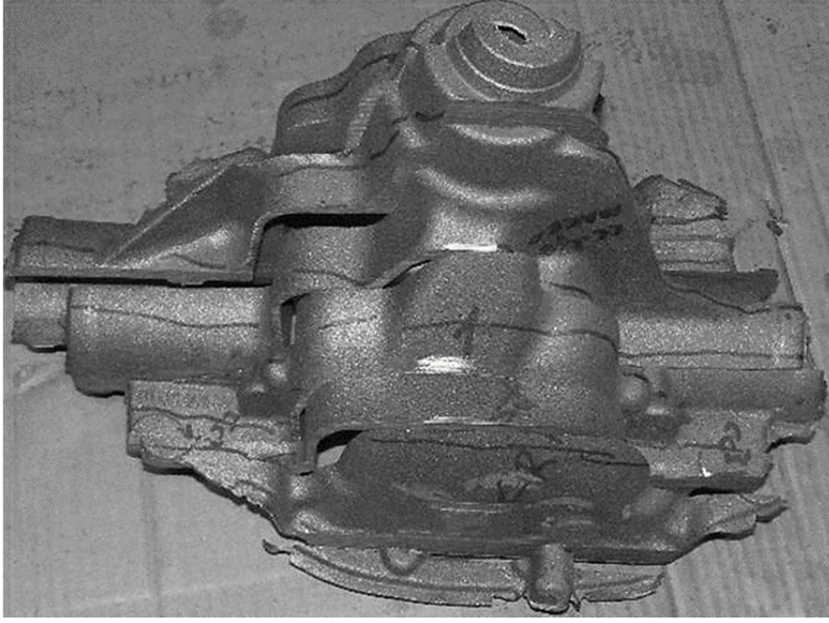
Şekil 6.65 Yeni yolluk ile dökülen parçanın dilimlenmesi
