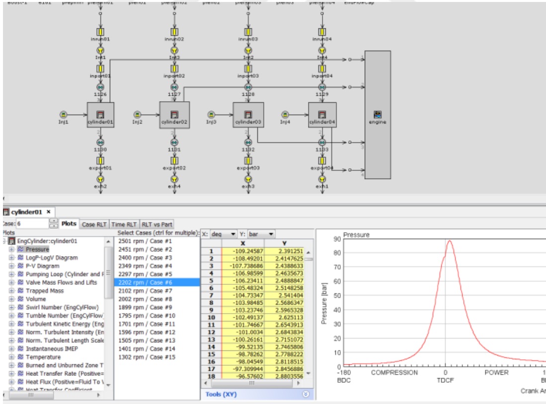
Şekil 3.1 Kıyaslama için kurulan GT-Power analiz modeli
