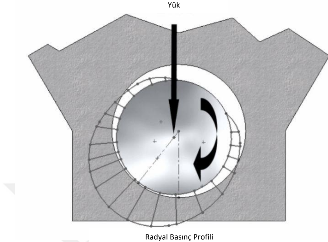
Şekil 2.6 Krank miline gelen kuvvetler
