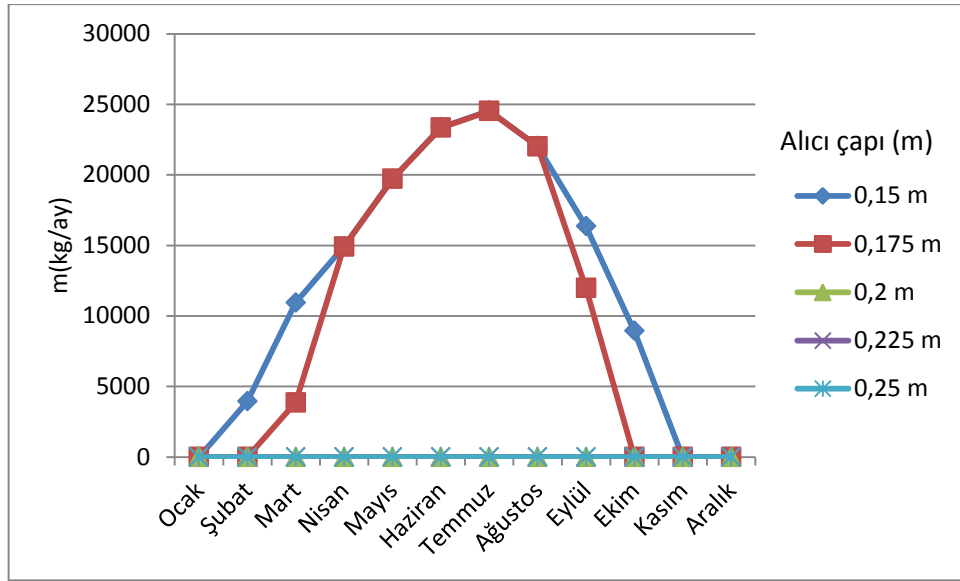
Şekil 4.14 Antalya'da Çanak çapı 10 m için aylara göre eriyen Al miktarı
