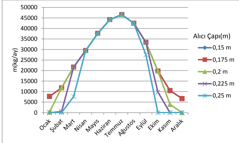
Şekil 4. 33 Mersin’de Çanak çapı 14 m için aylara göre eriyen Al miktarı
