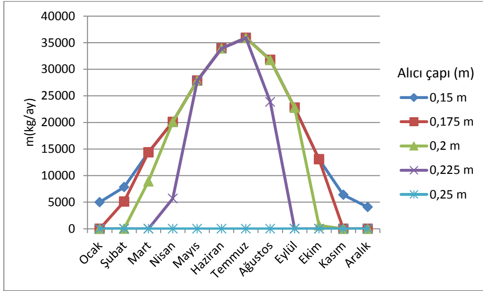
Şekil 4. 26 İzmir’de Çanak çapı 12 m için aylara göre eriyen Al miktarı
