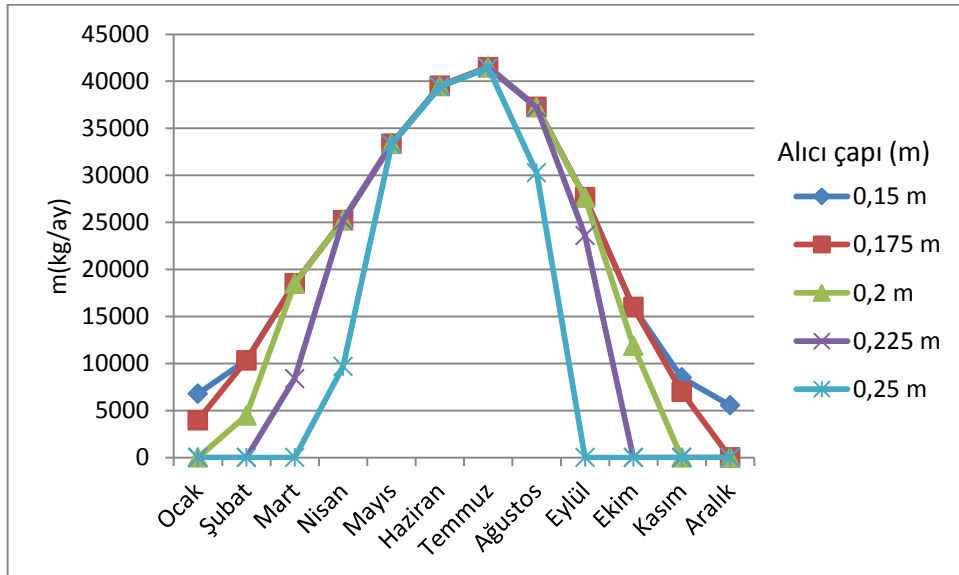
Şekil 4.17 Antalya'da Çanak çapı 13 m için aylara göre eriyen Al miktarı
