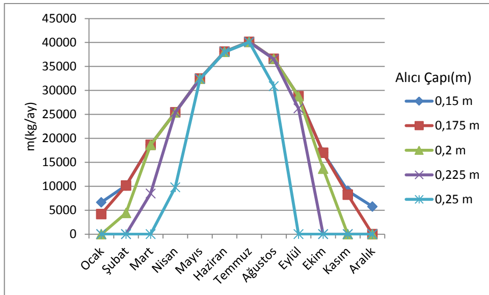
Şekil 4. 32 Mersin'de Çanak çapı 13 m için aylara göre eriyen Al miktarı
