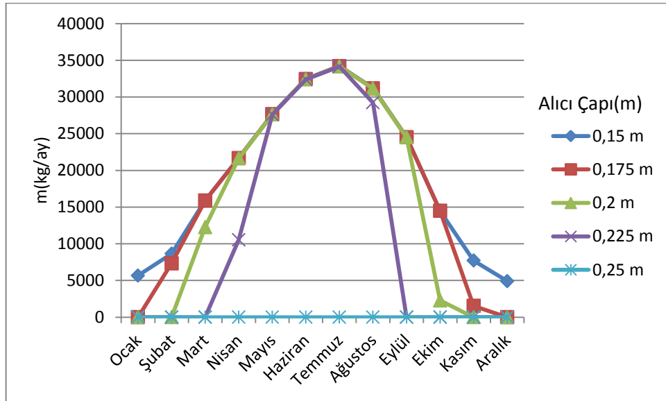
Şekil 4. 31 Mersin'de Çanak çapı 12 m için aylara göre eriyen Al miktarı
