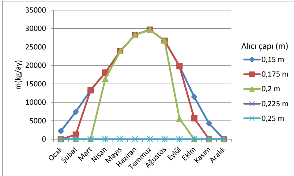
Şekil 4.15 Antalya'da Çanak çapı 11 m için aylara göre eriyen Al miktarı
