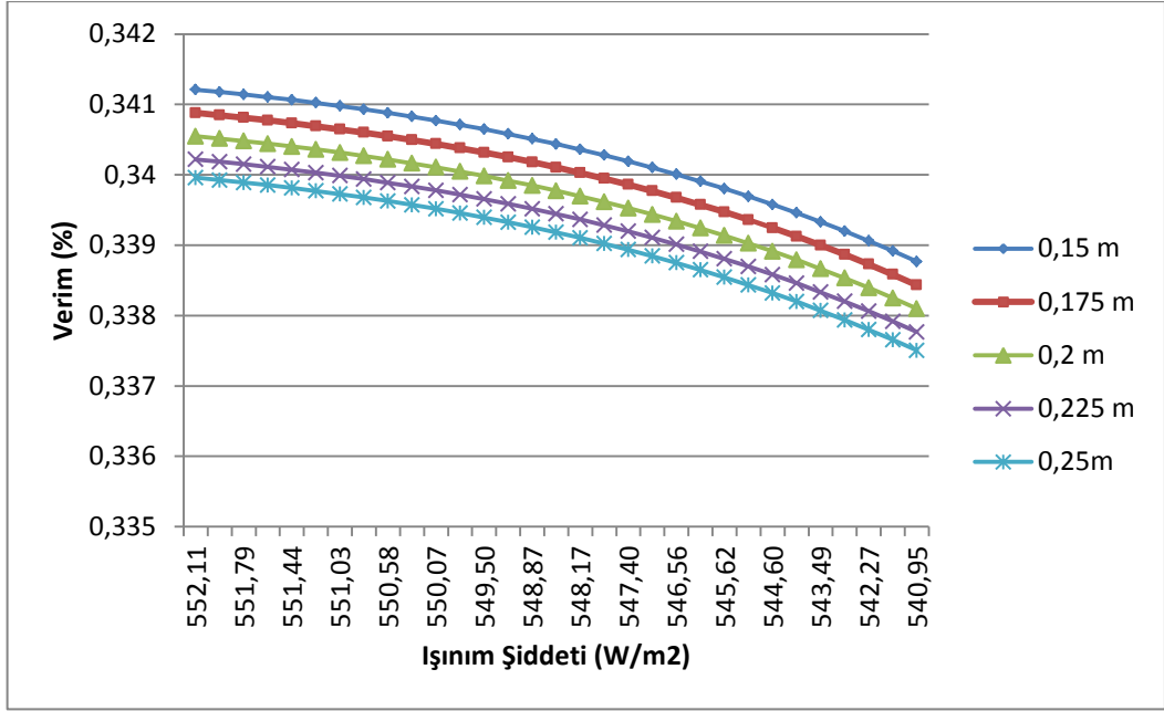
Şekil 4. 34 Antalya için (10 m) Alıcı çaplarında verim karşılaştırması
