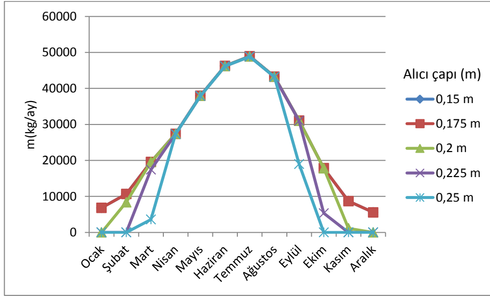
Şekil 4. 28 İzmir’de Çanak çapı 14 m için aylara göre eriyen Al miktarı
