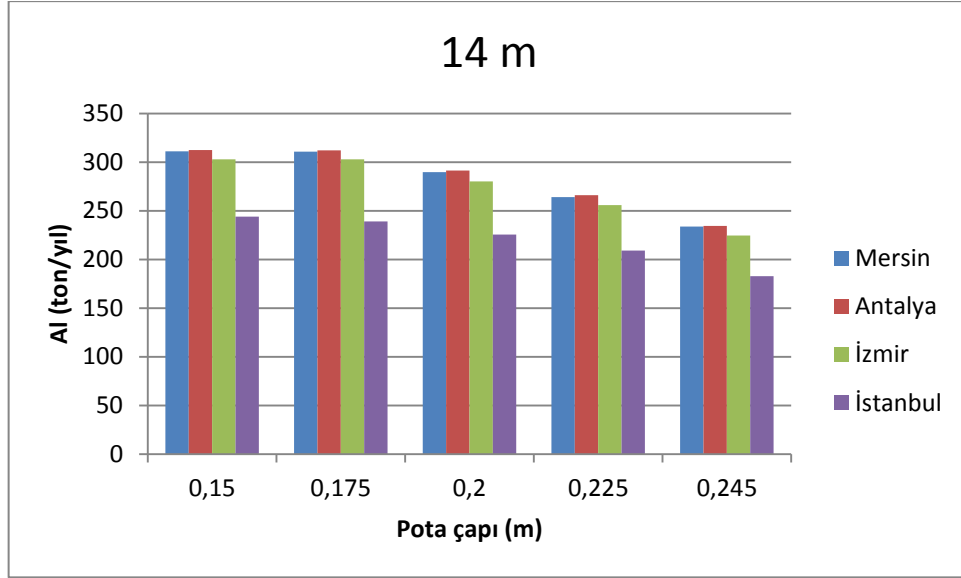
Şekil 4. 11 14 m'lik çanak çapı için 4 şehrin Al miktarı karşılaştırması
