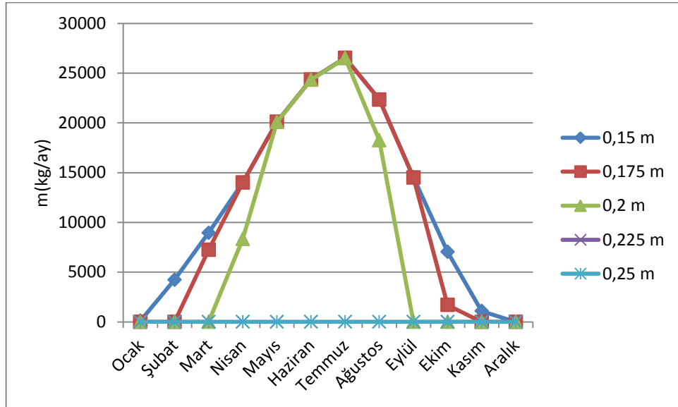
Şekil 4. 20 İstanbul'da Çanak çapı 11 m için aylara göre eriyen Al miktarı
