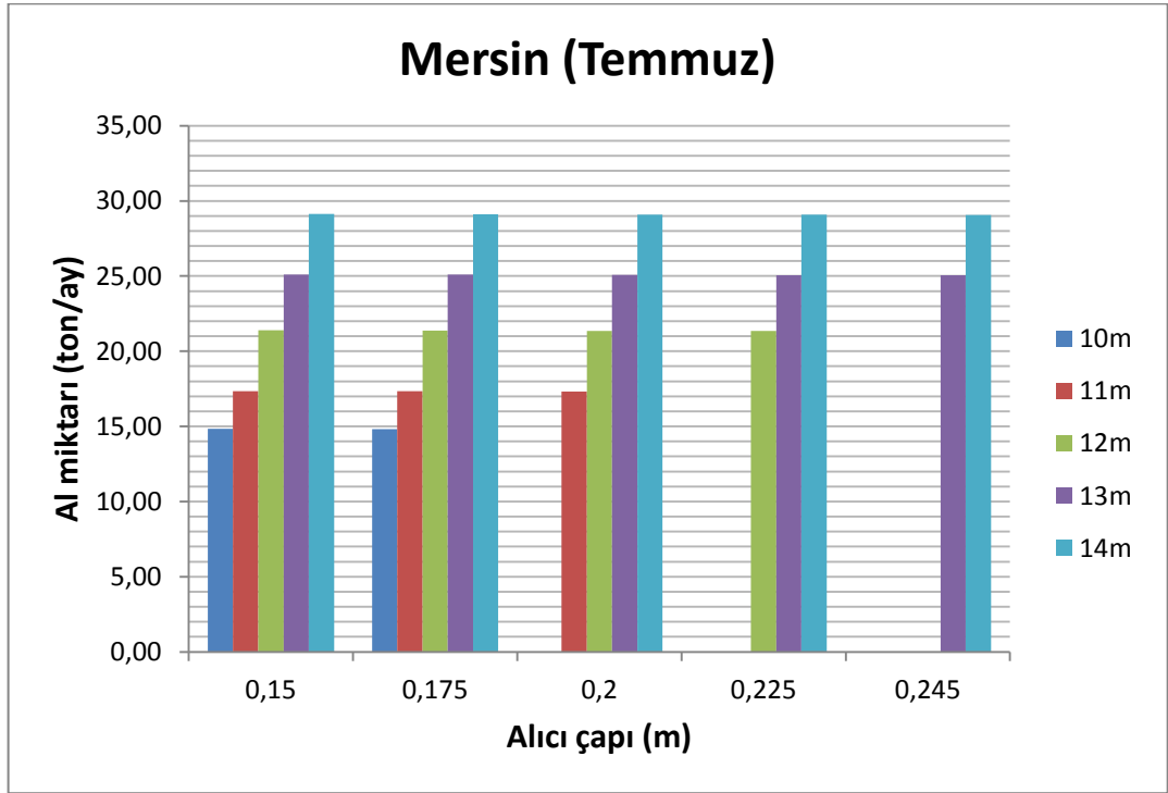
Şekil 4. 13 Temmuz ayı Mersin için çanak-pota çapı ve Al miktarı karşılaştırması
