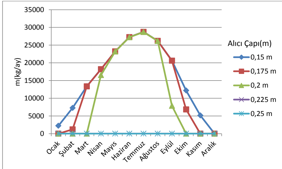
Şekil 4. 30 Mersin’de Çanak çapı 11 m için aylara göre eriyen Al miktarı
