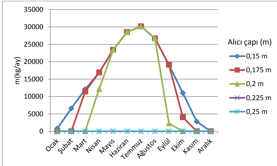
Şekil 4. 25 İzmir’de Çanak çapı 11 m için aylara göre eriyen Al miktarı
