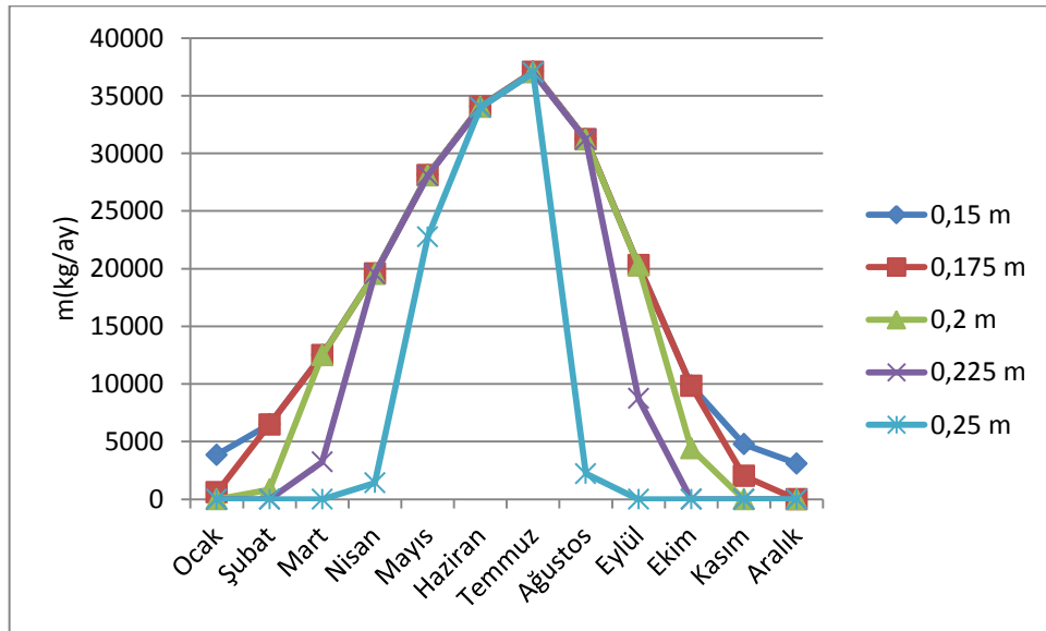
Şekil 4. 22 İstanbul'da Çanak çapı 13 m için aylara göre eriyen Al miktarı
