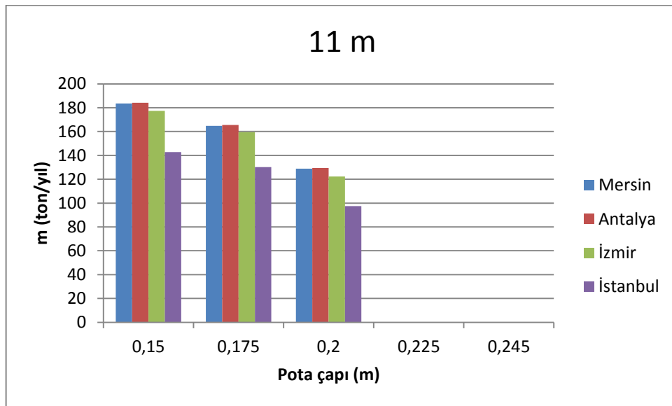
Şekil 4. 8 11 m'lik çanak çapı için 4 şehrin Al miktarı karşılaştırması
