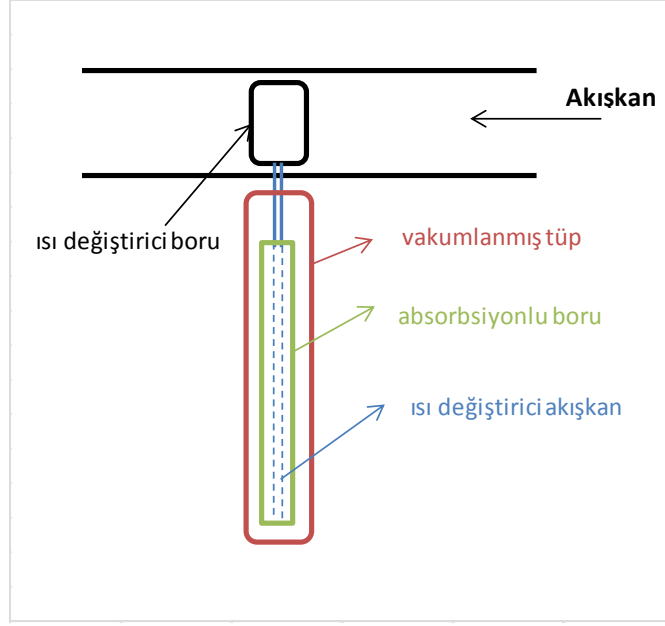
Şekil 2. 3 Vakum tüplü kolektör
