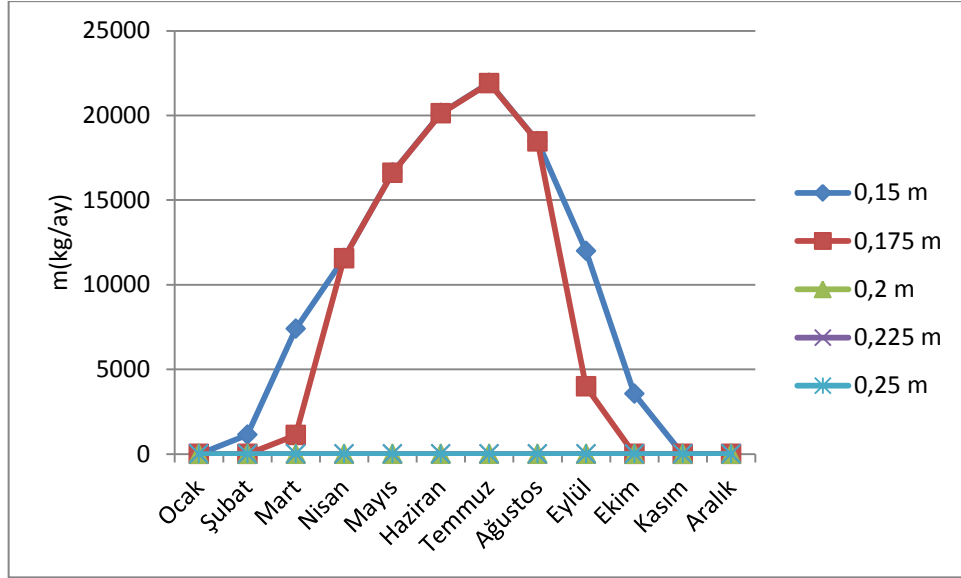
Şekil 4.19 İstanbul'da Çanak çapı 10 m için aylara göre eriyen Al miktarı
