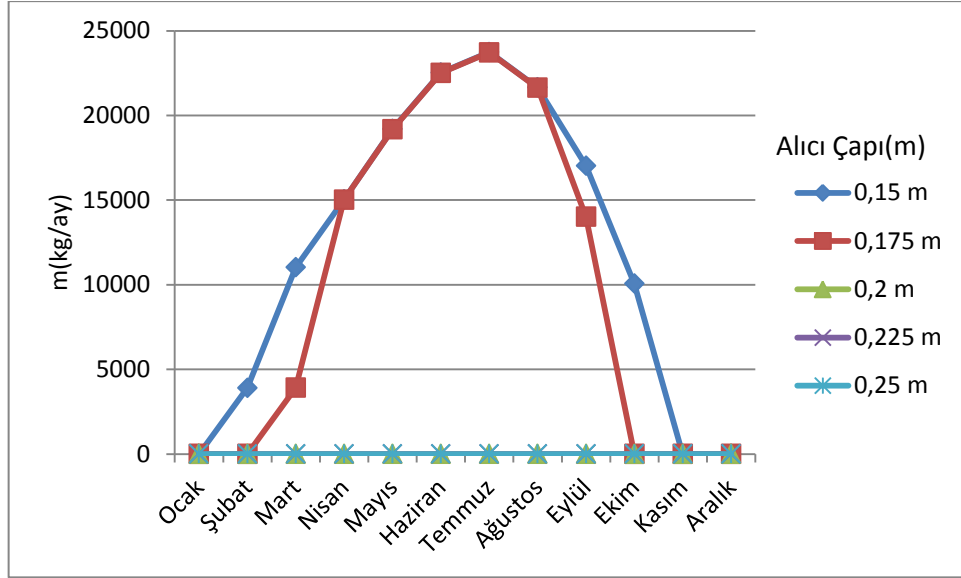
Şekil 4. 29 Mersin’de Çanak çapı 10 m için aylara göre eriyen Al miktarı
