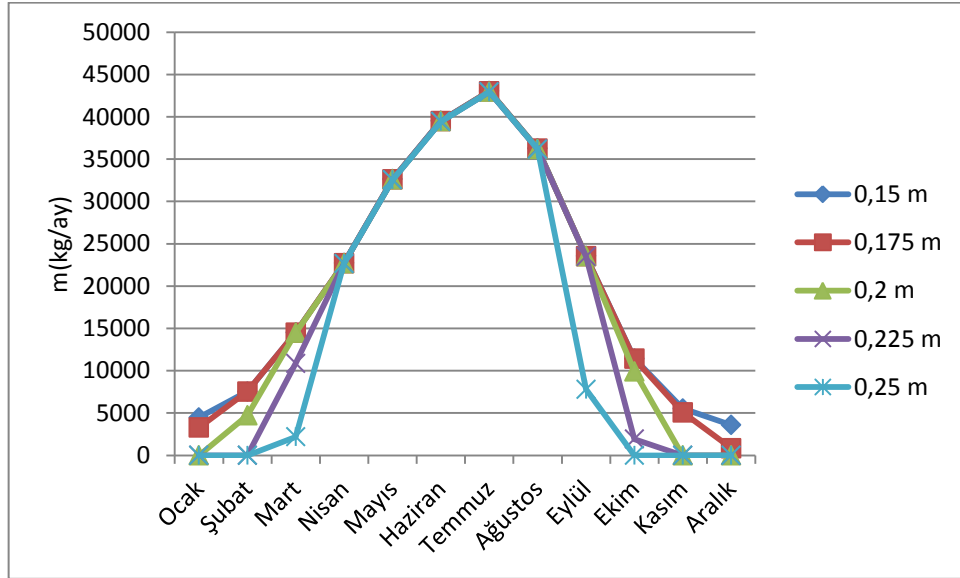
Şekil 4. 23 İstanbul’da Çanak çapı 14 m için aylara göre eriyen Al miktarı
