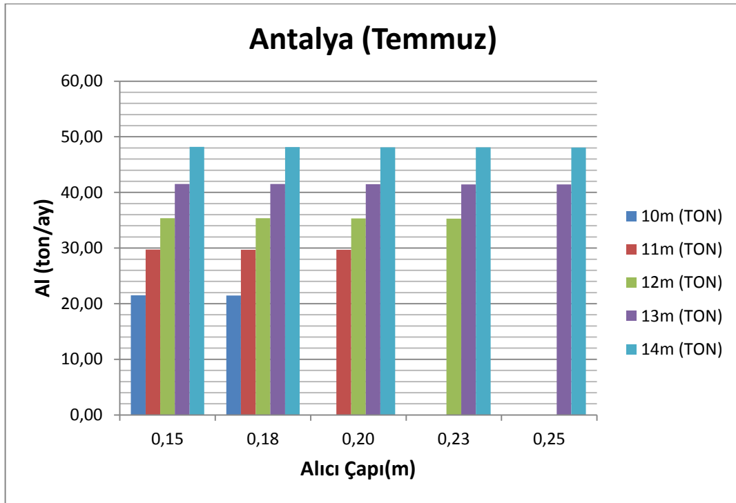
Şekil 4. 12 Antalya'da Temmuz ayı için ergiyen Al karşılaştırması
