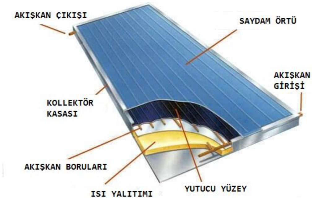
Şekil 2. 1 Düz toplayıcı
