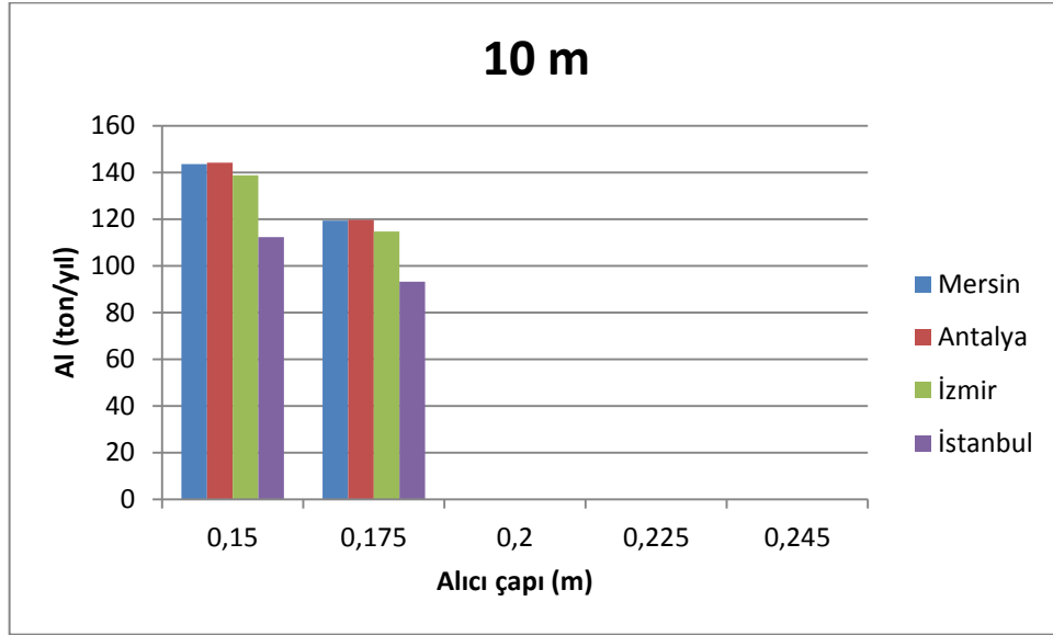
Şekil 4. 7 10 m'lik çanak çapı için 4 şehrin Al miktarı karşılaştırması
