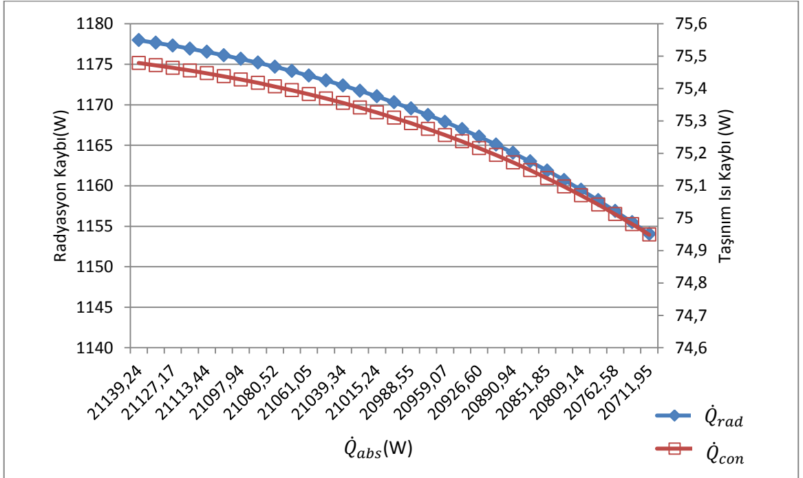
Şekil 4. 35 10 m'lik çanakta 0,15 m'lik alıcıdaki oluşan toplam kayıp
