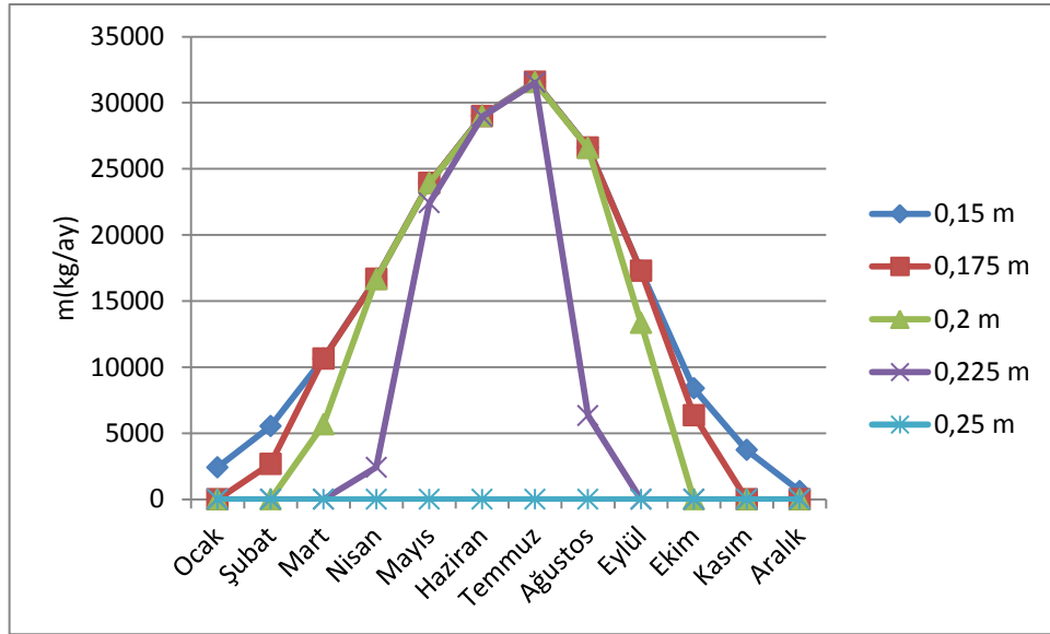
Şekil 4. 21 İstanbul'da Çanak çapı 12 m için aylara göre eriyen Al miktarı
