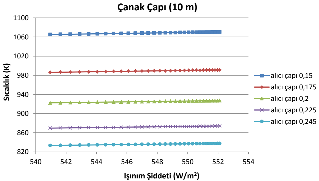
Şekil 4. 5 Antalya'daki çanak çapı 10 m için İşınım Şiddeti-Sıcak
