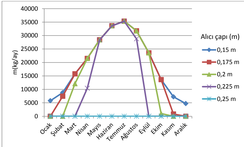
Şekil 4.16 Antalya'da Çanak çapı 12 m için aylara göre eriyen Al miktarı
