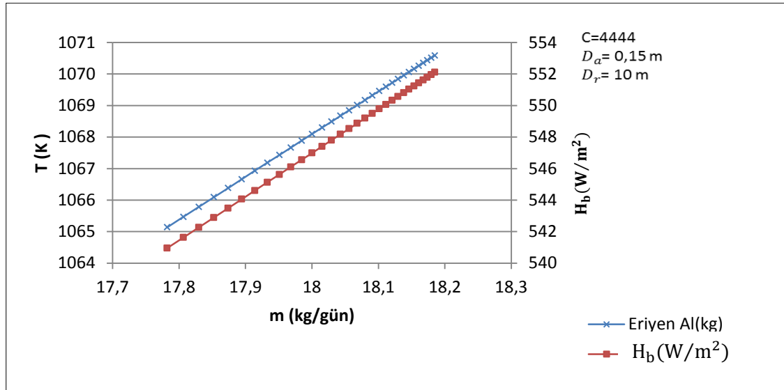
Şekil 4. 6 Antalya için Sıcaklık-ışınım Şiddeti-Al miktarı ilişkisini gösteren grafik
