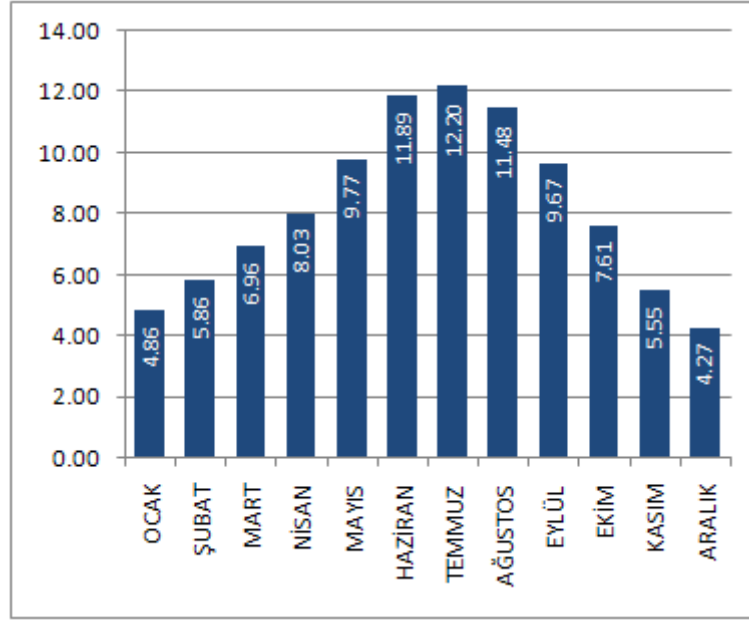
Şekil 4. 3 İzmir aylık ortalama güneşlenme süresi [24]
