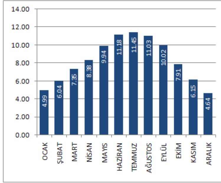
Şekil 4. 1 Mersin aylık ortalama güneşlenme süresi [24]
