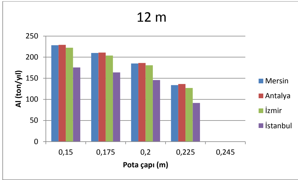
Şekil 4. 9 12 m'lik çanak çapı için 4 şehrin Al miktarı karşılaştırması
