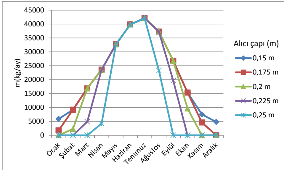
Şekil 4. 27 İzmir’de Çanak çapı 13 m için aylara göre eriyen Al miktarı
