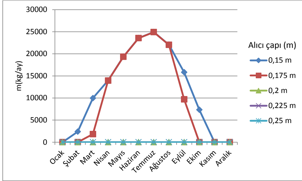
Şekil 4. 24 İzmir’de Çanak çapı 10 m için aylara göre eriyen Al miktarı
