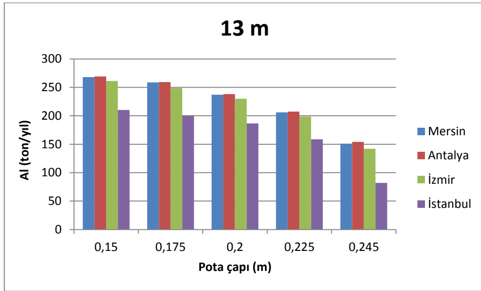
Şekil 4. 10 13 m'lik çanak çapı için 4 şehrin Al miktarı karşılaştırması
