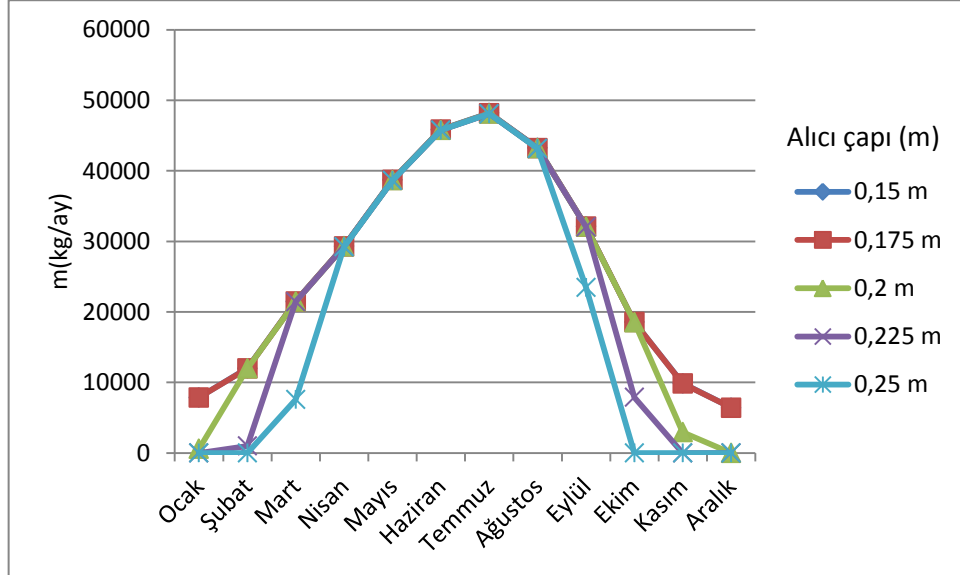
Şekil 4.18 Antalya’da Çanak çapı 14 m için aylara göre eriyen Al miktarı
