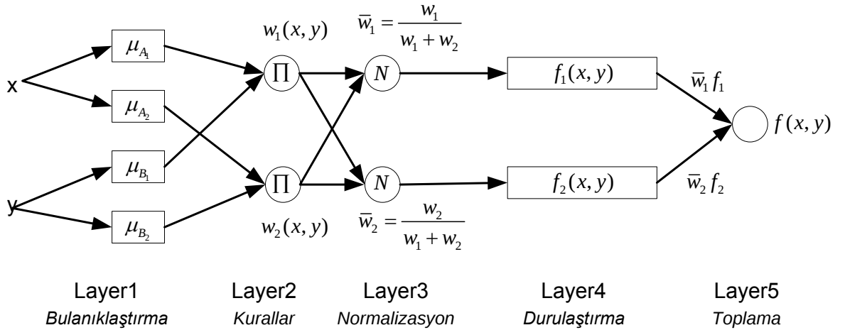
Şekil 4.4 Genel ANFIS yapısı.
