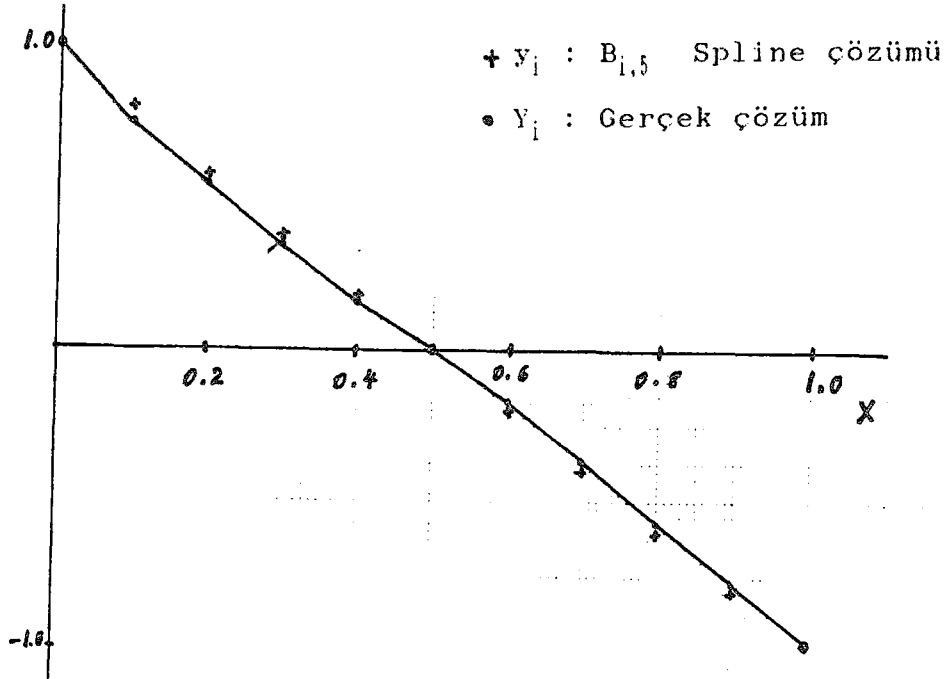
Şekil 4.5 B_{i,5} spline ve gerçek çözüm grafiği
