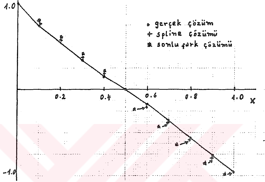
Şekil 4.7 Spline çözümü ve sonlu fark yöntemiyle çözümün grafik olarak gösterilmesi
