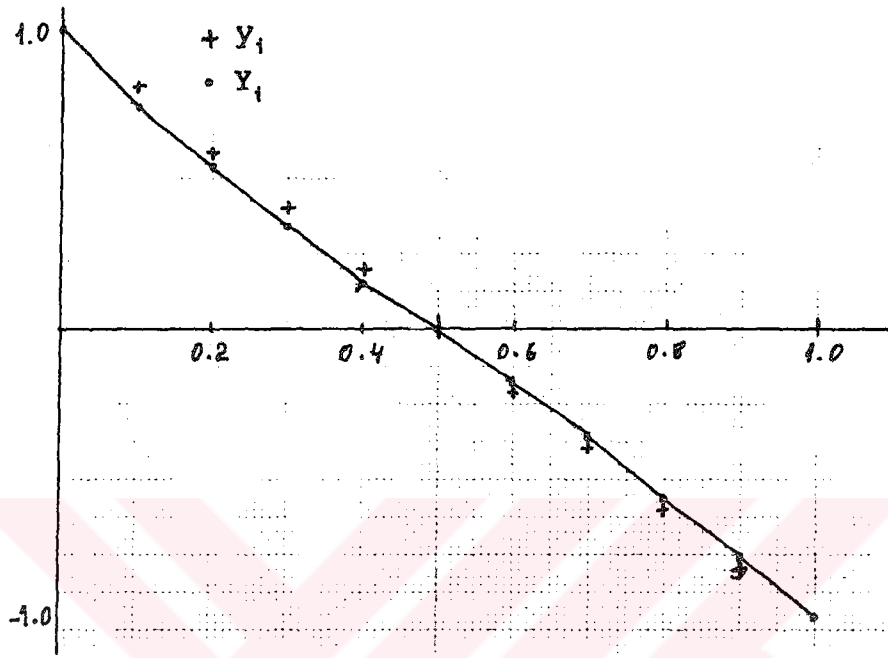
Şekil 4.10 B_{1,6} Spline ve gerçek çözüm grafiği
