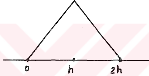
Şekil 3.2.2 B_{1,2} Spline
