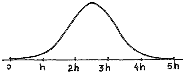
Şekil 3.2.5 B_{1,5} Spline
