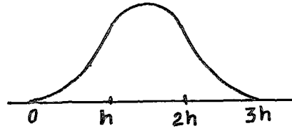
Şekil 3.2.3 B_{i,3} Spline
