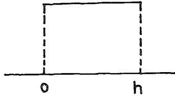
Şekil 3.2.1 B_{i,1} Spline
