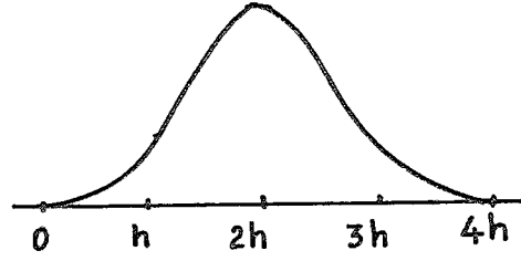
Şekil 3.2.4 B_{i,4} Spline
