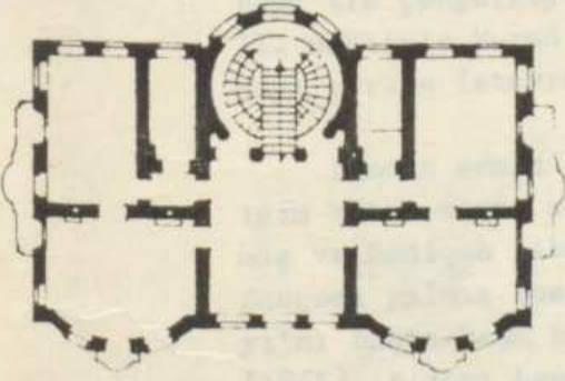
KÜÇÜKSU KASRI PLANI
