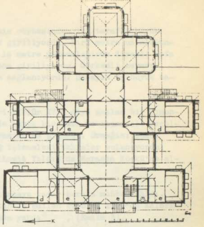
Bebek kasrının 18.yüzyıl Gudenus krokisine göre restitüsyonu
