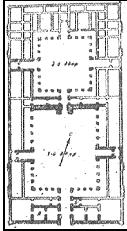
Akçakale Kervansarayı planı (Karahanlılar) (Aslanapa, 1984)
