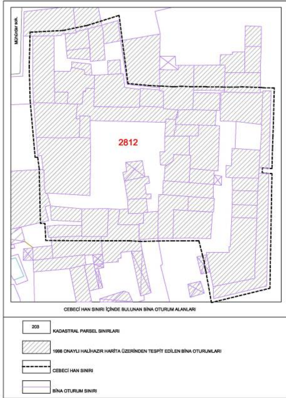
Plan 7.1 Cebeci Han sınırı içinde bulunan bina oturma alanları; günümüzde Cebeci Handa mevcut bulunan yapıların işgal ettikleri alanlar
