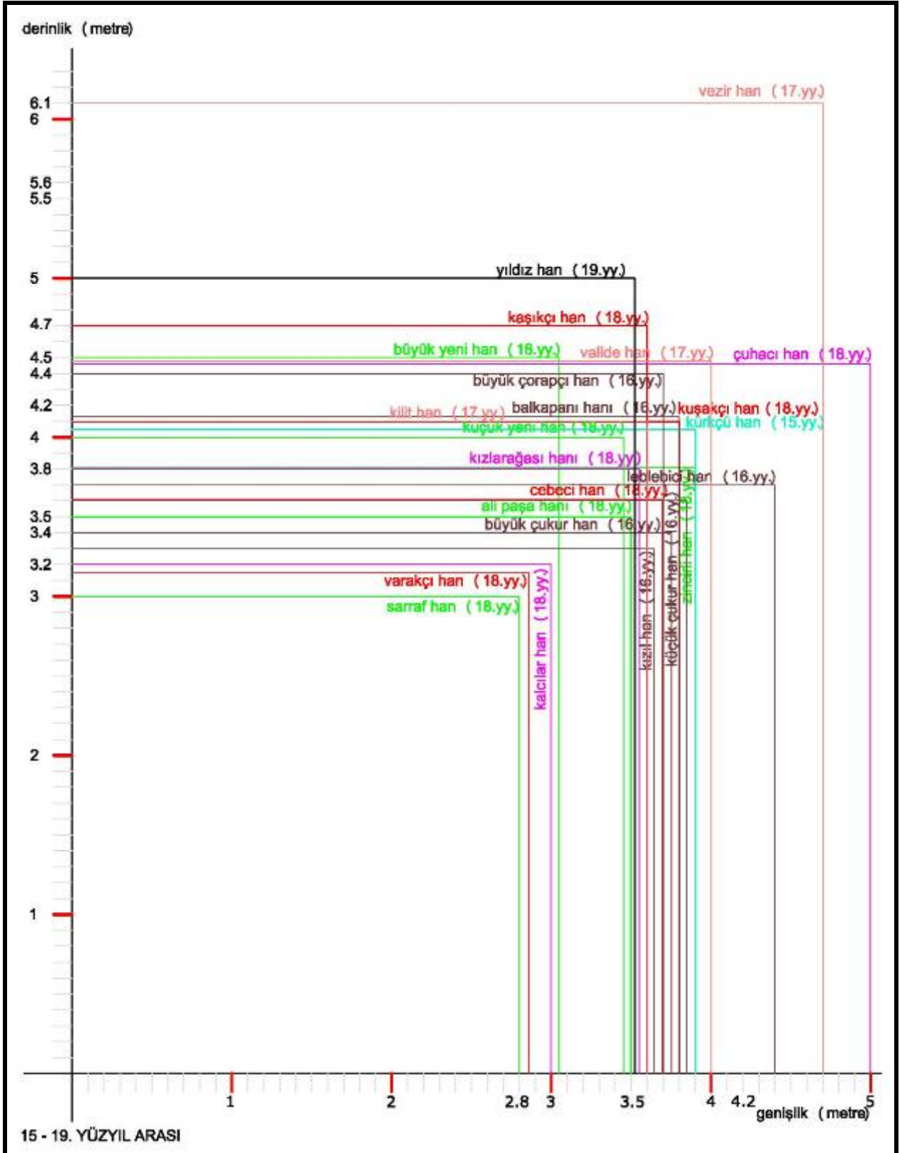
Grafik 5.6 23 adet örnek odada uygulanan genişlik ve derinlikler (oda planını vermektedir)
