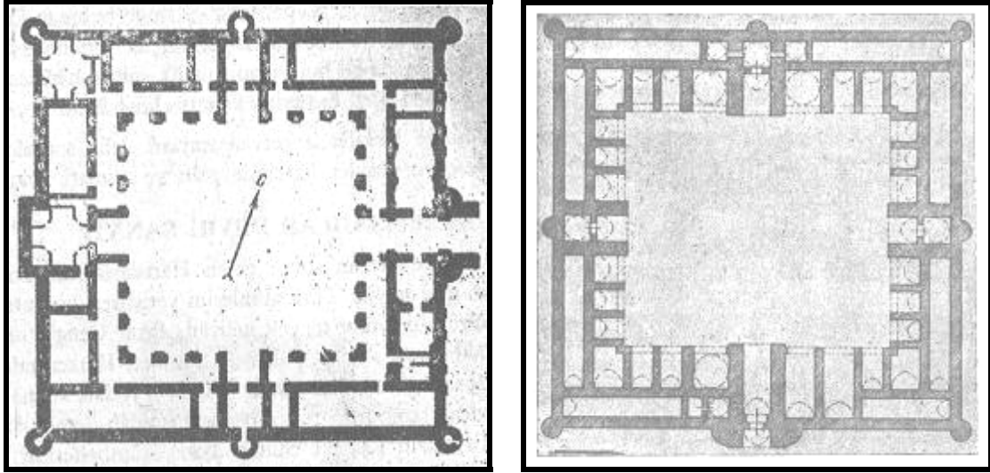
Plan 2.1 Day Hatun Kervansarayı (Aslanapa, 1984) Ribatı Mahi Planı (Aslanapa, 1984)
