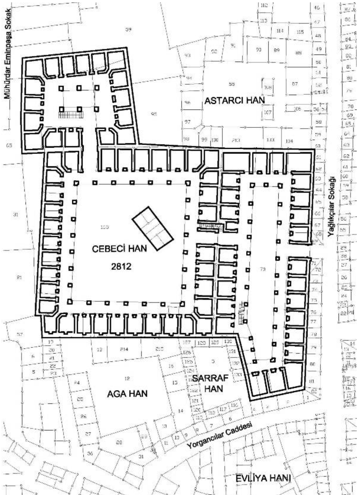
Plan 7.7 Cebeci Han zemin plan restitüsyonu
