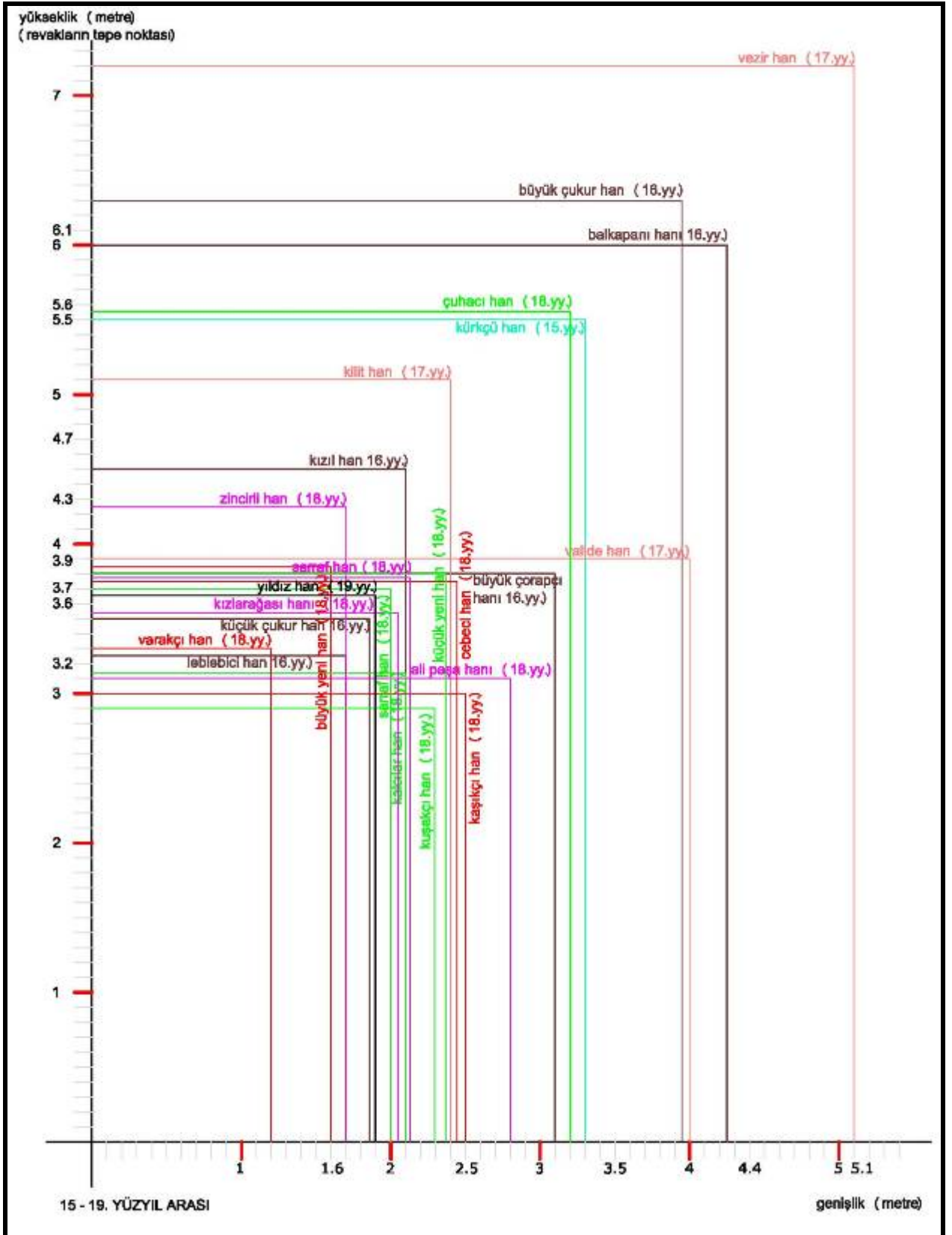
Grafik 5.3 Revak kesitleri (23 adet örnek üzerinden revakta uygulanan genişlik ve tepe noktasını gösteren yüksekliklerin bir arada gösterilmesi)
