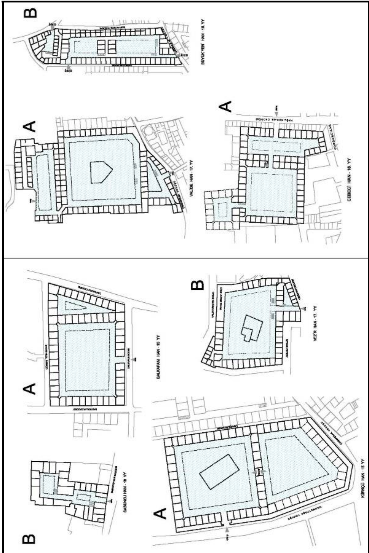
Plan 5.2 İki ve üç avlulu hanlar (planlar aynı ölçektir ve ismin yanında yazılı olan harf, planlama ilkesini temsil etmektedir)
