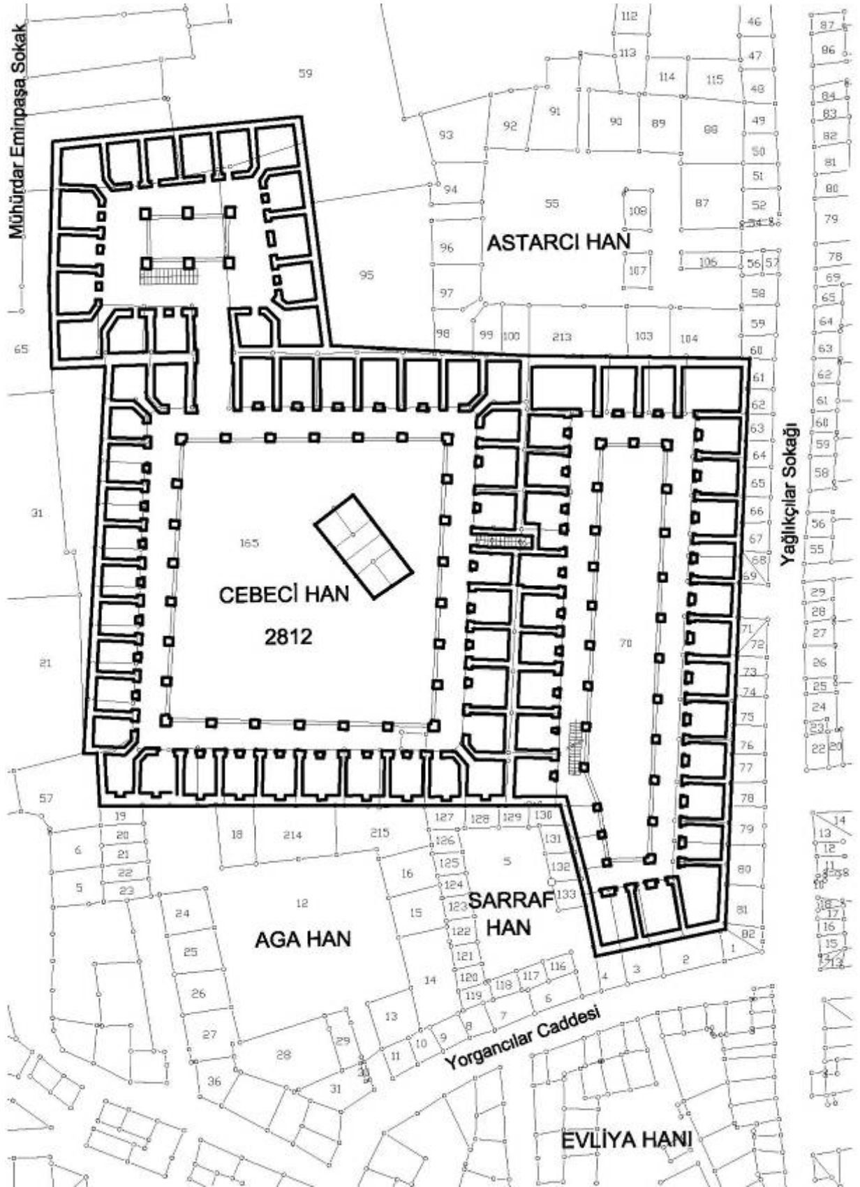
Plan 7.7.6 Cebeci Han 1. kat plan restitüsyonu
