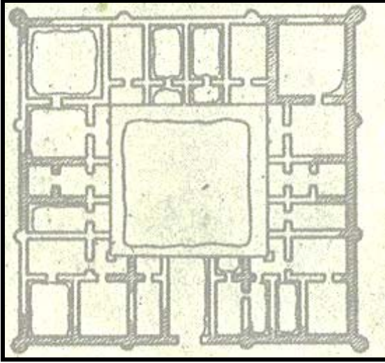
Plan 2.2 Dehistan Kervansarayı
