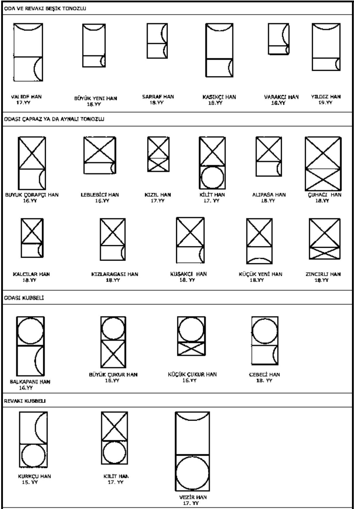
Şekil 5.1 Üst örtü biçimlenişleri
