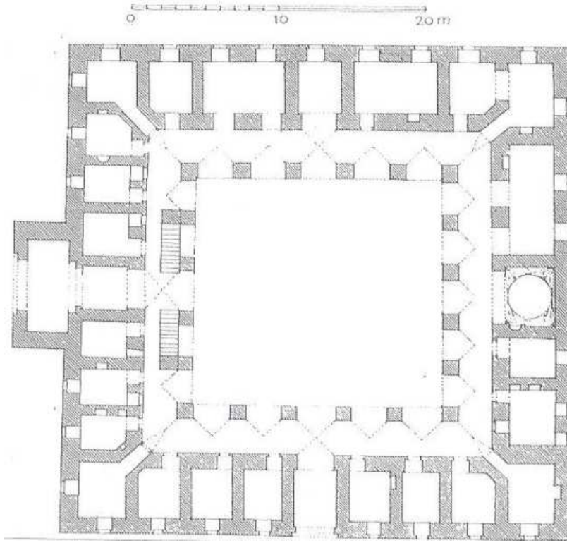
Şekil 4.13 Geyve Han zemin kat planı ve kesiti(Gabriel, 1958).
