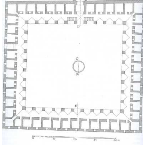
Şekil 4.33 Fidan Han zemin kat planı ve kesiti (Gabriel, 1958)
