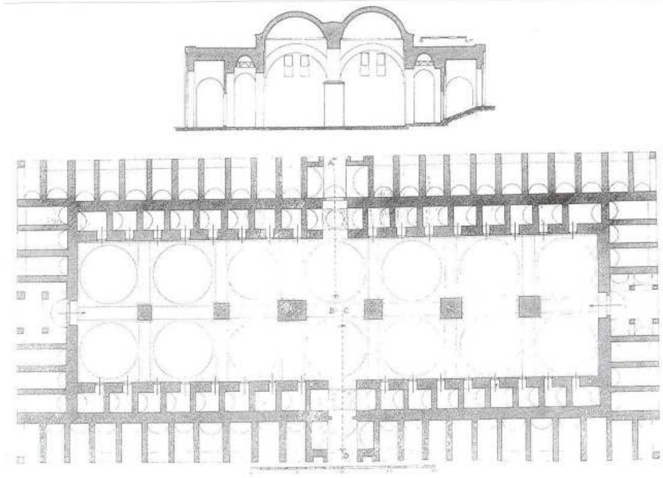
Şekil 4.9 Bedesten plan ve kesiti(Gabriel, 1958).
