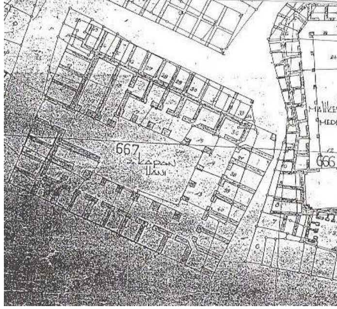
Şekil 4.7 Kapan Han zemin kat planı (BKTVKK arşivi).
