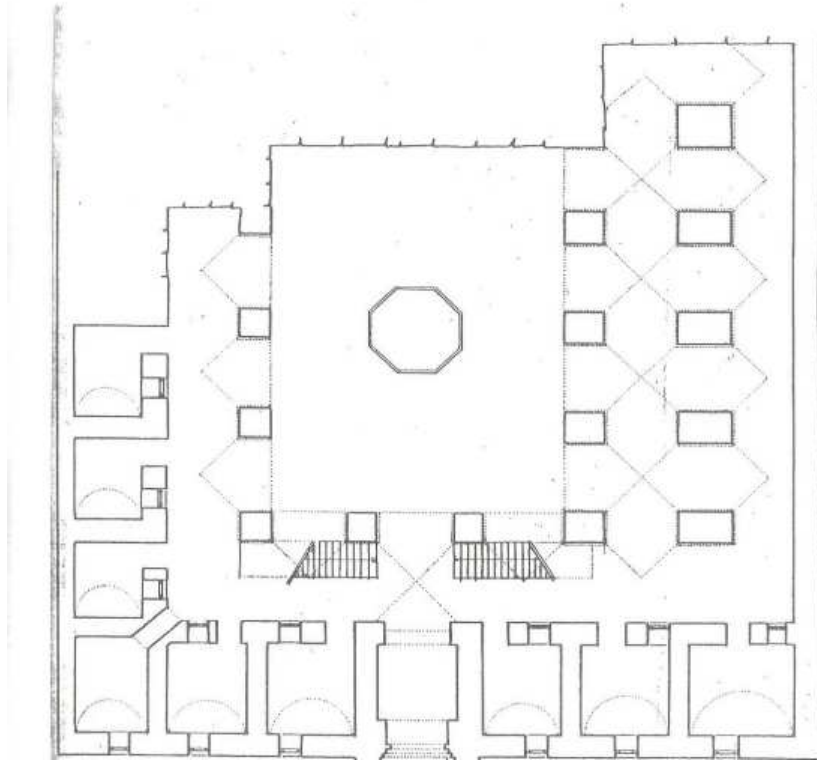
Şekil 4.41 Bali Bey Hanı zemin kat planı (Çobanoğlu, 1986)
