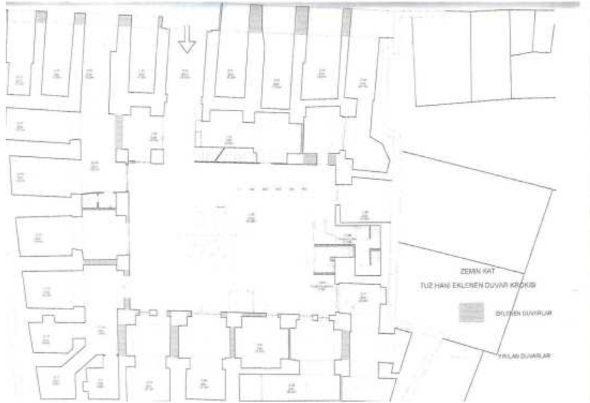
Şekil 4.31 Tuz Han zemin kat planı (Üngörgil, 2003).
