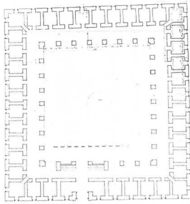
Şekil 4.11 İpek Han zemin kat planı (Ayverdi,1972).
