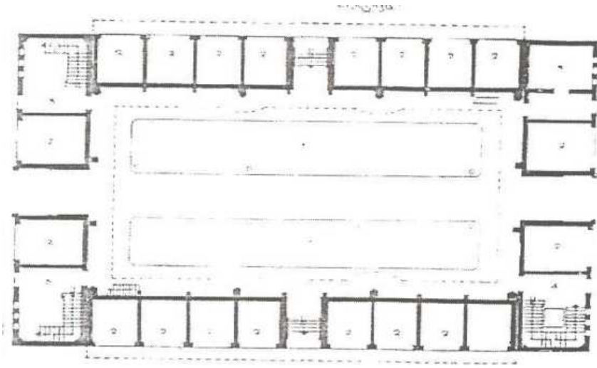
Şekil 4.143 Hal binası zemin kat planı (Arkitekt, 1950)
