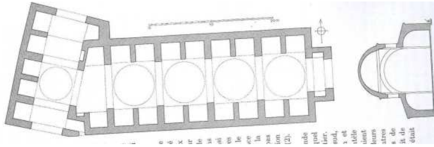
Şekil 4.68 Sipahi Çarşısı plan ve kesiti(Gabriel,1958).
