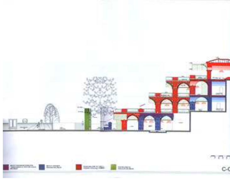
Şekil 4.208 Bali Bey Hamı restorasyon projesi kesiti( www.bursa-bld.gov.tr ).
