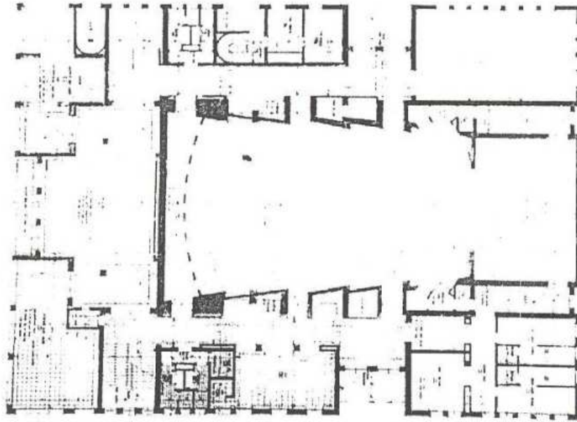
Şekil 4.157 Tayyare Kültür Merkezi zemin kat planı(Mimarlık Dergisi, Bursa Şubesi ,1999).
