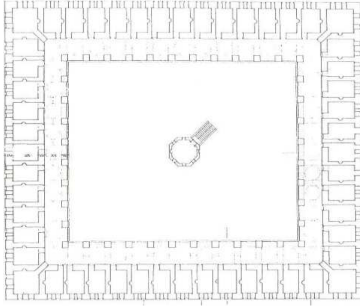
Şekil 4.37 Koza Han birinci kat planı (Yüksel, 1980, s.75)
