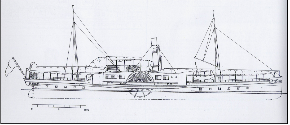
Şekil 2.3 Büyükada Vapuru
