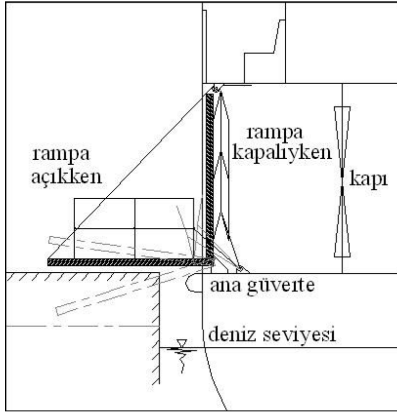
Şekil 3.7 Yolcu Rampası
