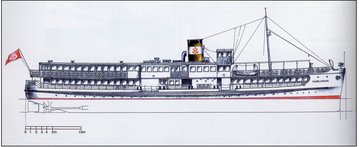
Şekil 2.29 Rumelihisari Vapuru
