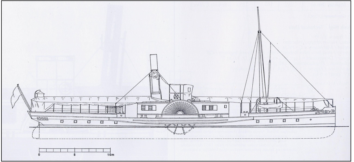
Şekil 2.2 Beykoz Vapuru
