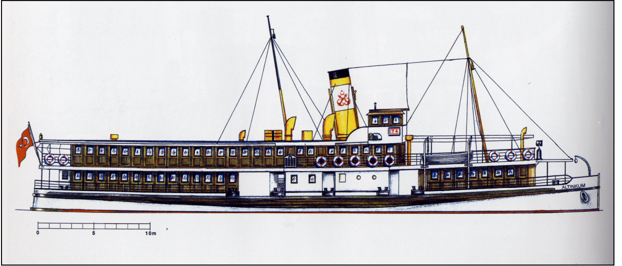
Şekil 2.27 Altınkum Vapuru
