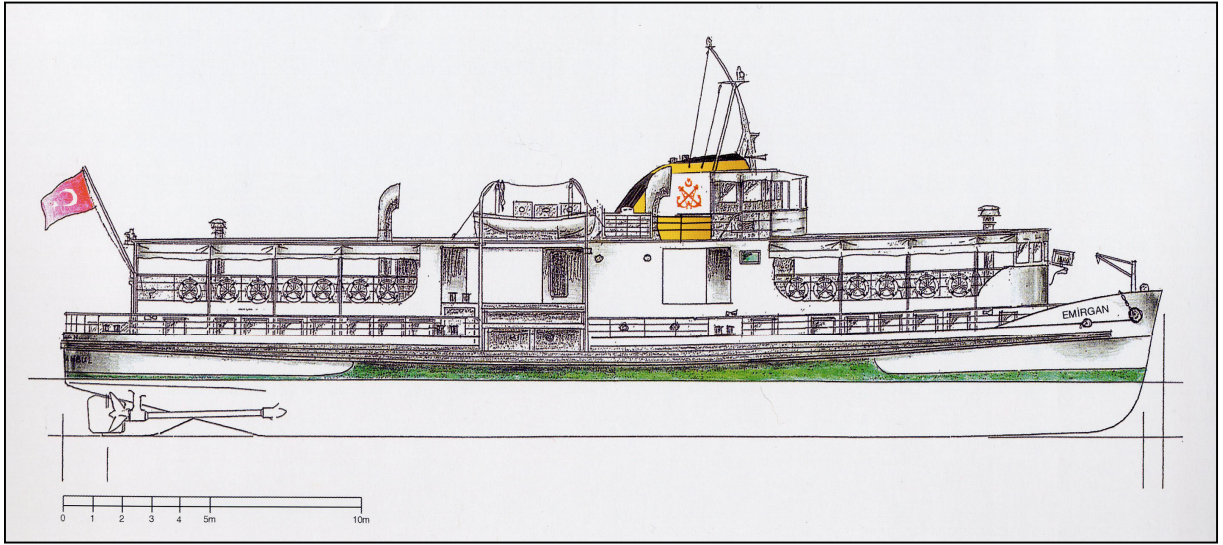
Şekil 2.32 Emirgan Vapuru
