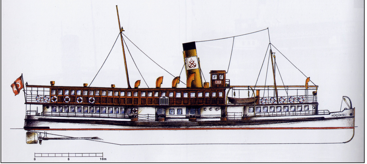
Şekil 2.20 Küçükusu Vapuru
