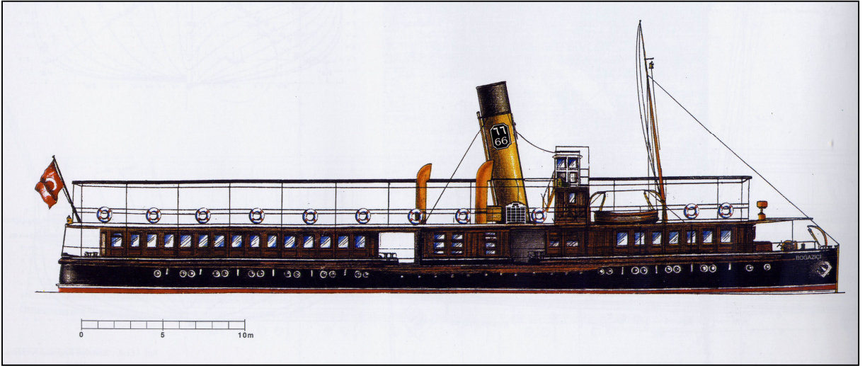
Şekil 2.22 Boğaziçi Vapuru
