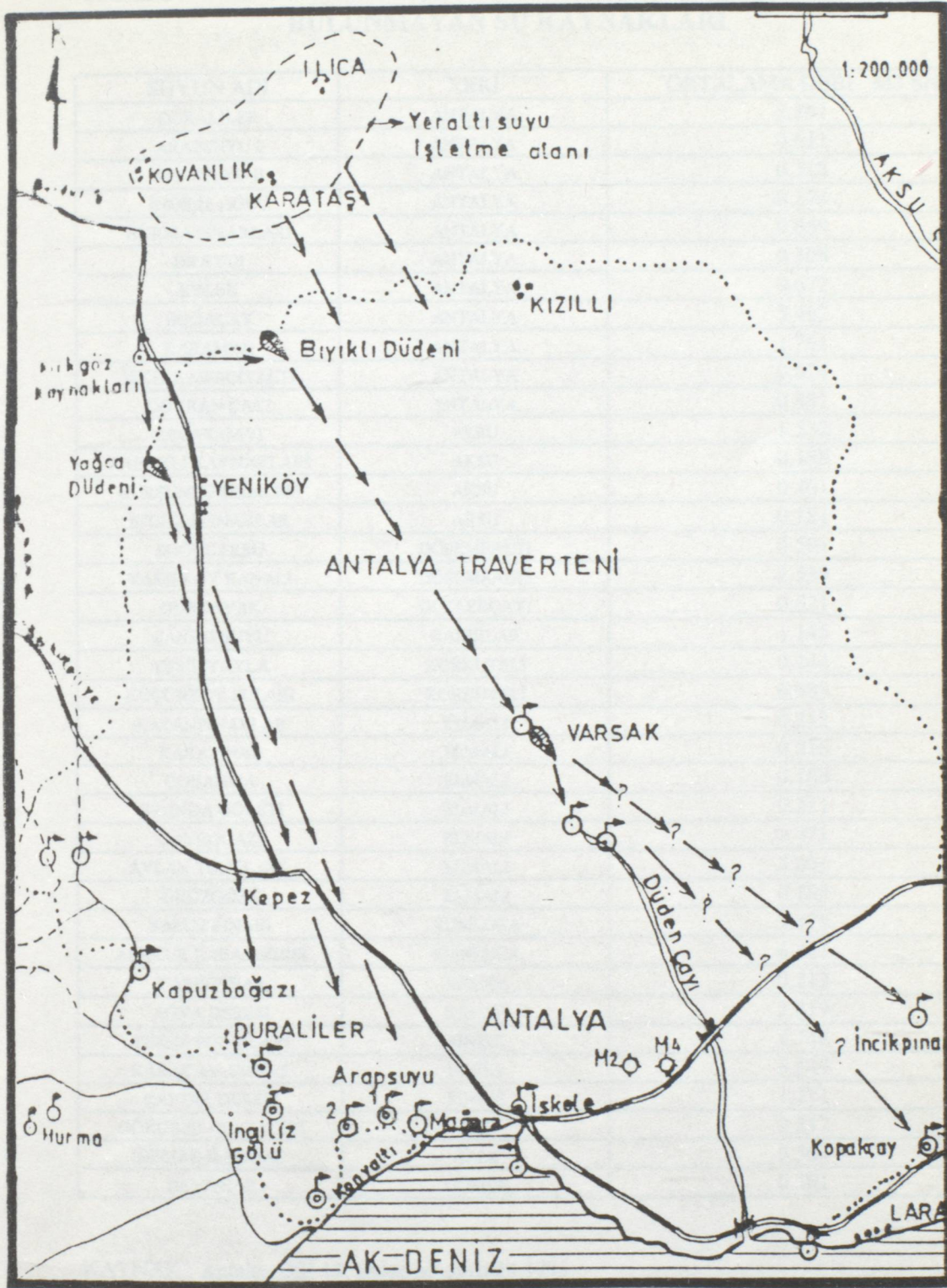
HARİTA - 6 ANTALYA'DAKİ MEVCUT SU KAYNAKLARI
