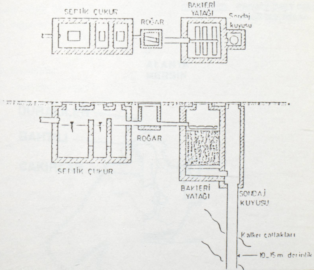
ŞEKİL - 3 ANTALYA ŞEHRİNİN ATIK SULARINI UZAKLAŞTIRMA TESİSİ
