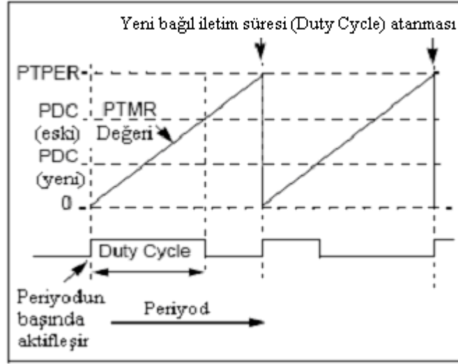
Şekil 4.6 Kenar ile çakışık PWM.
