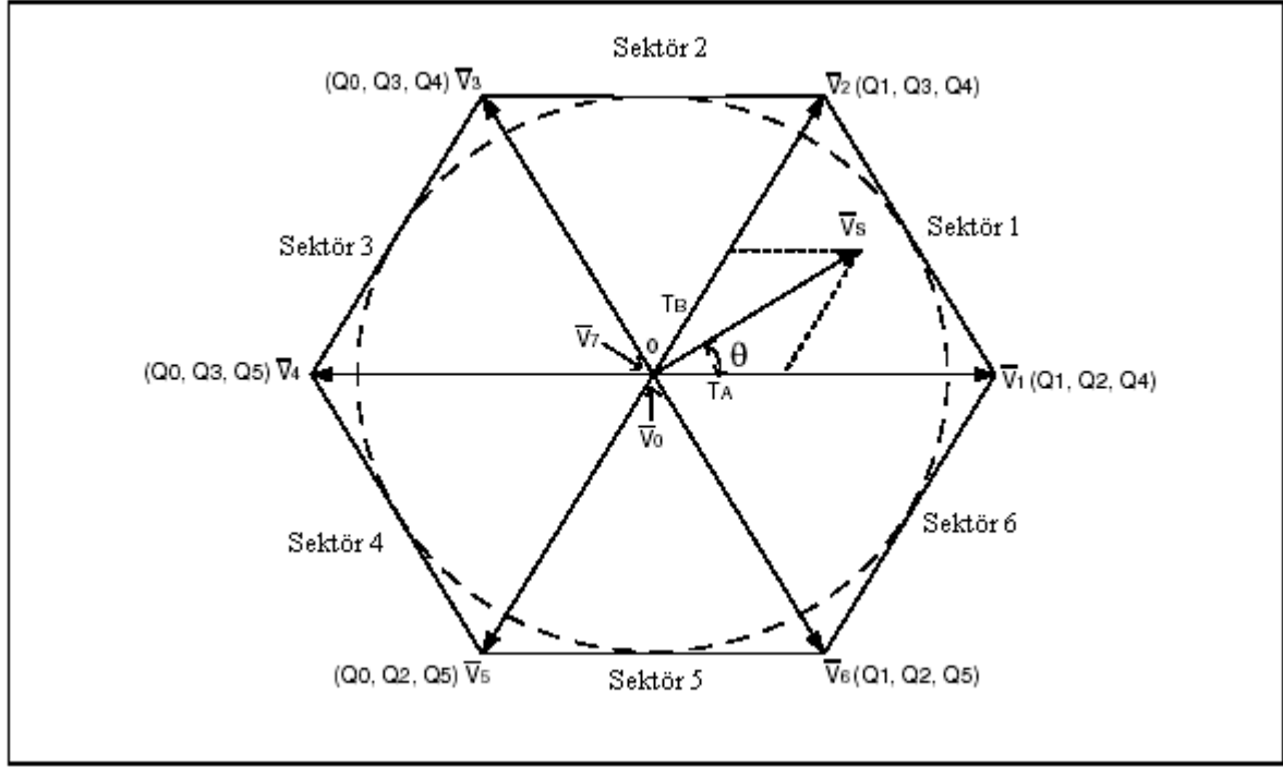
Şekil 4.14 Uzay vektör altıgeni.
