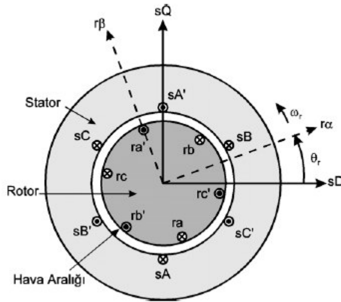
Şekil 2.1 Üç fazlı simetrik asenkron motorun temel yapısının temel kesiti.
