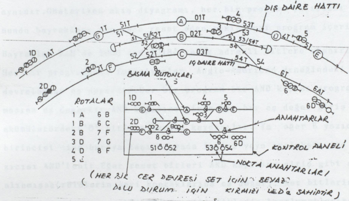
şekil 4: Ana kilitleme modeli
