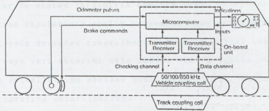
Şekil 21- Çalışma Prensibi
