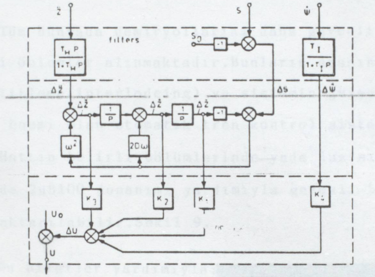
Şekil 8- Bir manyetik tekerleğin kontrolör yapısı
