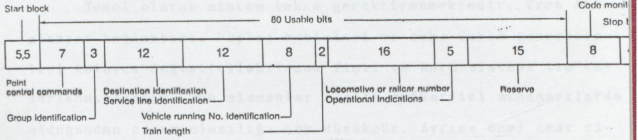
Şekil 23- Trenden raya gönderilen telgrafın genel yapısı
