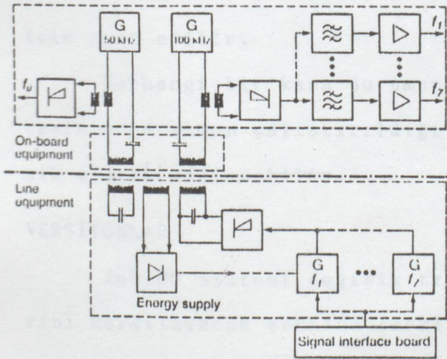
Şekil 19-Frekans Bölümlü Çalışma
