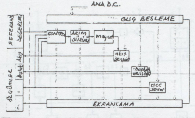
Şekil 7-Manyetik tekerleğin elektriksel yapısı
