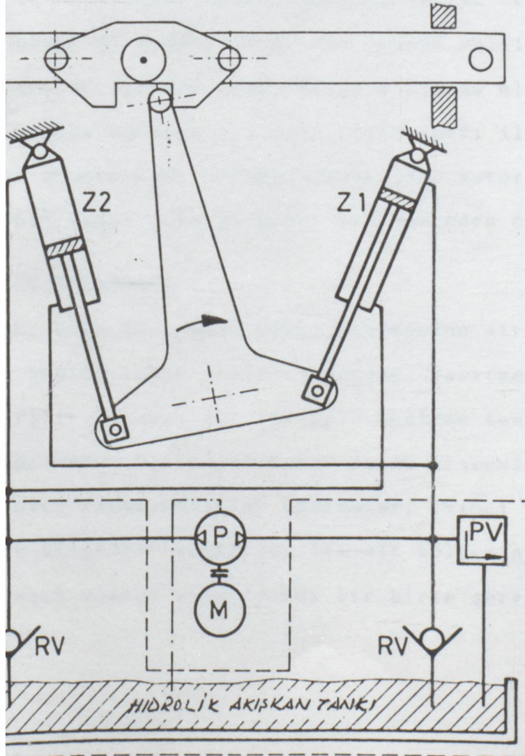
Hidrolik anahtar
