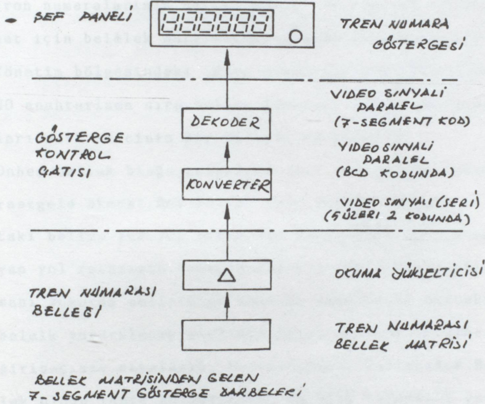
Şekil 25-Bellekmatrisinden 7- segment gösterge.
