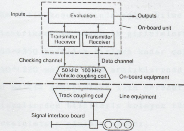
Şekil 16-Sistemin çalışma prensibi.
