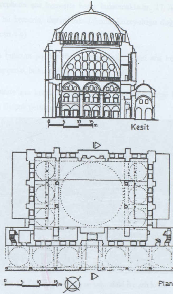
Şekil 4.1 Caminin plan ve kesiti
