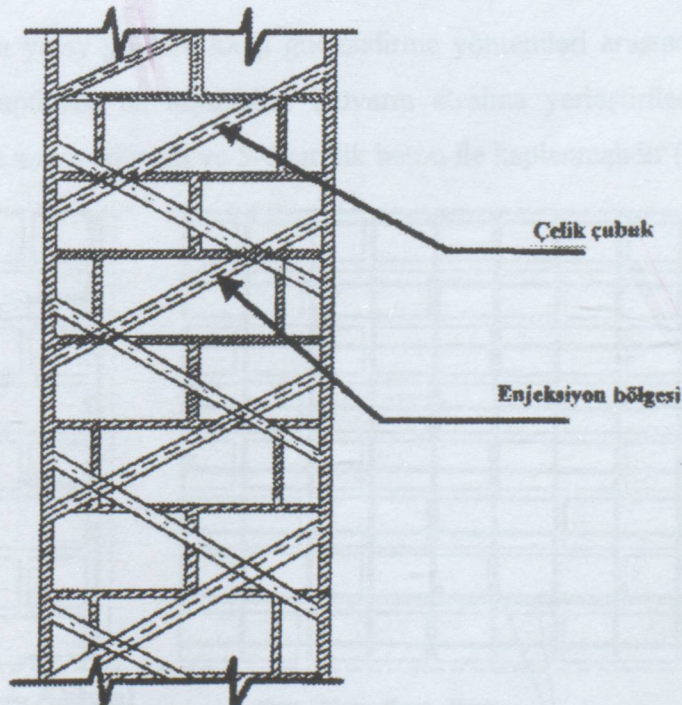
Şekil 2.6 Çimento ağı ile takviye (Garevski, 1995)
