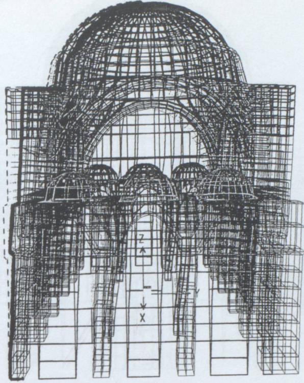
Şekil 4.5 Yapının 1. mod şekli (Doğu cephesinden görünüş, T=0.4422 s)
