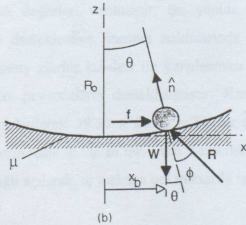
Şekil 3.7 Sürtünmeli sarkaç yalıtım sistemi elemanı
