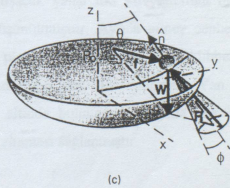
Şekil 3.7 Sürtünmeli sarkaç yalıtım sistemi elemanı
