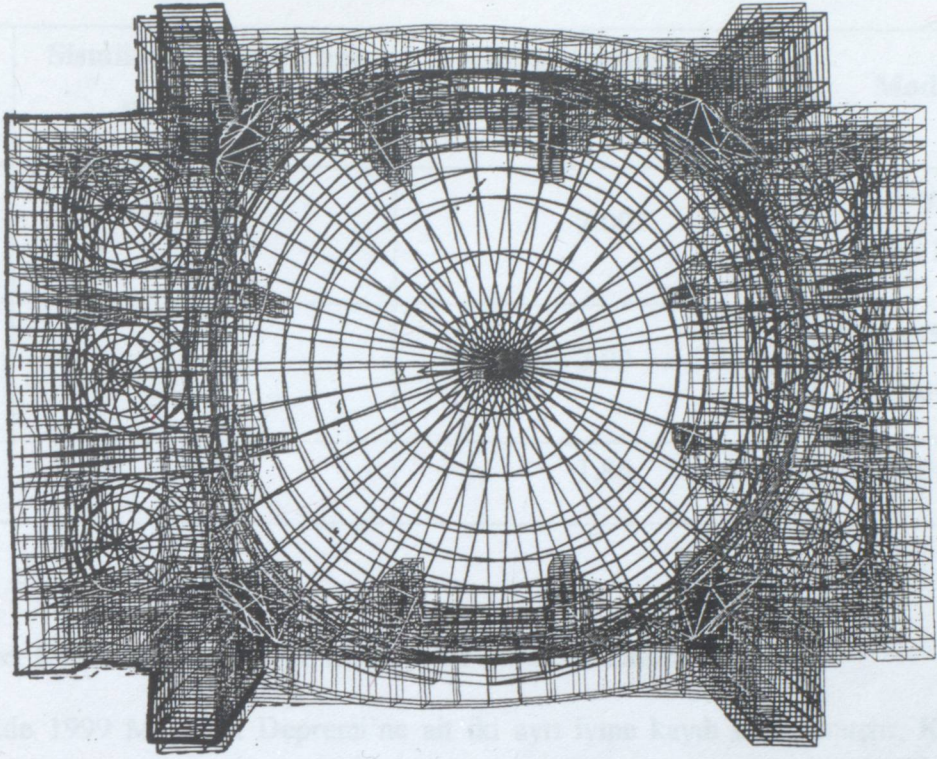
Şekil 4.9 Yapının 3. mod şekli (Üstten görünüş, T=0.1702 s)
