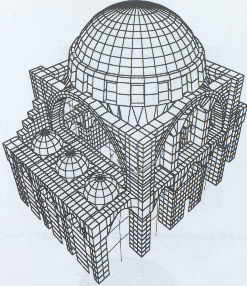
Şekil 4.4 Modelin genel görünüşü
