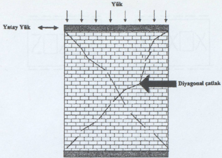
Şekil 2.1 Yığma duvar elemanında kesme çatlakları
