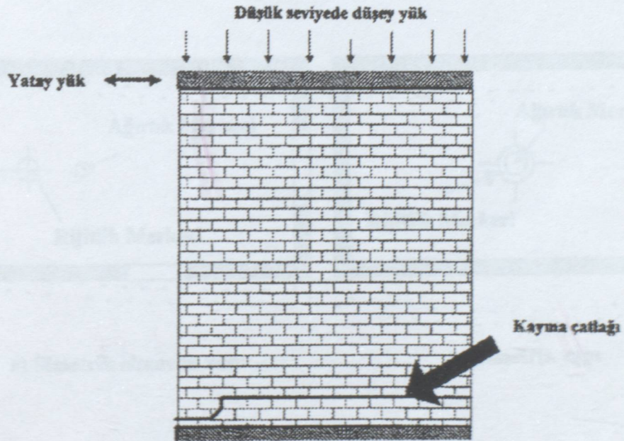
Şekil 2.2 Düşük düşey yük etkisindeki yığma duvar elemanında kayma çatlakları
