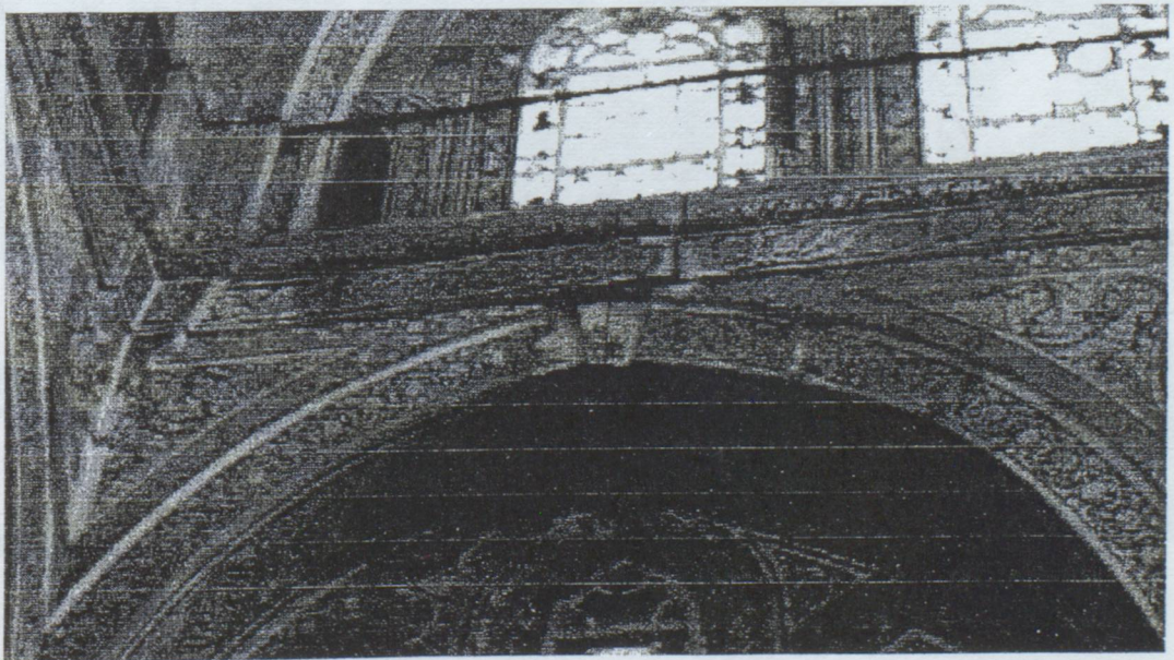
Foto 4.3 Güney cephesinde galeri seviyesindeki hasarlı kemer.
