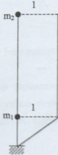
Şekil 3.2 Sismik yalıtımlı yapıya ait 1. mod şekli
