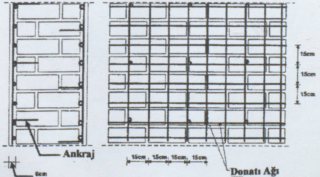
Şekil 2.8 Mantolama (Garevski, 1995)
