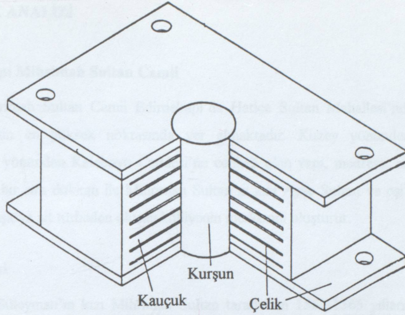
Şekil 3.6 Merkezinde kurşun bulunan elastomerik yalıtım sistemi elemanı
