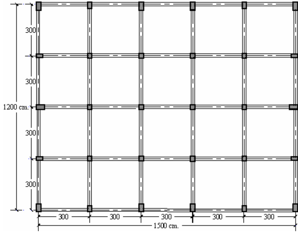
Şekil 5.1 Taşıyıcı sistem kat kalıp planı
