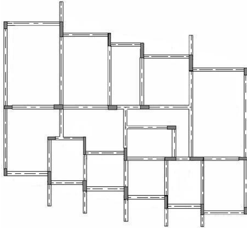
Şekil 6.57 Şahin Apt. bodrum, zemin ve normal kat kalıp planı
