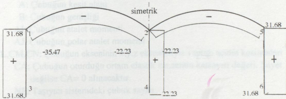
Şekil 4.3 Normal Kuvvet Diyagramı (t)
