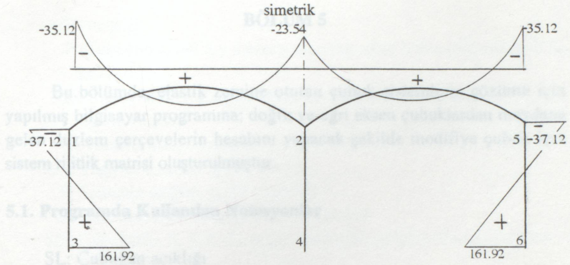
Şekil 4.2 Eğilme Momenti Diyagramı (tm)
